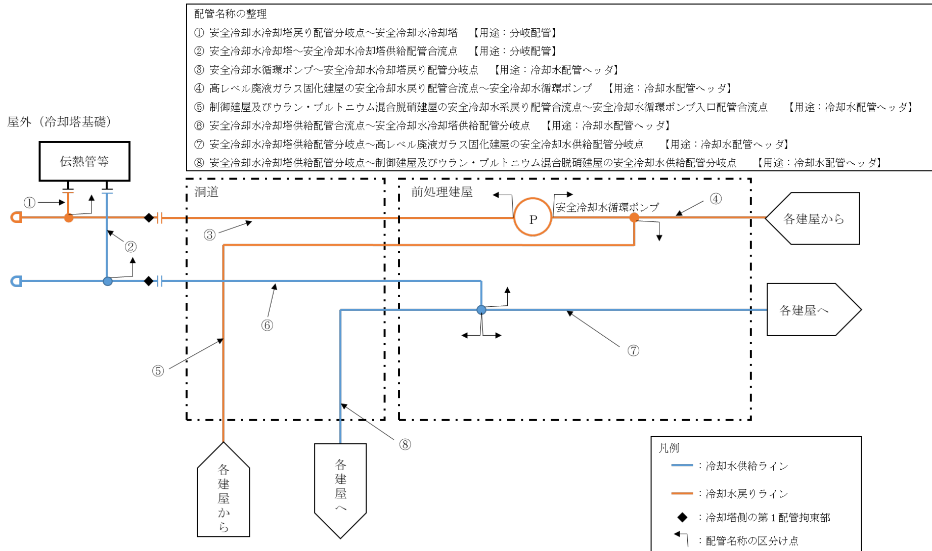
図－1 安全冷却水系の系統概要及び配管名称の区分け図
