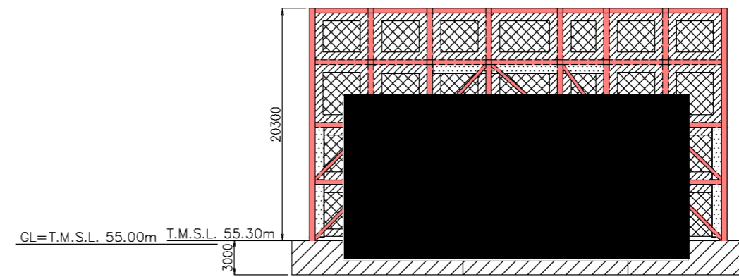
西面 (d 視)
