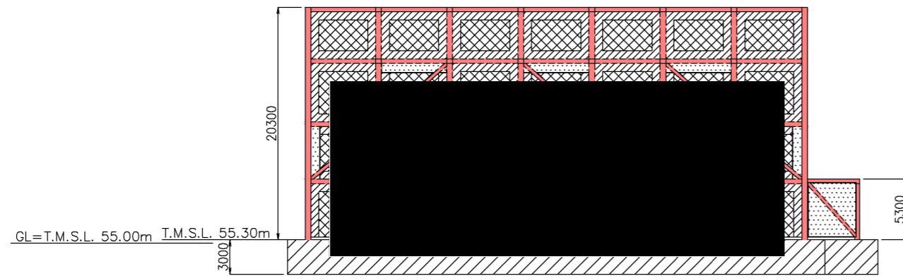
北面 (a 視)
