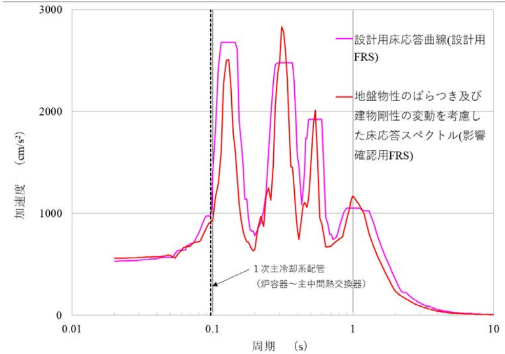
【Ss-6 (UD 方向) / 減衰定数 : 0.025 / 原子炉建物 質点④】
