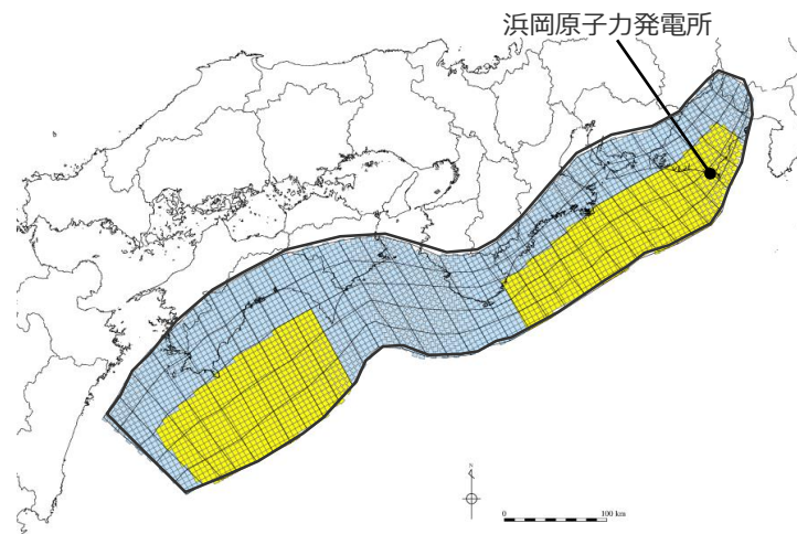
南海トラフ広域の痕跡再現モデル
