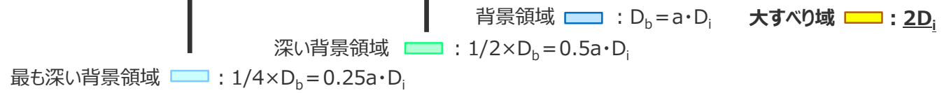
遷移領域のすべり量 D (m)の設定方法
