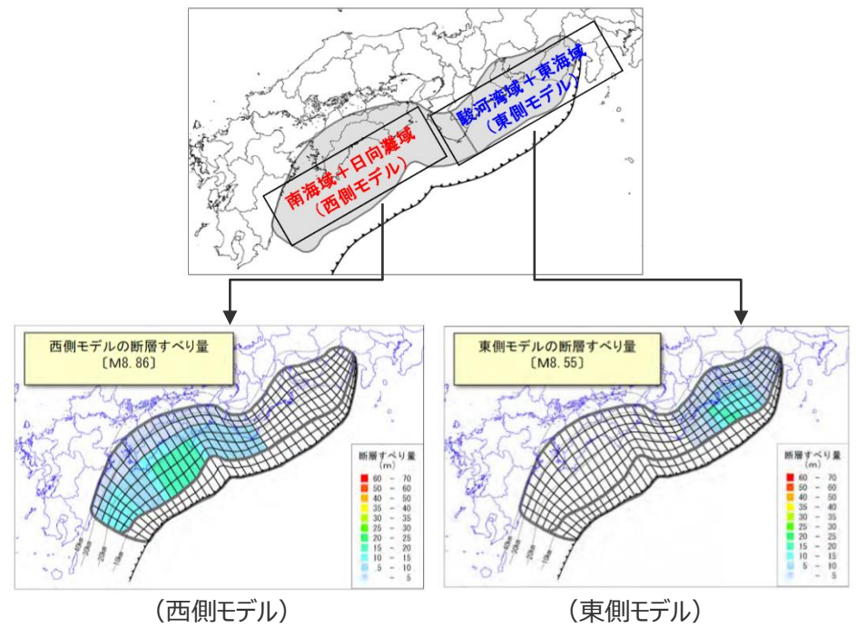
時間差発生モデル (内閣府(2012))
