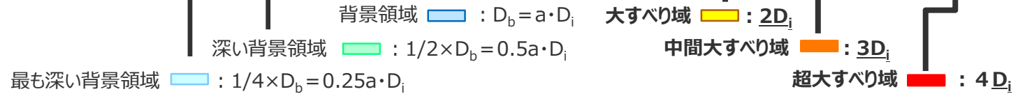
遷移領域のすべり量D(m)の設定方法
