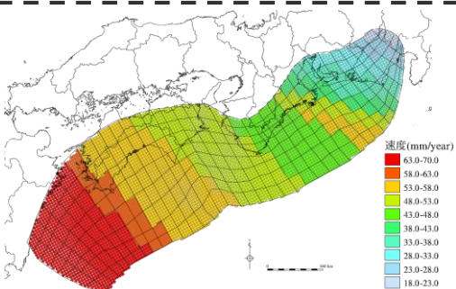
各小断層の沈み込速度分布 (Loveless and Meade(2010)を基に作成)
