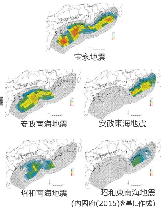
既往地震の津波断層域と発生履歴
