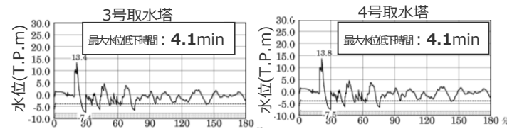
水位の時刻歴波形 ・網掛け部の上端は当該地点の標高 ・点線は取水塔呑口下端レベル ・朔望平均干潮位T.P. - 0.93mを考慮
