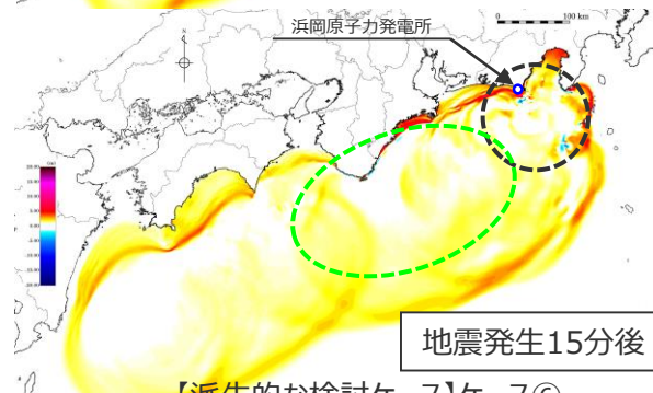
内閣府の最大クラスモデルの津波伝播状況スナップショット
