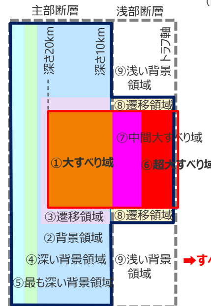
内閣府の最大クラスモデルのすべり量分布概念図（ケース①の例）
