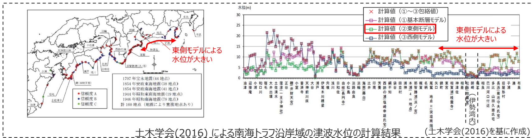
土木学会(2016)モデル (土木学会(2016)を基に作成)
