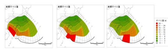
相模トラフ沿いの最大クラスの地震による津波の波源モデル (内閣府(2013)に基づき作成)
