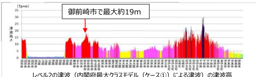
レベル2の津波(内閣府最大クラスモデル(ケース①)による津波)の津波高 (静岡県(2015)に基づき作成)
