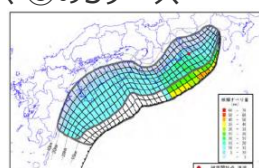
内閣府最大クラスモデル(ケース①)の波源モデル (内閣府(2012))
