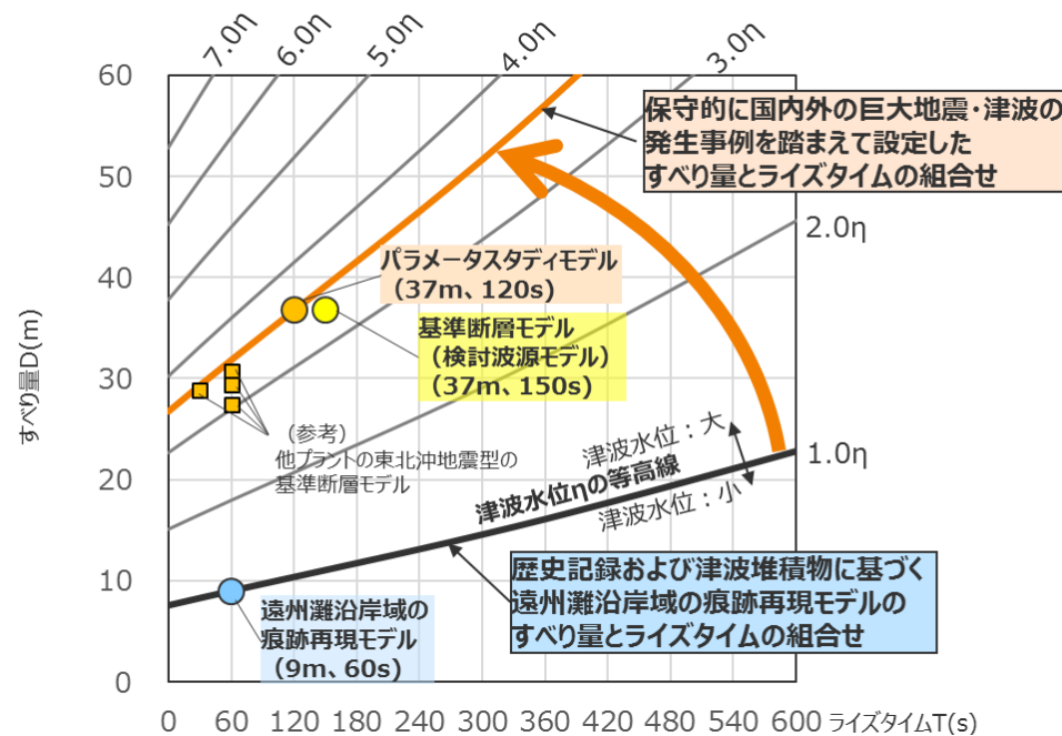
国内外の地震のすべり量とライズタイムの組合せの比較分析結果
