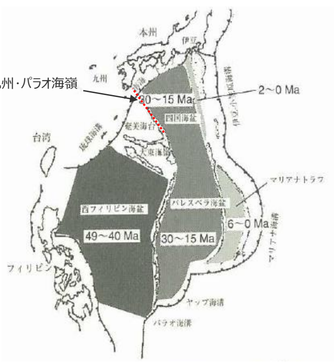
フィリピン海プレートを構成する海盆の年代 (Okino et al.(1998)などによる、Seno(2000)に加筆)
