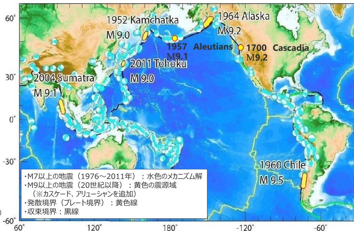
Global CMT による M ≥ 7 の地震 (佐竹 (2012) を基に作成)
