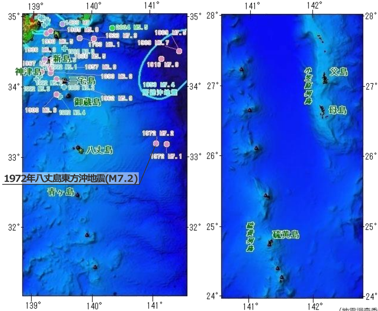
伊豆・小笠原海溝周辺の主な過去の地震
