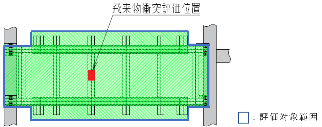
第 2 -20 図 相対する 2 辺以上で支持する防護板 飛来物衝突評価 (鉛直) 位置
