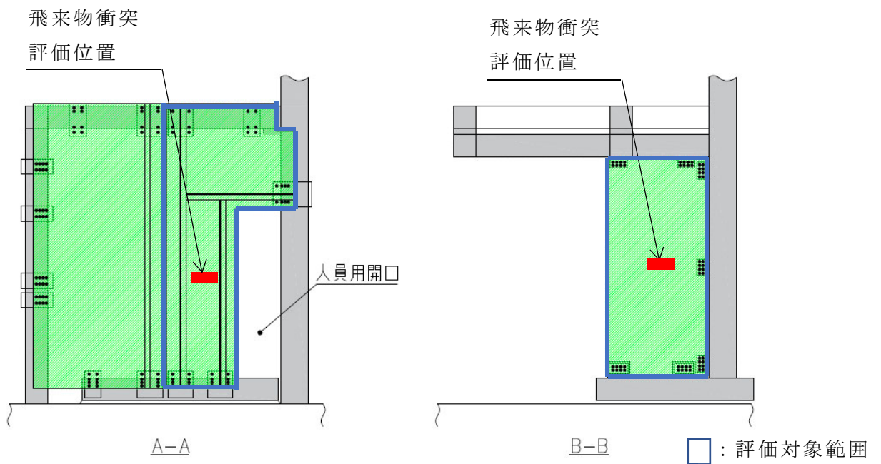
第 2 -21 図 相対する 2 辺以上で支持する防護板 飛来物衝突評価 (水平) 位置
