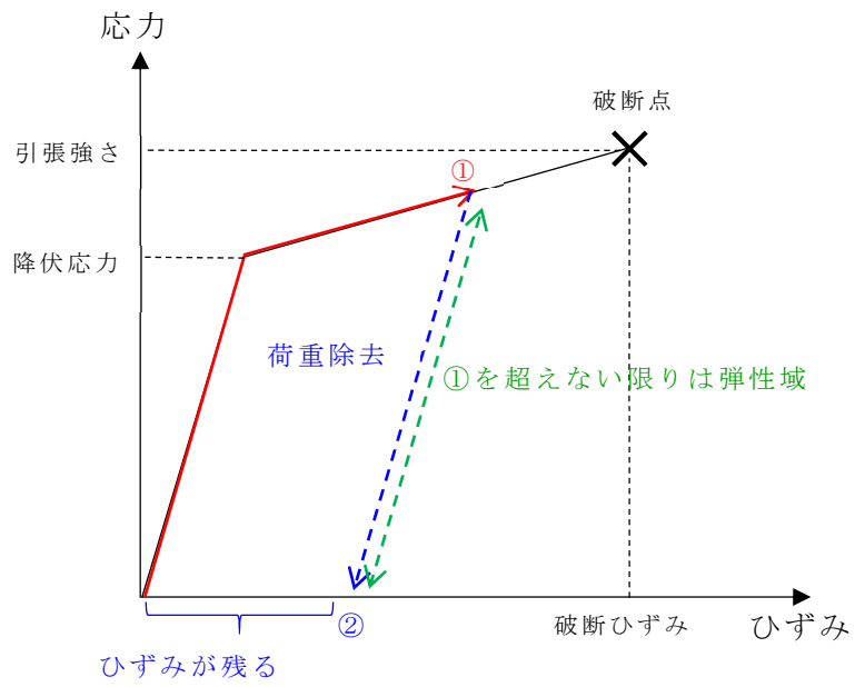
第 2 -22 図 取付ボルトの応力—ひずみ線図
