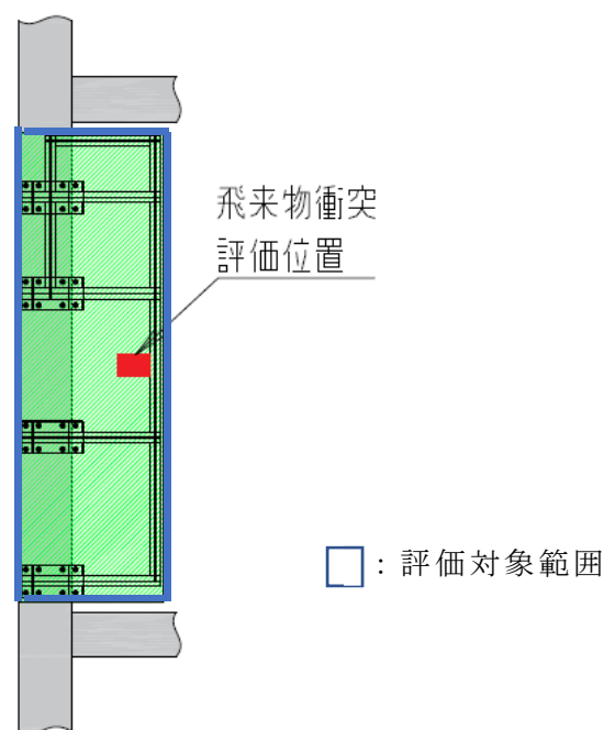
第 2-19 図 1 辺で支持する防護板 飛来物衝突評価（水平）位置
