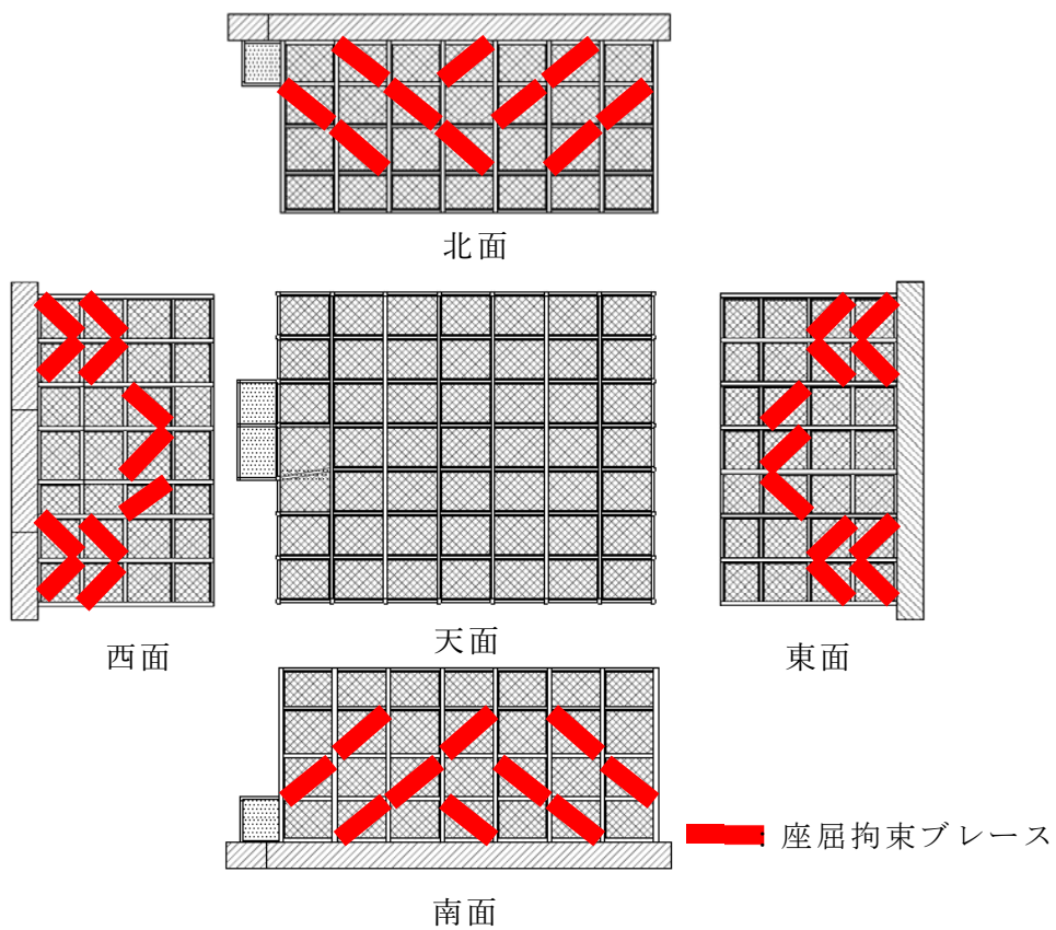
第 2 -25 図 座屈拘束ブレースの配置概要
