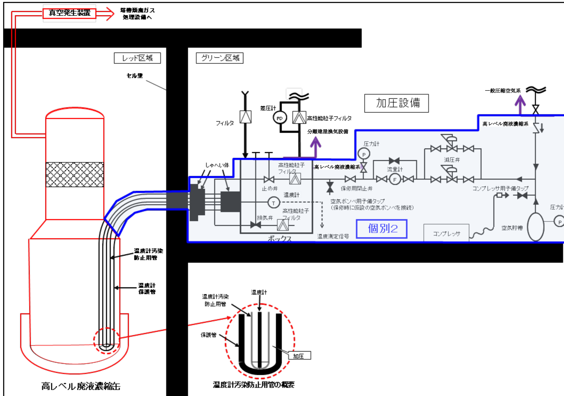
第4-2図 高レベル廃液濃縮缶及び温度計保護管と加圧設備に係る主流路の範囲及び主流路としていない範囲の概要図
