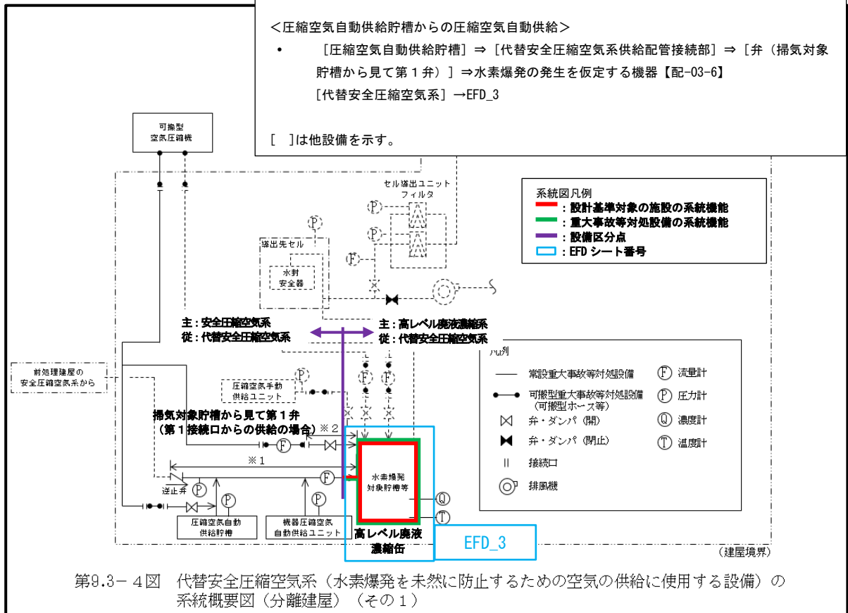
第3-12図 代替安全圧縮空気系（水素爆発を未然に防止するための空気供給に使用する設備） 系統概要図（第1接続口からの空気供給）（兼用配管を含む場合） （事業変更許可申付書類六 第9.3-4図抜粋）
