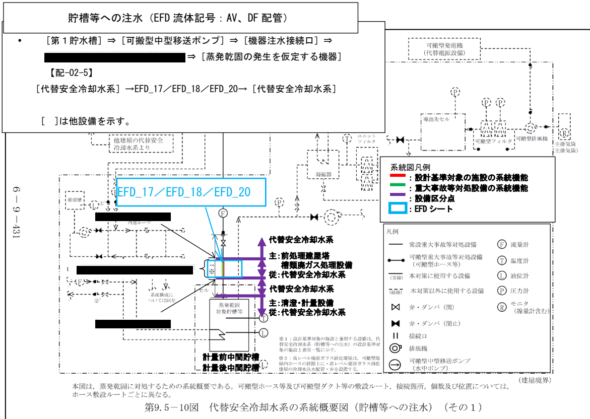
第3-3図 代替安全冷却水系 系統概要図（貯槽等への注水）
