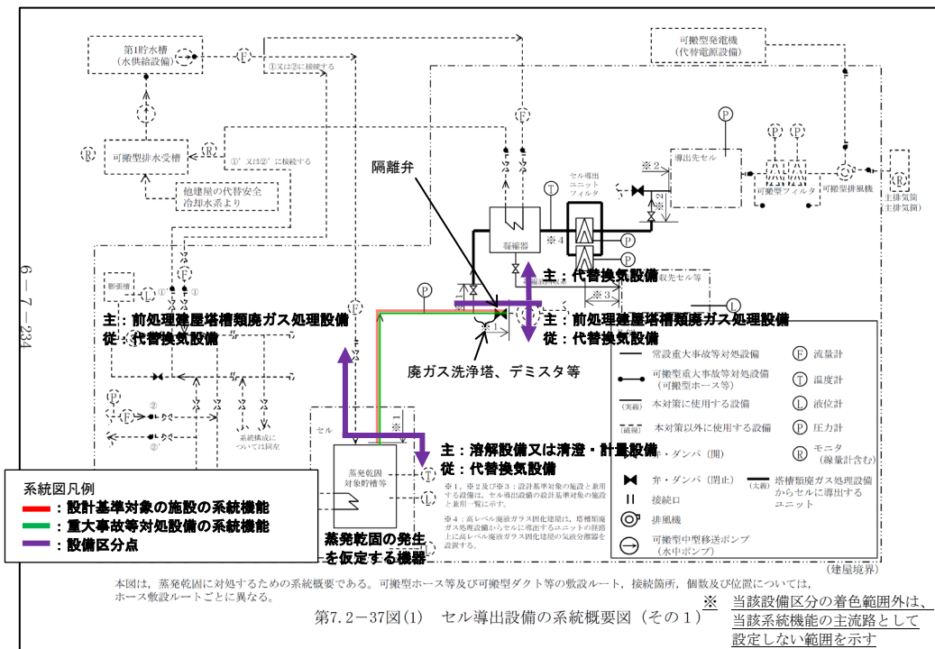
第2-4図 代替換気設備 系統概要図 (事業変更許可申請書 添付書類六 第7.2-37図(1)抜粋)
