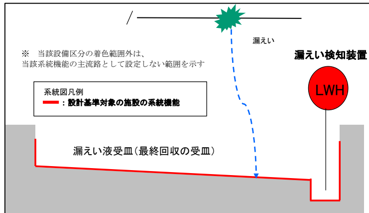
第2-4図 漏えいした溶液（プルトニウムを含む溶液又は抽出廃液）の保持 （漏えいした溶液の保持）
