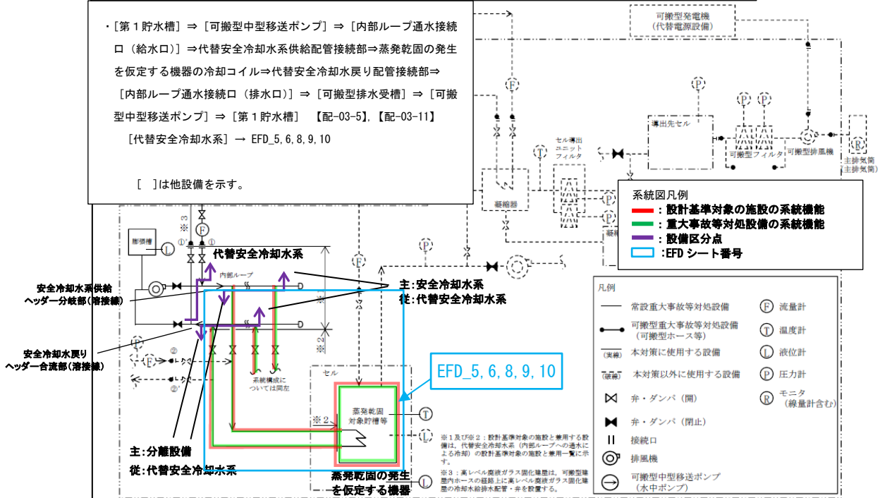
第9.5-7図 代替安全冷却水系の系統概要図 (内部ループへの通水による冷却) (その1)
