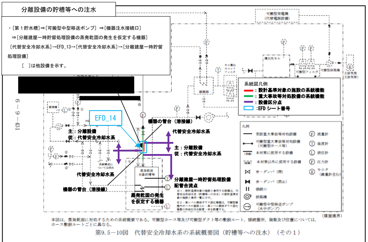
第3-10図 (2) 代替安全冷却水系 系統概要図 (貯槽等への注水) (兼用配管を含む場合) (計装用空気ライン以外からの貯槽等への注水その1) (事業変更許可申請書 添付書類六 第9.5-10図抜粋)
