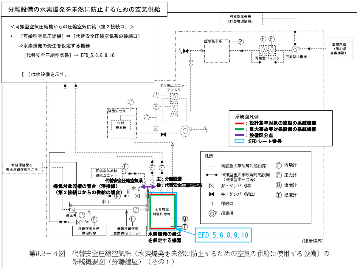
* 1 : 水素掃気配管・弁、* 2 : 機器圧縮空気供給配管・弁 第 3 - 15 図 代替安全圧縮空気系（水素爆発を未然に防止するための空気供給に使用する設備）の系統概要図（2） （事業変更許可申付書類六 第9. 3-7図抜粋）
