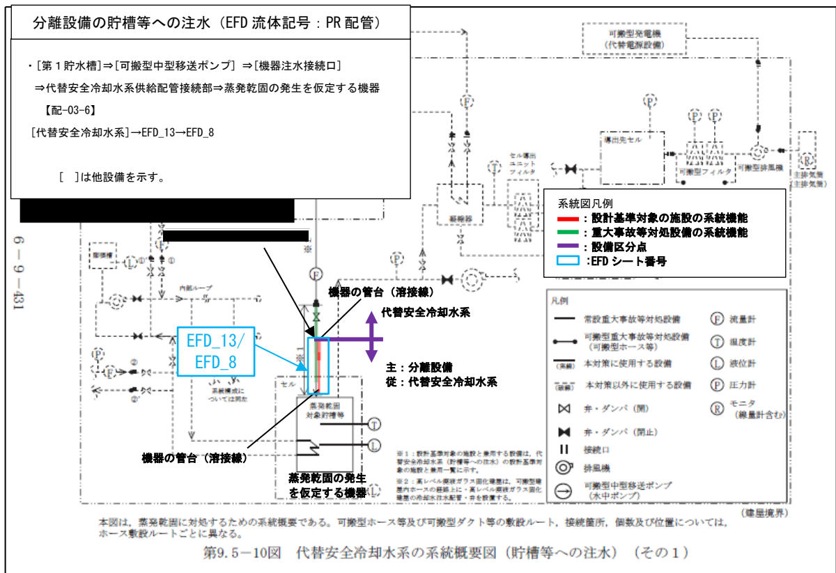
第 3-10 図 (3) 代替安全冷却水系 系統概要図 (貯槽等への注水)
