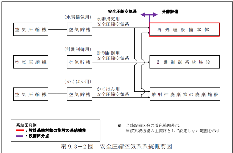
第 2-9 図 安全圧縮空気系 系統概要図
