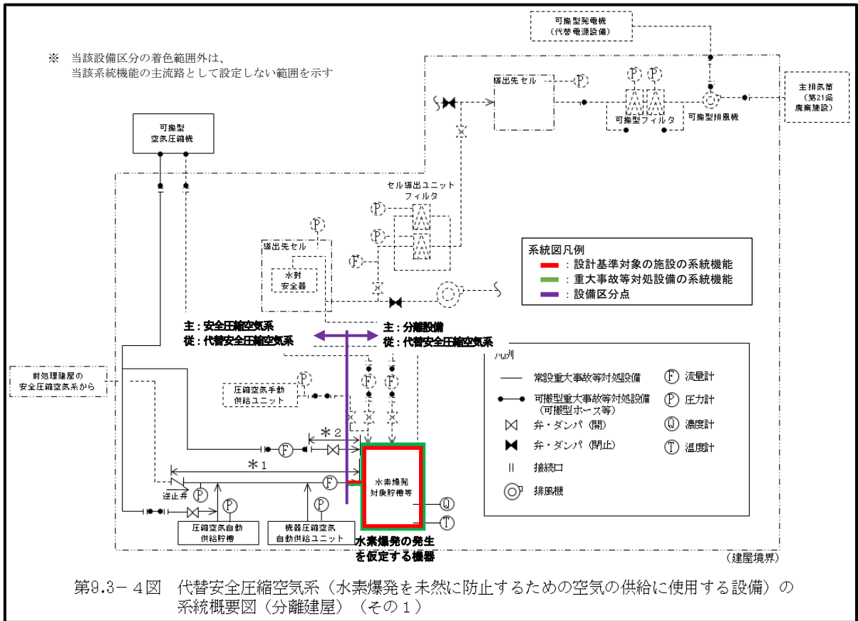
第2-16図 代替安全圧縮空気系 (水素爆発を未然に防止するための空気供給に使用する設備) の系統概要図 (兼用配管を含む場合) (事業変更許可申付書類六 第9.3-4図抜粋)
