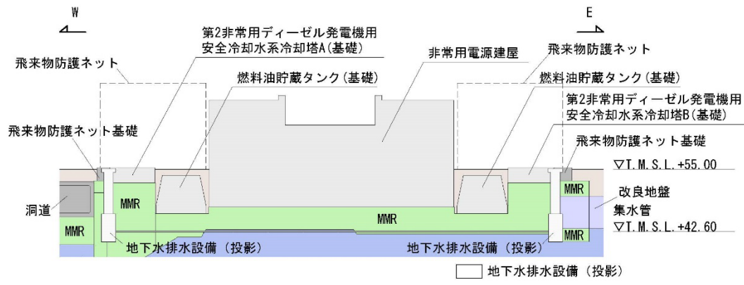
B - B 立面図
