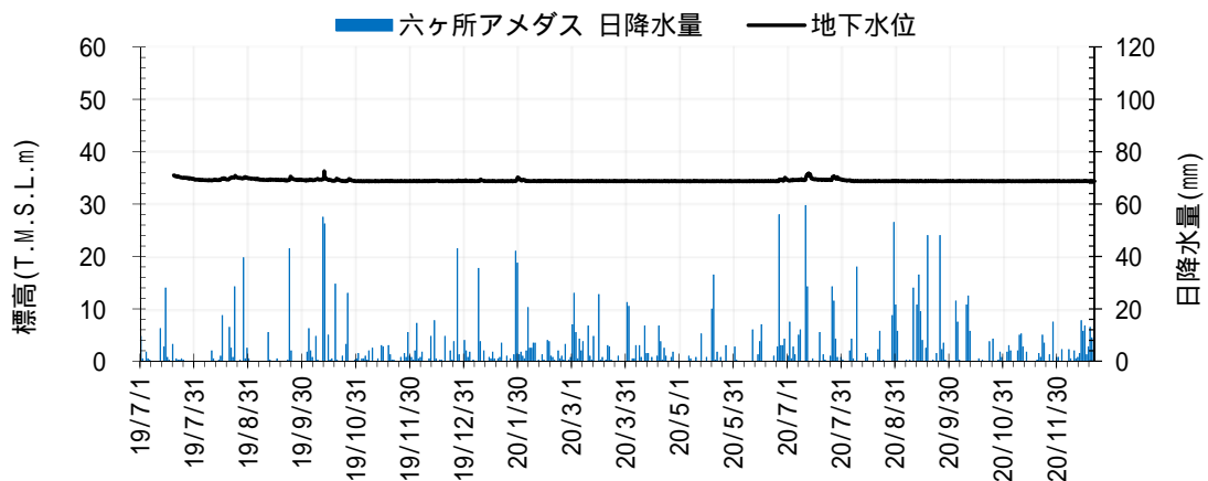
第 1.-1 図(4) GW-01 孔における地下水水位観測記録と降水量データ
