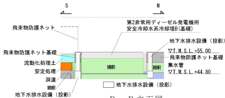
B - B 立面図
