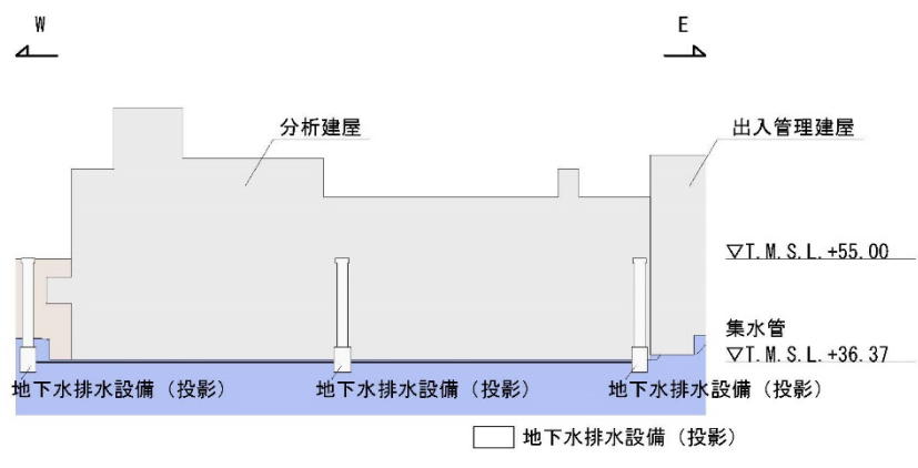
B - B 立面図
