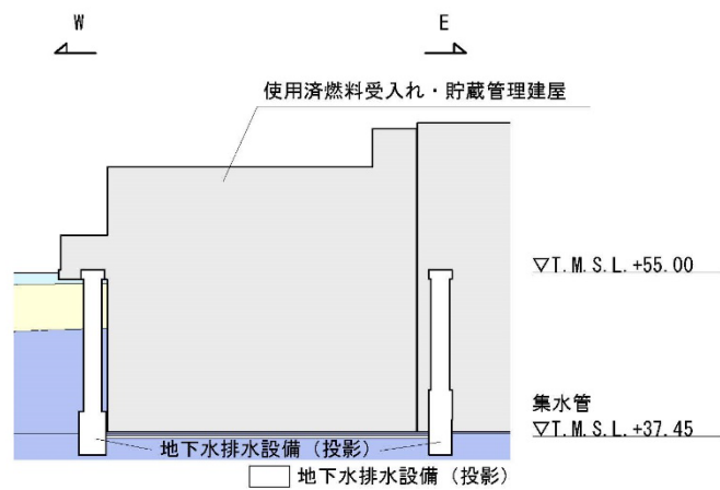
B - B 立面図
