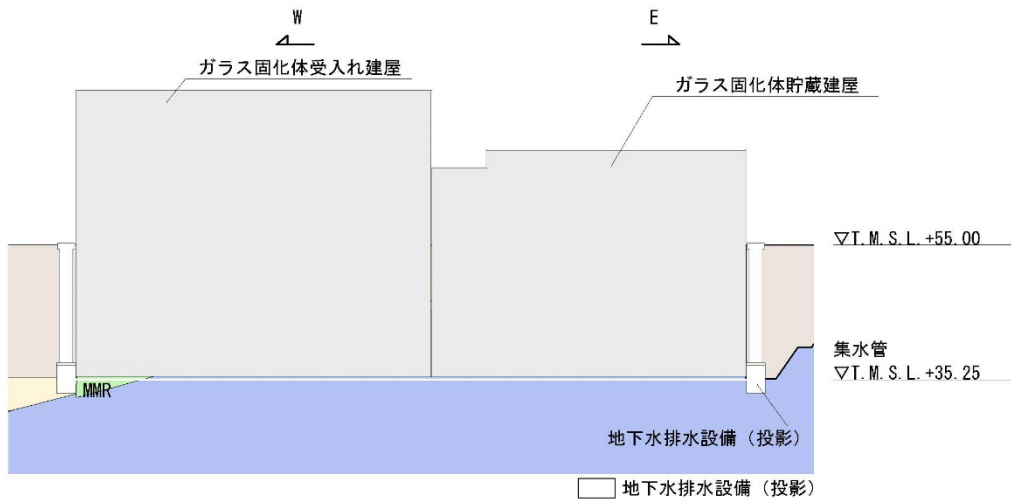
B - B 立面図
