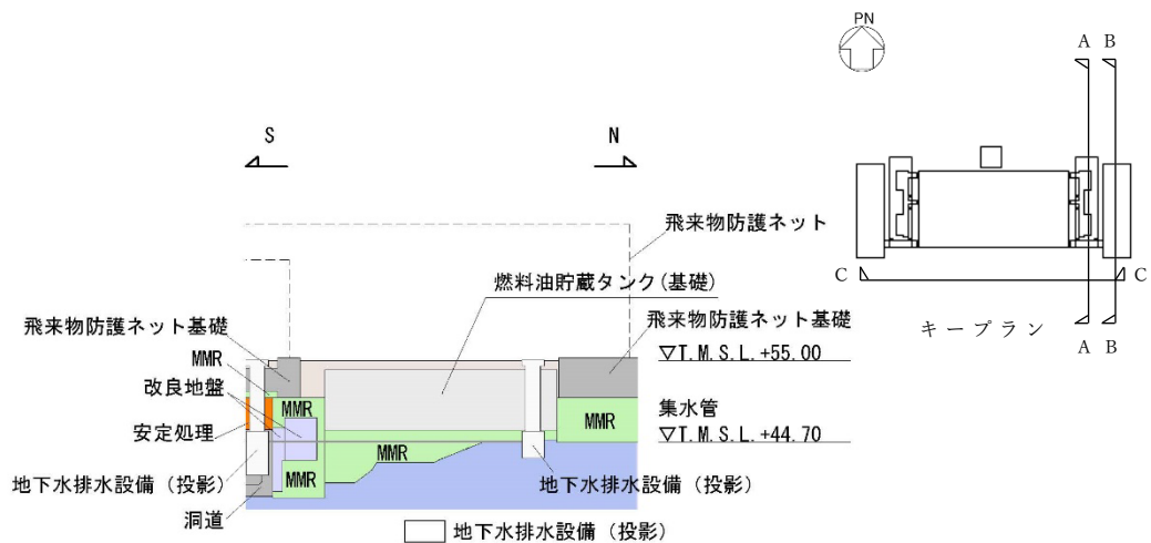
A - A 立面図
