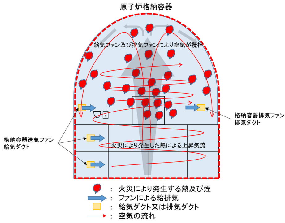
第 3-2-6 図 給気ファン及び再循環ファンの停止時（格納容器送気・排気ファンは運転）における火災による熱及び煙の流れ
