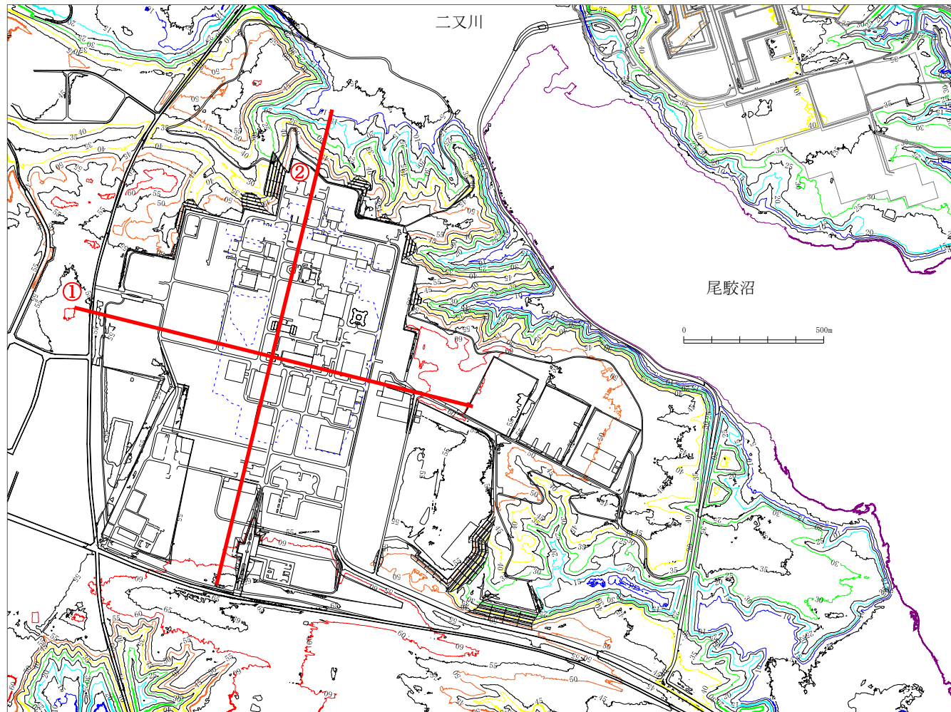
第 5.3.2-1 図 敷地周辺の地形図
