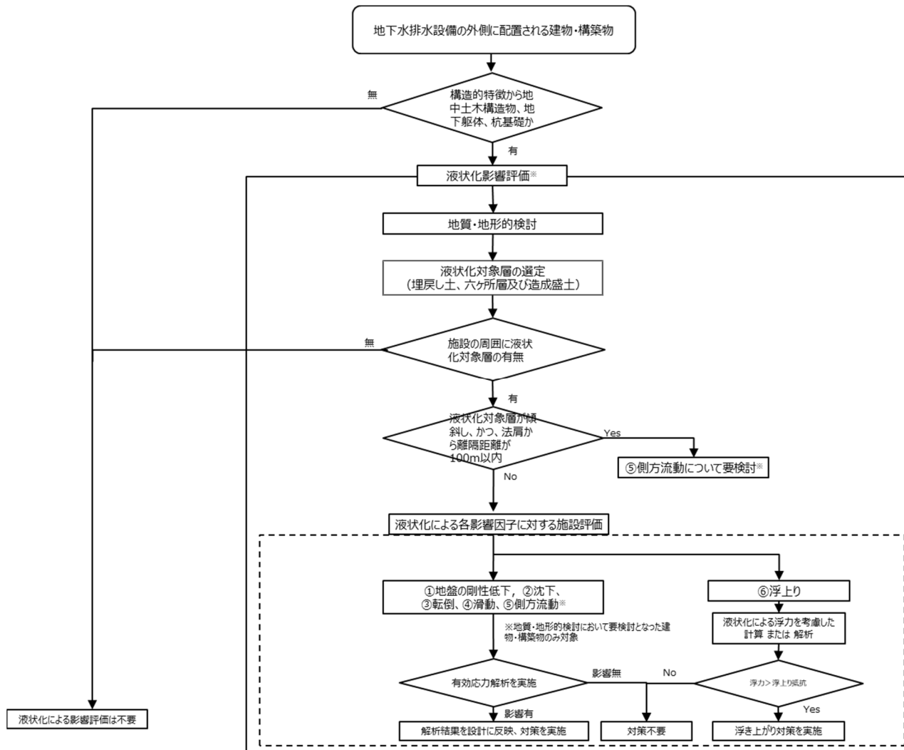
第 5.1-2 図 液化化影響評価 対象施設の検討フロー
