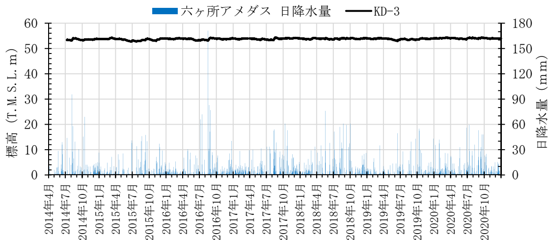
第 1. -2 図 (2) KD-3 孔における地下水位観測記録と降水量データ (長期)
