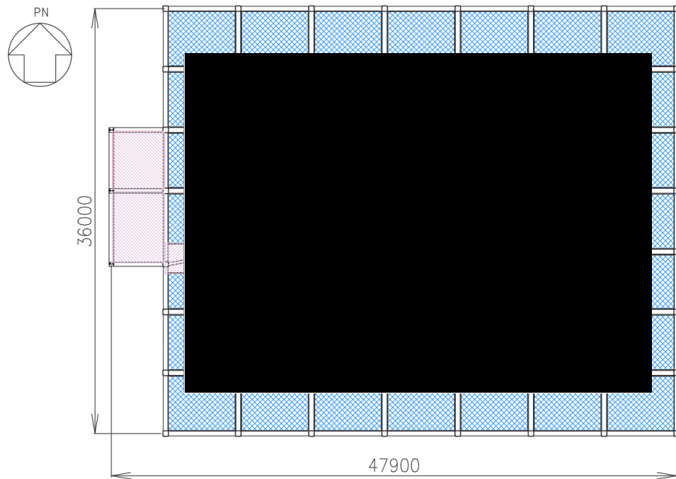
A視 (T.P.+75600)
