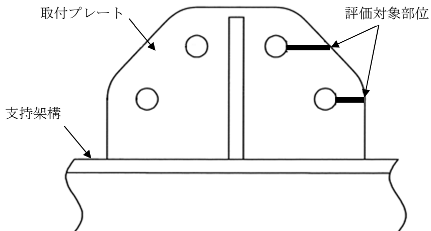
第3.1.1-3図 隅角部固定ボルトの評価対象部位
