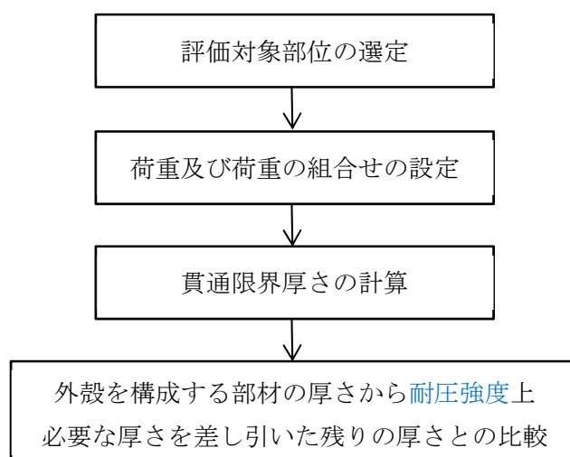
第2.3-1図 配管の衝突評価フロー
