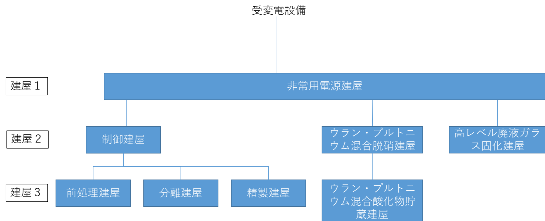
第2-3表 建屋間で取り合う落雷防護対象施設のうち電気設備
