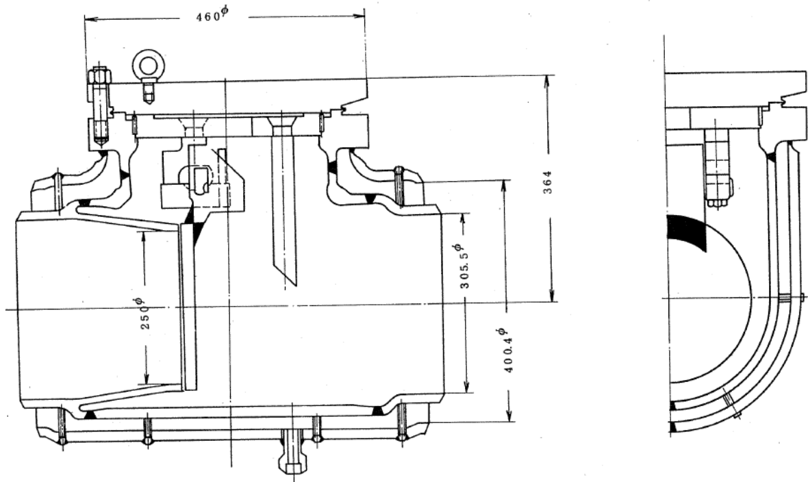
第5図 1次主冷却系の逆止弁
