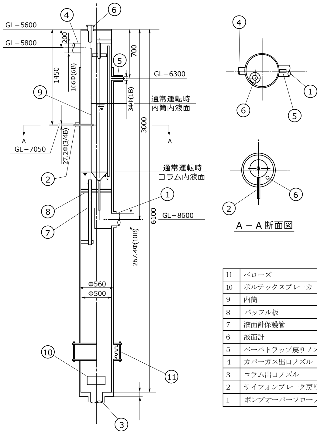
第4図 オーバフローカラム
