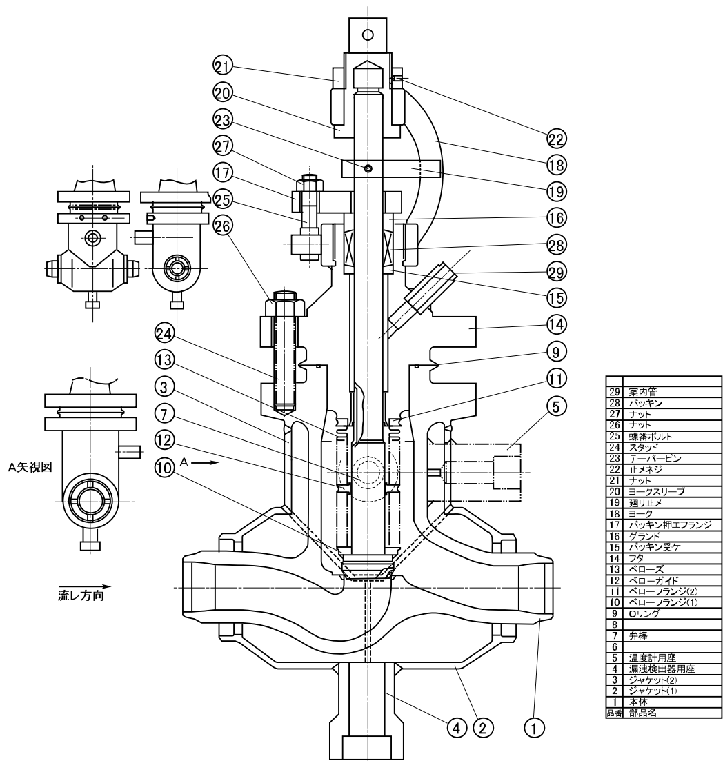
第 6 図 1 次主冷却系圧力計止弁
