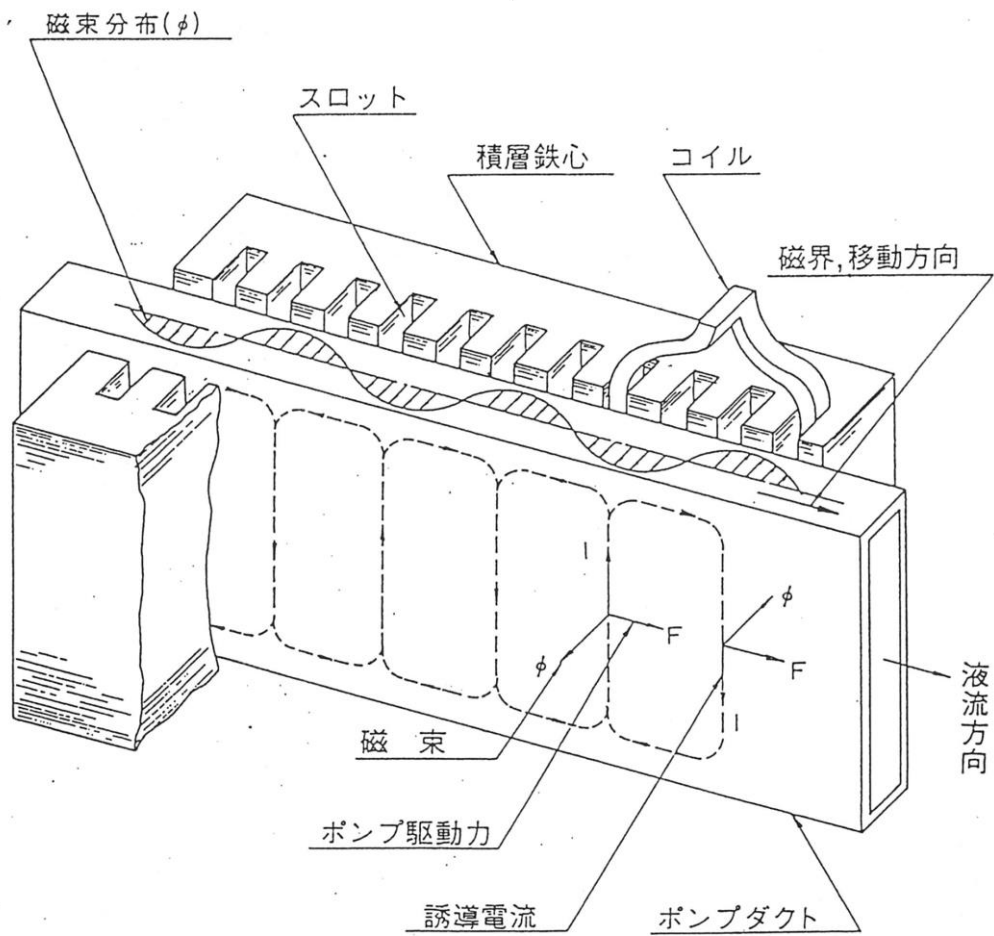
第2図 1次補助冷却系循環ポンプ
