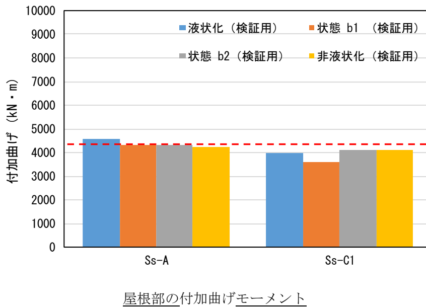
第7.5.2-1図 検証用モデルの中間状態における応答値比較
