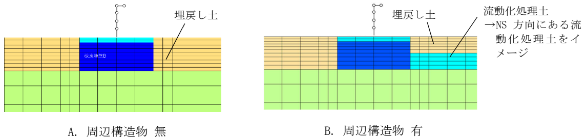
第4.1-1図 設計モデル(A：周辺構造物 無)と 確認用モデル(B：周辺構造物 有)
