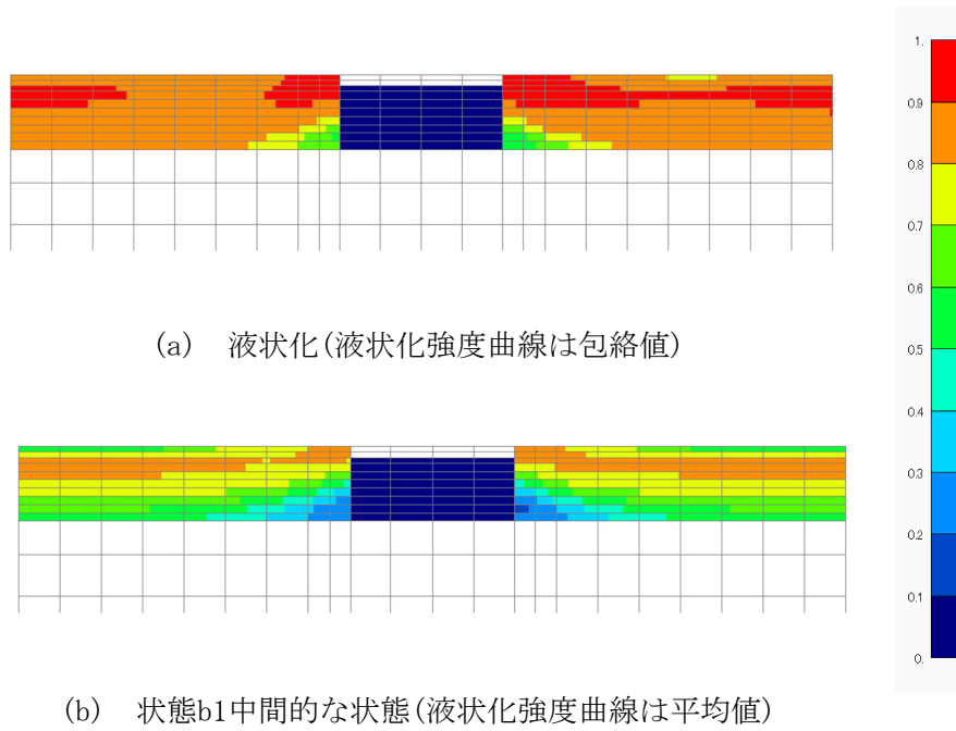
第6.1.2-12図 最終時刻(20秒加振後)の過剰間隙水圧比分布(Ss-C1)
