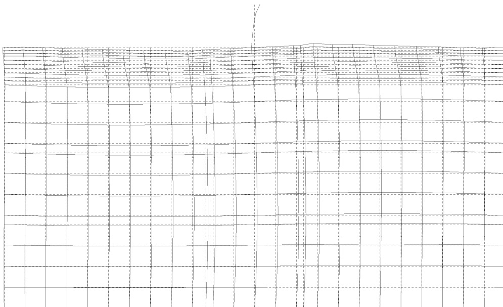
(b) 確認用モデル(B : 改良地盤幅 大) (モデル全体のモード次数 : 6次, 固有振動数 : 3.65Hz, 固有周期 : 0.27s) 第3.2-4図 ロッキングが卓越する固有値解析結果
