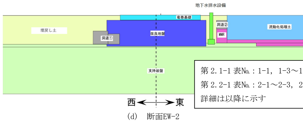
第2.3-1図 飛来物防護ネット架構周辺の地中状況図(2/2) 断面図
