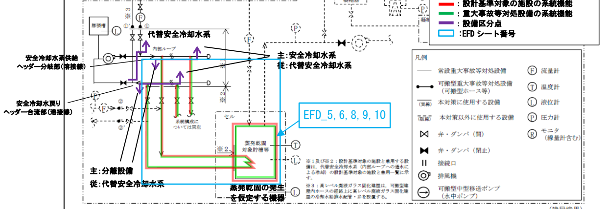
第9.5-7図 代替安全冷却水系の系統概要図 (内部ループへの通水による冷却) (その1)
