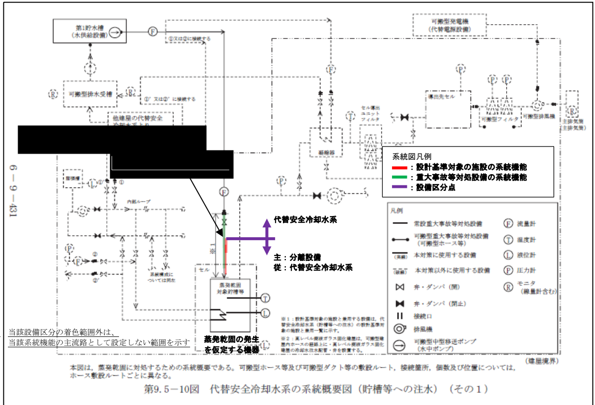
第2-13図 (3) 代替安全冷却水系 系統概要図 (計装用空気ライン以外からの貯槽等への注水その2) (事業変更許可申請書 添付書類六 第9.5-10図抜粋)
