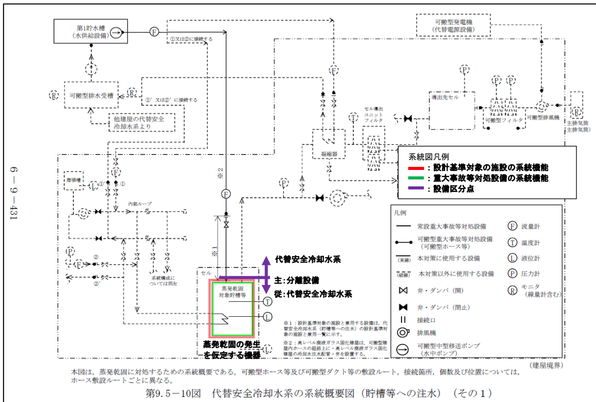
第2-13図 (1) 代替安全冷却水系 系統概要図 (事業変更許可申請書 添付書類六 第9.5-10図抜粋)
