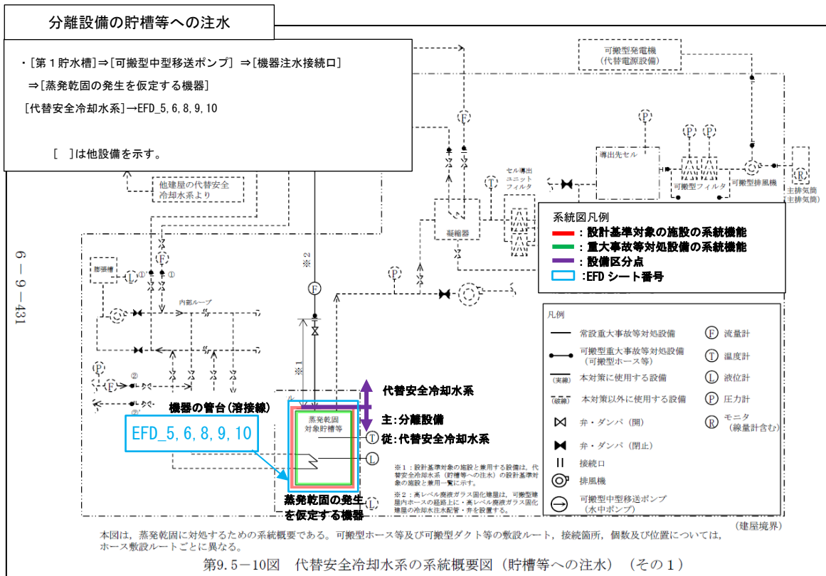
第3-10図 (1) 代替安全冷却水系 系統概要図 (事業変更許可申請書 添付書類六 第9.5-10図抜粋)
