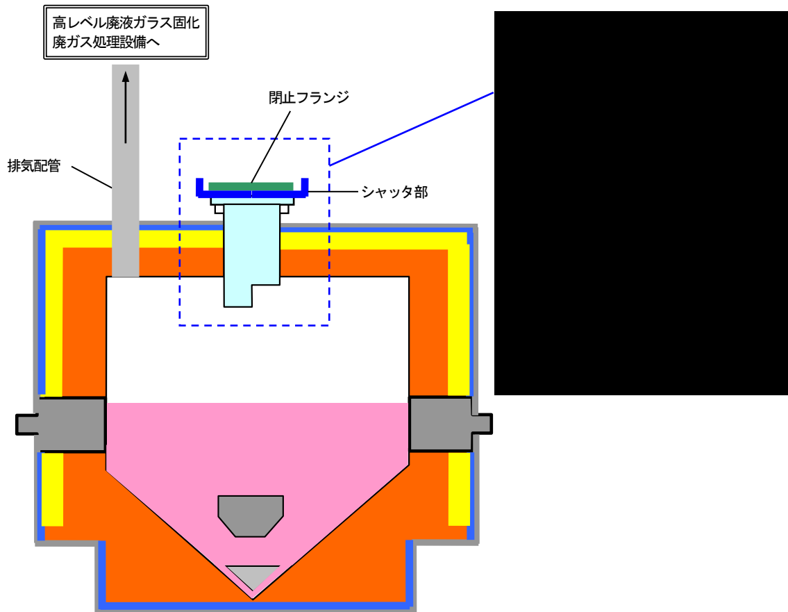
第4-3図 保守治具入り口シャッタ 据付図
