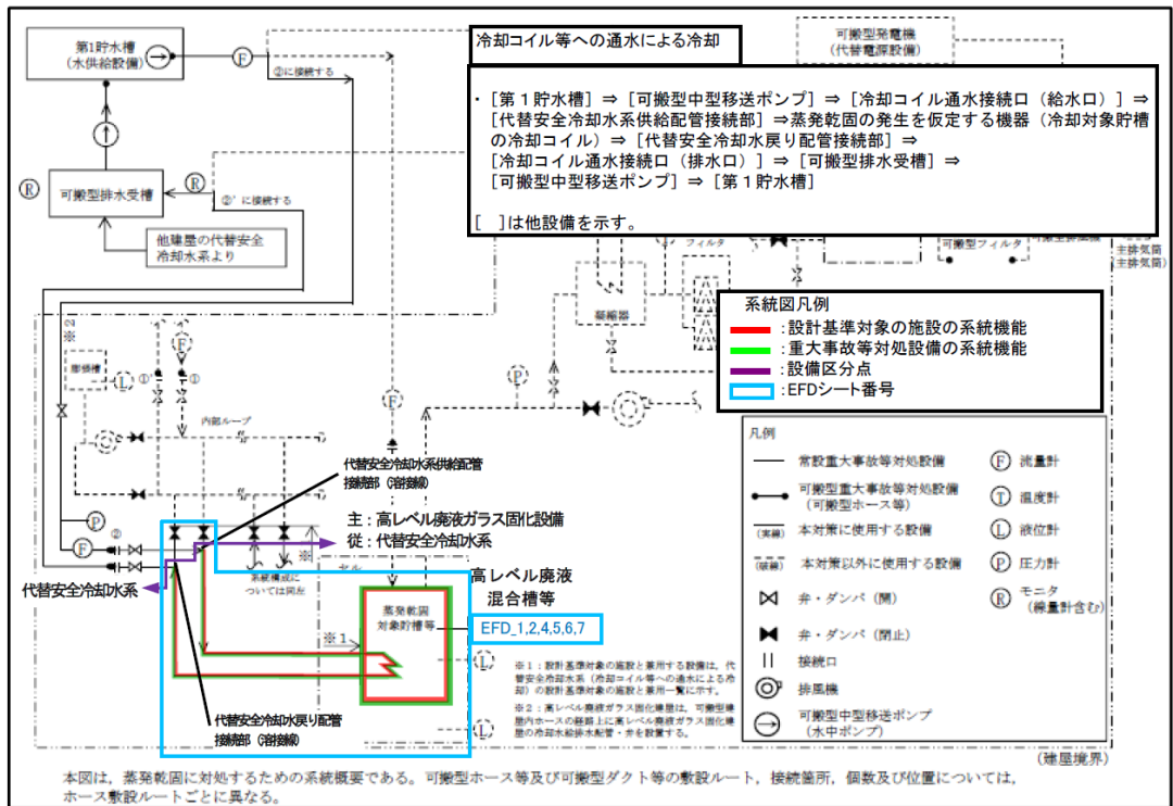
第3-11図 代替安全冷却水の系統概要図 (冷却コイル等への通水による冷却)
