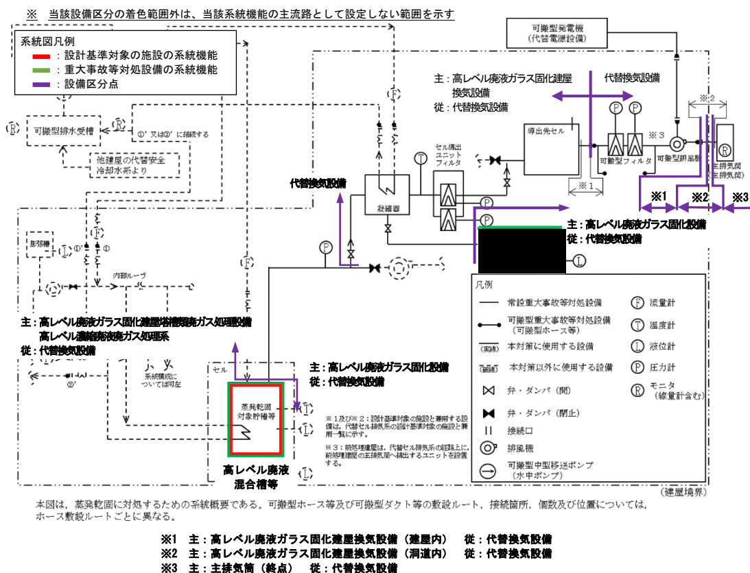
第2-13図 代替換気設備の系統概要図
