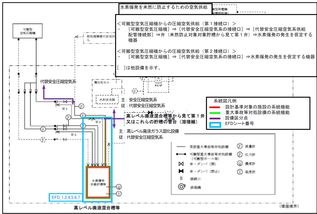
第3-13図 代替安全圧縮空気系（水素爆発を未然に防止するための空気の供給に使用する設備）の系統概要図 （事業変更許可申請書 添付書類六 第9.3-7図抜粋）
