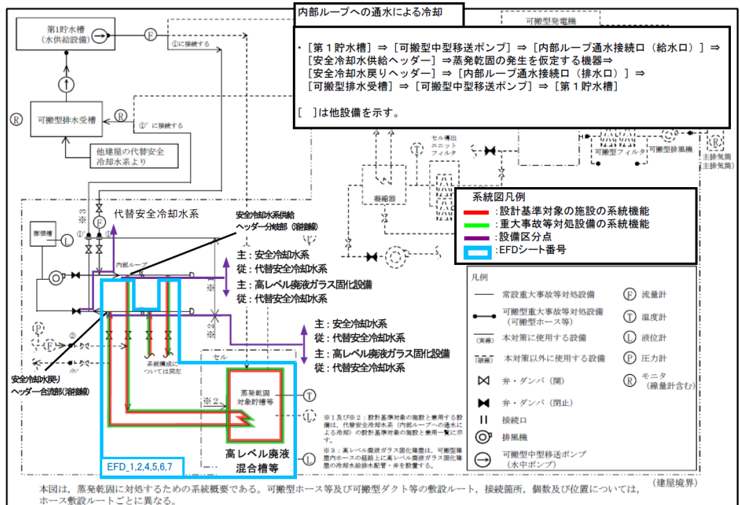
第3-8図 代替安全冷却水系の系統概要図 (内部ループへの通水による冷却)
