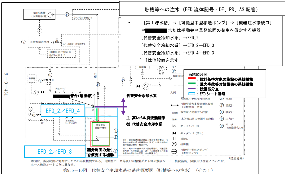
第3-7図 代替安全冷却水系 系統概要図 (貯槽等への注水) (配管含む場合) (事業変更許可申請書 添付書類六 第9.5-10図抜粋)
