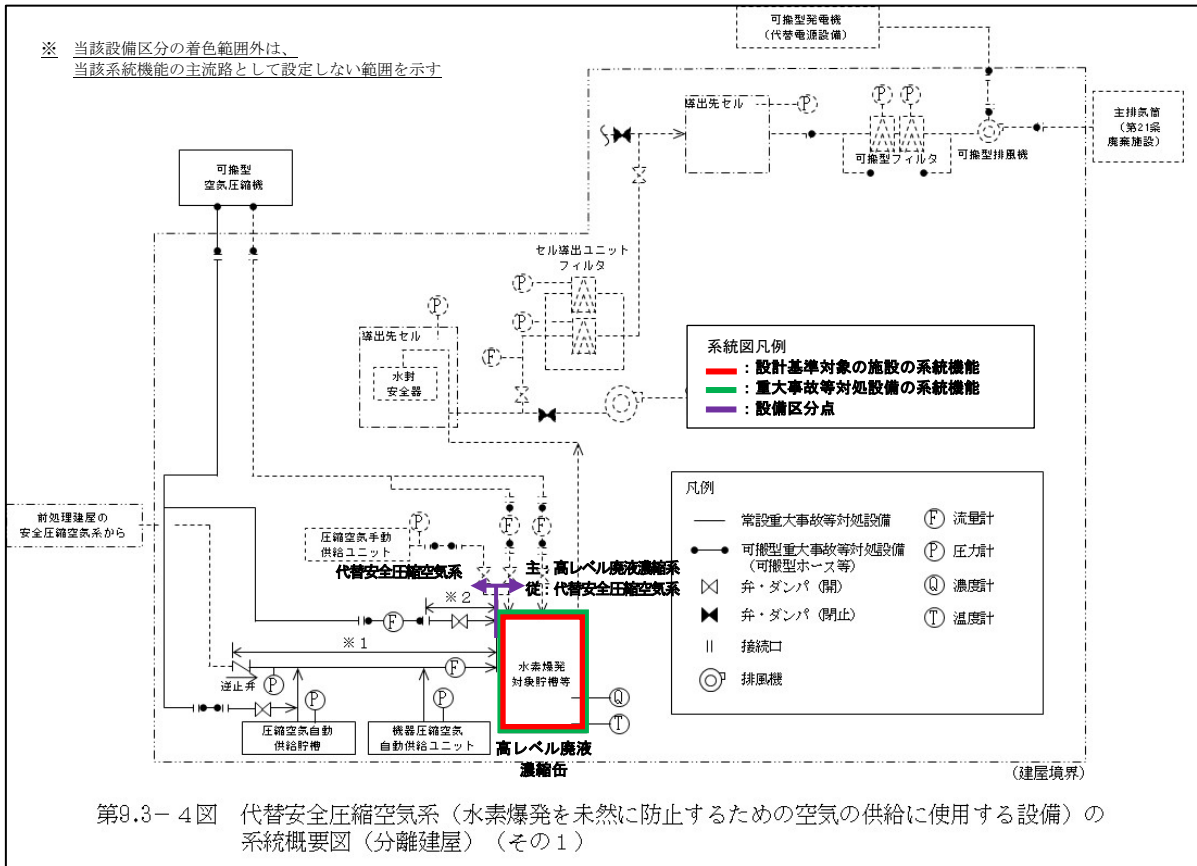
第2-17図 代替安全圧縮空気系（水素爆発を未然に防止するための空気供給に使用する設備）の系統概要図（第2接続口からの空気供給） （事業変更許可申付書類六 第9.3-4図抜粋）
