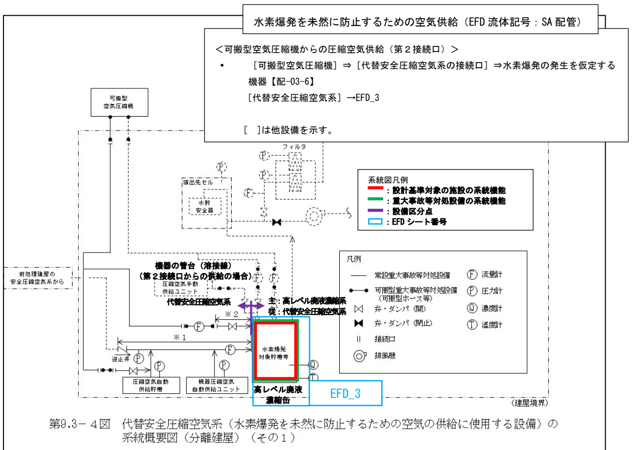
第3-13図 代替安全圧縮空気系（水素爆発を未然に防止するための空気供給に使用する設備） 系統概要図（第2接続口からの空気供給） （事業変更許可申付書類六 第9.3-7図抜粋）
