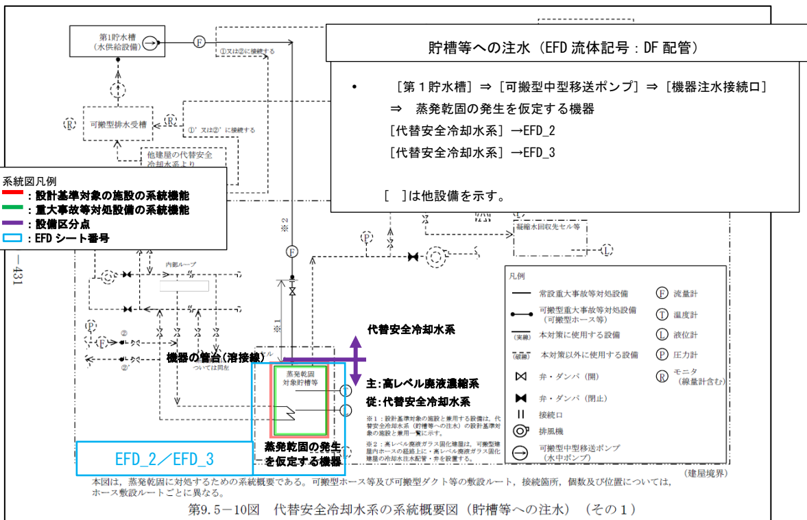
第3-8図 代替安全冷却水系 系統概要図 (貯槽等への注水) (配管含まない場合) (事業変更許可申請書 添付書類六 第9.5-10図抜粋)
