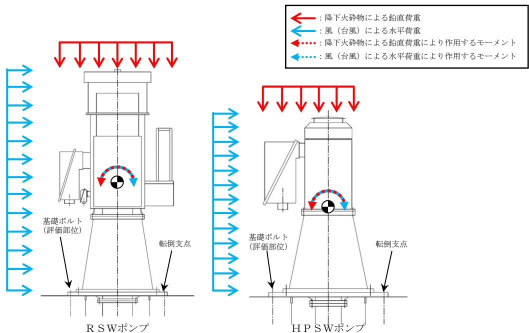
図1 降下火砕物による鉛直荷重の基礎ボルトへの影響概要図
