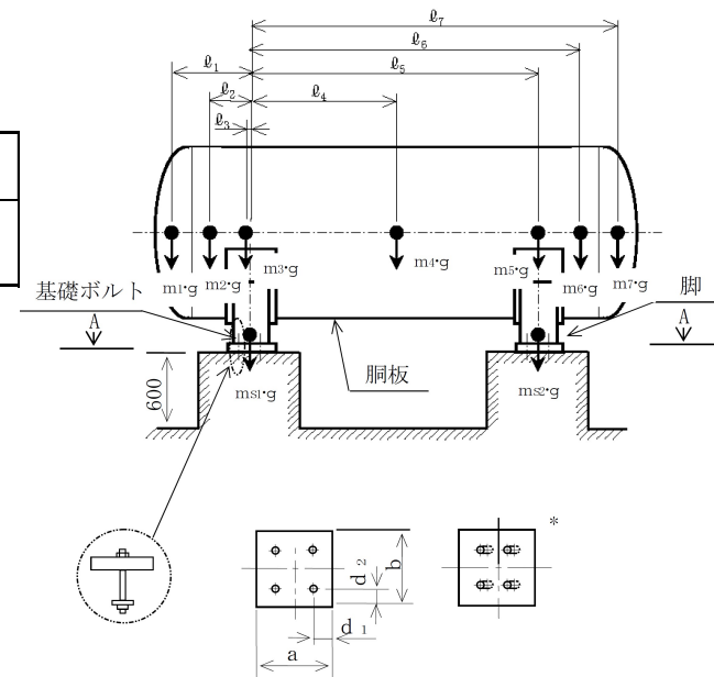
A~A矢視図
