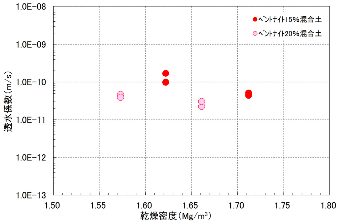
第 3 図 ベントナイト混合率ごとの乾燥密度と透水係数の関係
