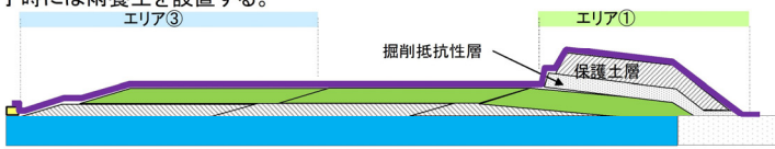
西側トレンチ工事 断面
