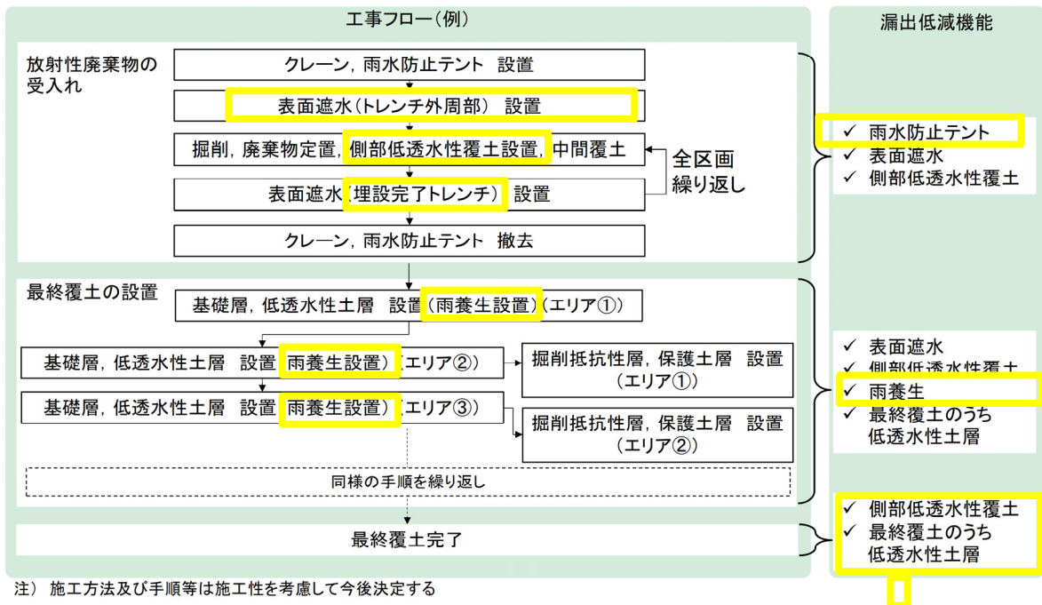
第2図 工事フローと漏出低減機能
