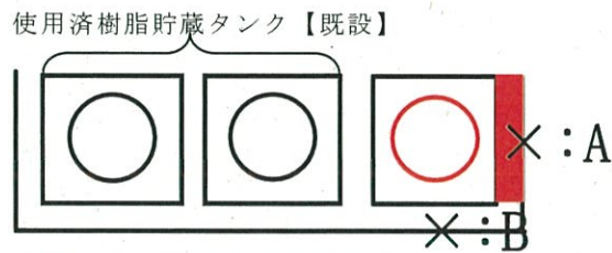
第30-2-23図 評価点 (○ : 使用済樹脂貯蔵タンク、— : 遮蔽壁【増設】)
