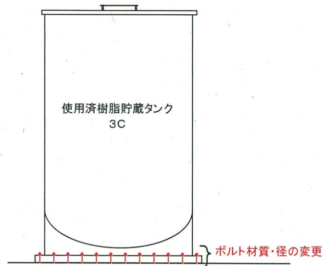
第9-2-23図 新たに設置する使用済樹脂貯蔵タンクの耐震評価に係る既設タンクからの変更箇所
