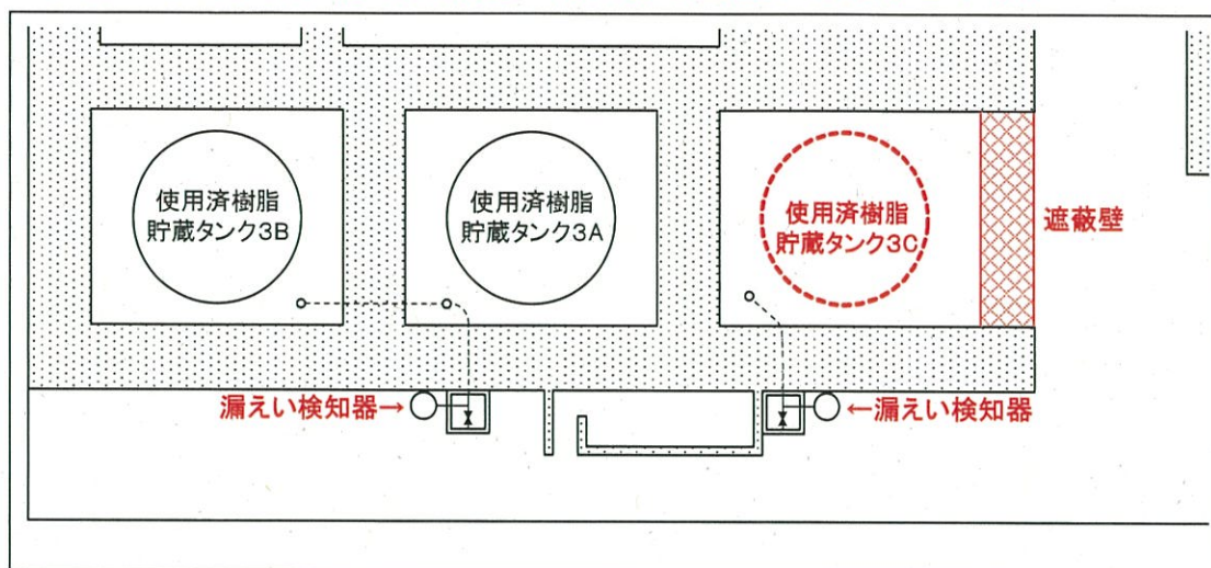
第28-3-1図 使用済樹脂貯蔵タンクの概略配置図
