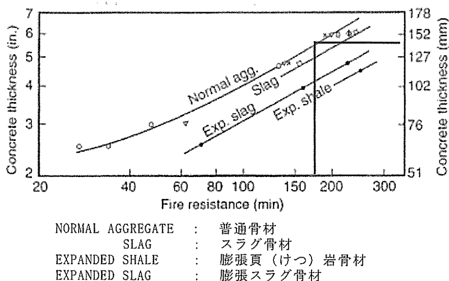
図2 耐火壁の厚さと耐火時間の関係
