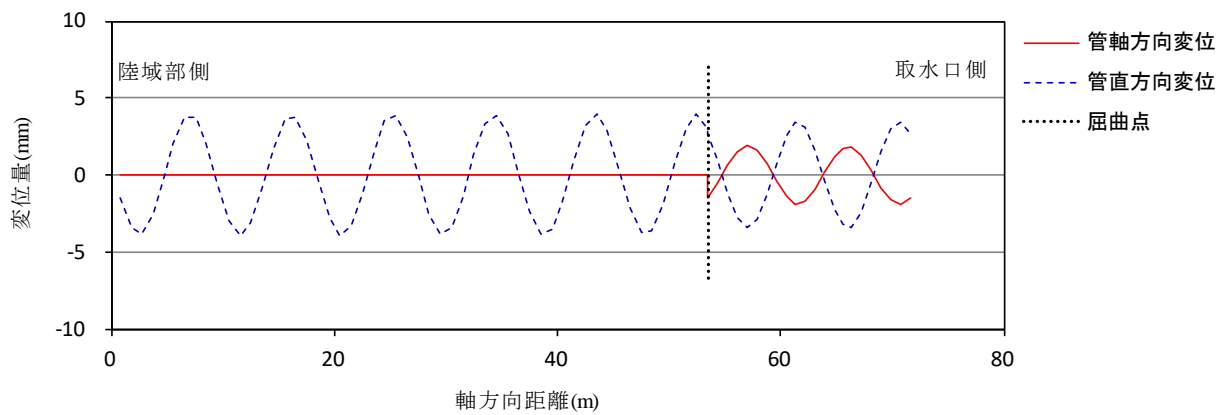
図 5-5 入力地盤変位（入射角 0°）
