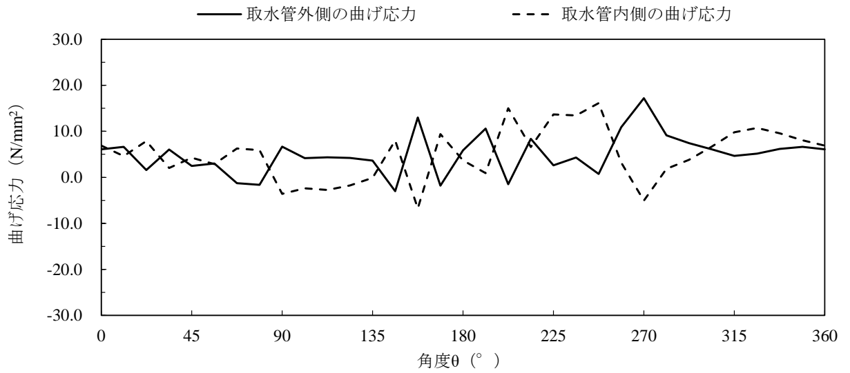
(曲げ応力分布 t=23.66\text{s} )
