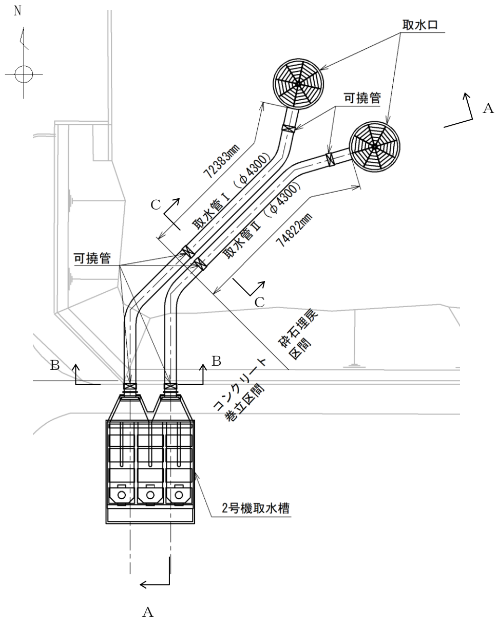
図 2-2 取水管 平面図
