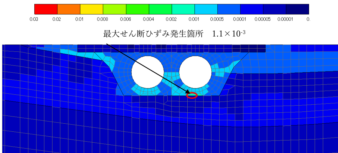
図 3-47 基礎地盤の最大せん断ひずみ分布図 (7/12) (解析ケース①, S_s - N 1 (+ +) )
