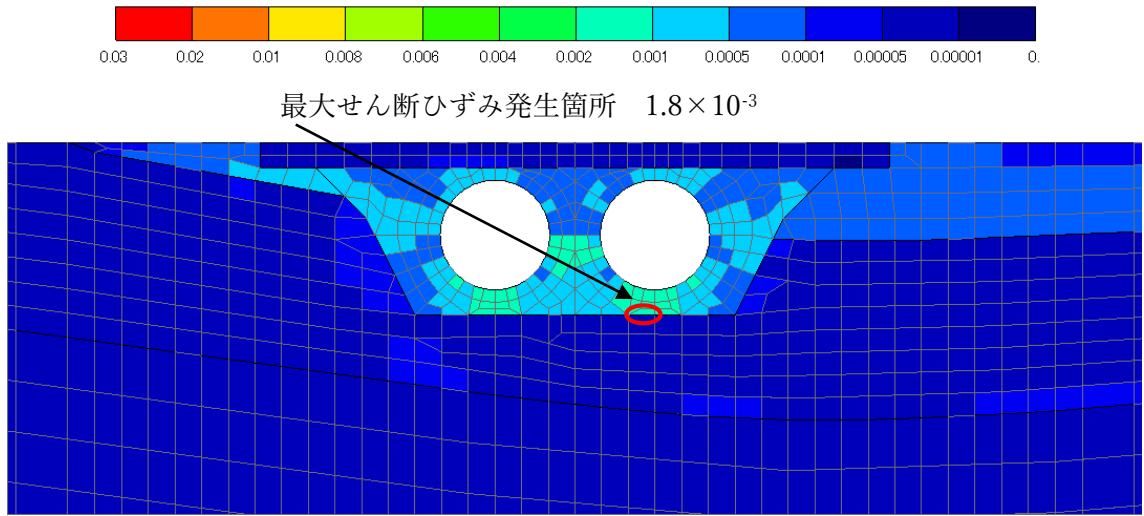
図 3-55 基礎地盤の最大せん断ひずみ分布図 (1/2) (解析ケース②, S_s - F_2 (++) )
