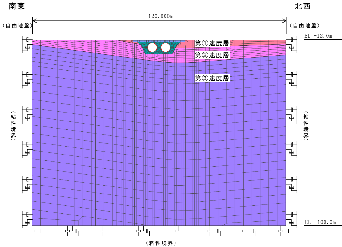
図 3-6 地震応答解析モデル図
