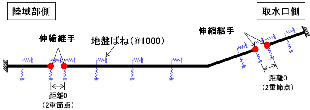
図 5-3 管軸方向解析モデル概念図
