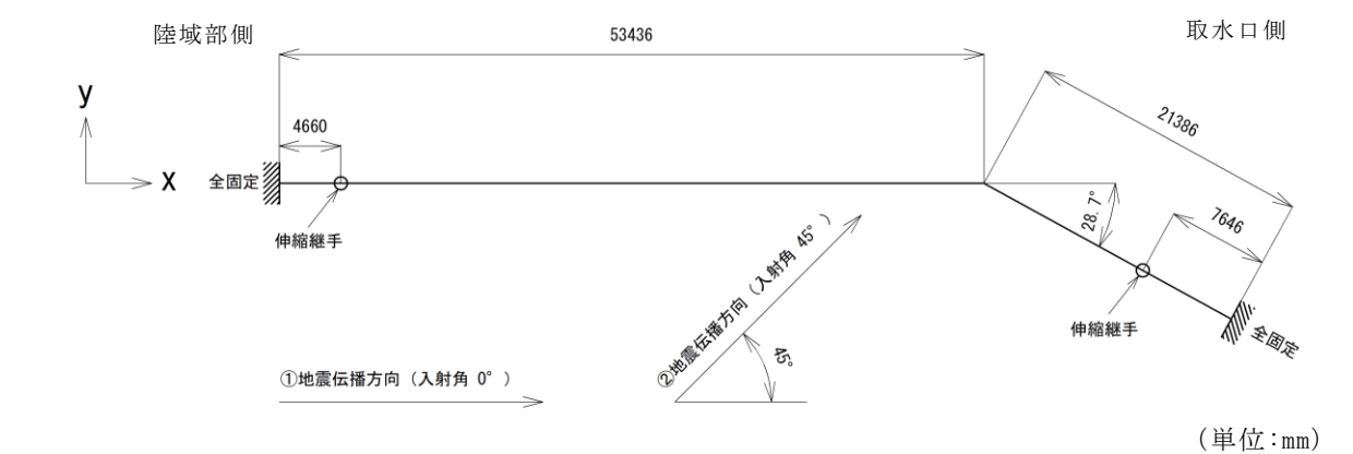
図 5-1 管軸方向の応力解析モデル
