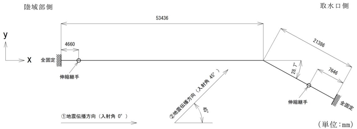
図 5-4 管軸方向の応力解析モデル
