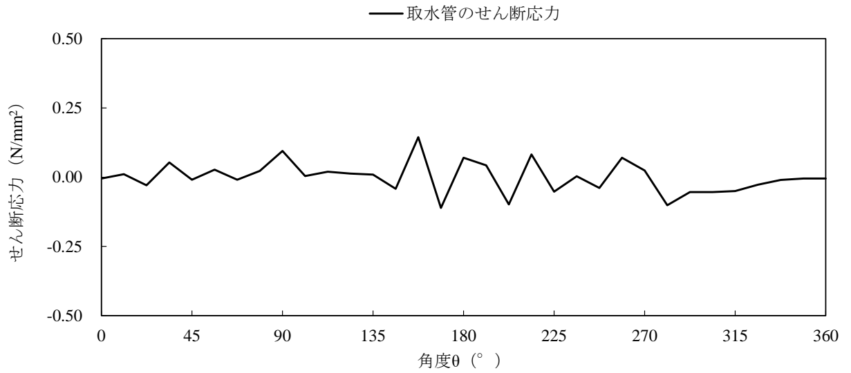
(せん断応力分布 t=23.66\text{s} )
