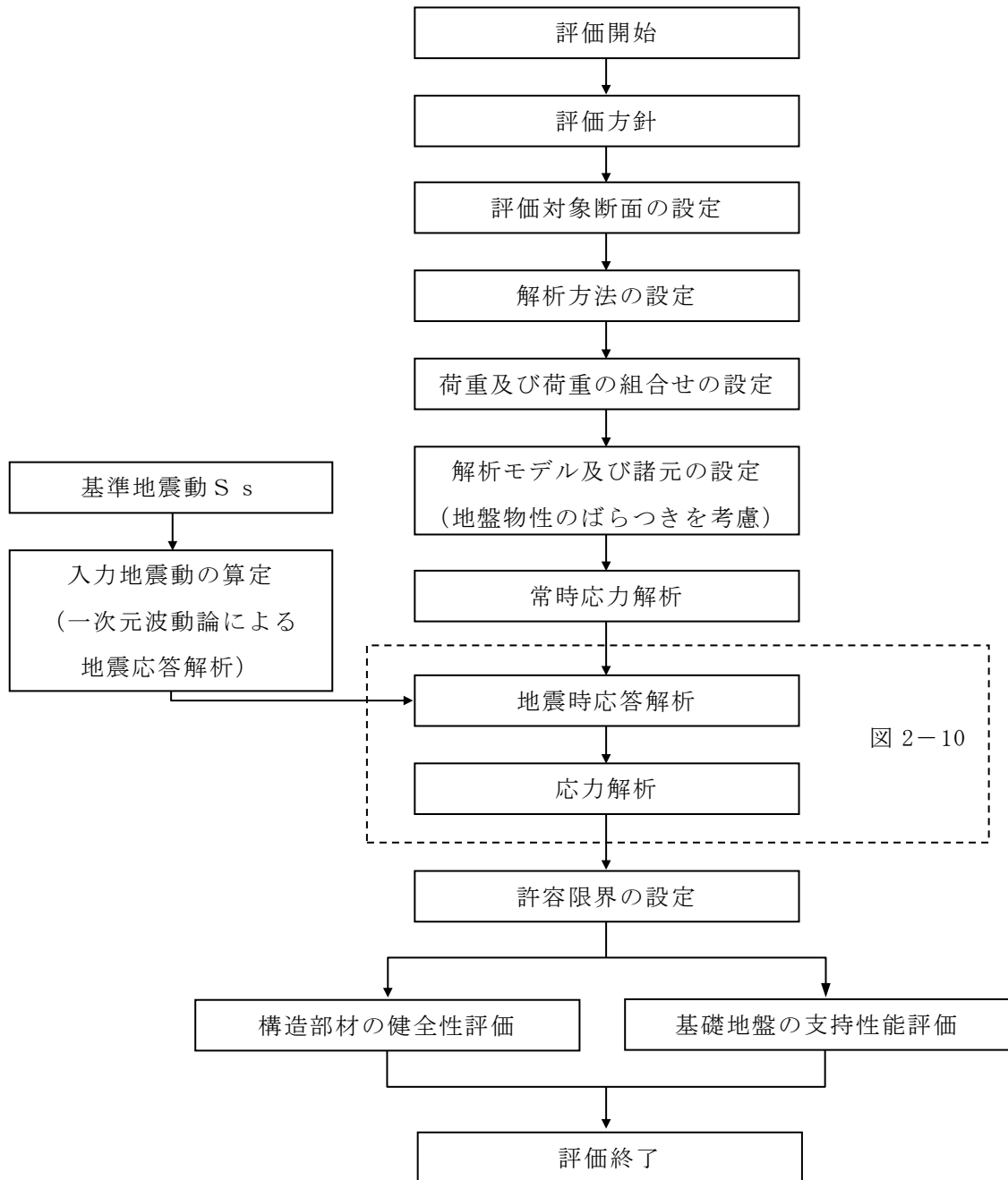
図 2-9 取水管の地震応答解析フロー
