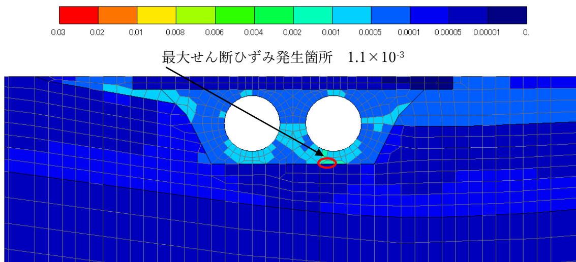
図 3-49 基礎地盤の最大せん断ひずみ分布図 (9/12) (解析ケース①, S_s - N_2 (NS) (+ +) )
