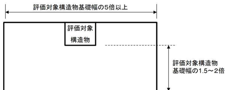
図 3-3 モデル化範囲の考え方
