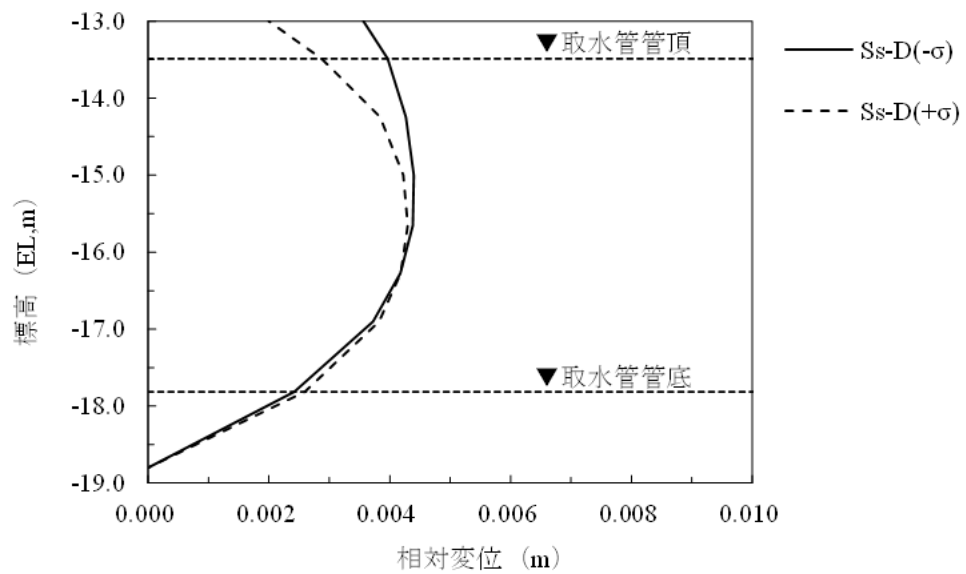
図 4-8 砕石の最大応答変位分布図（面外加振）（解析ケース②，③）
