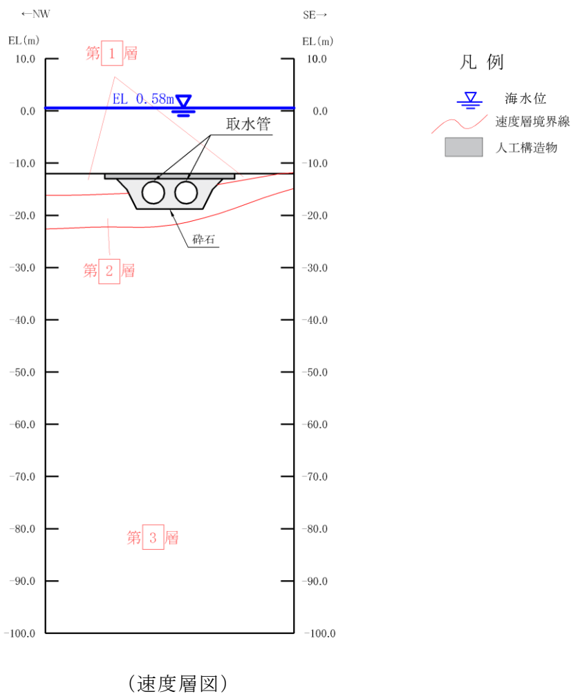
図 2-8 取水管 地質断面図 (C-C 断面)
