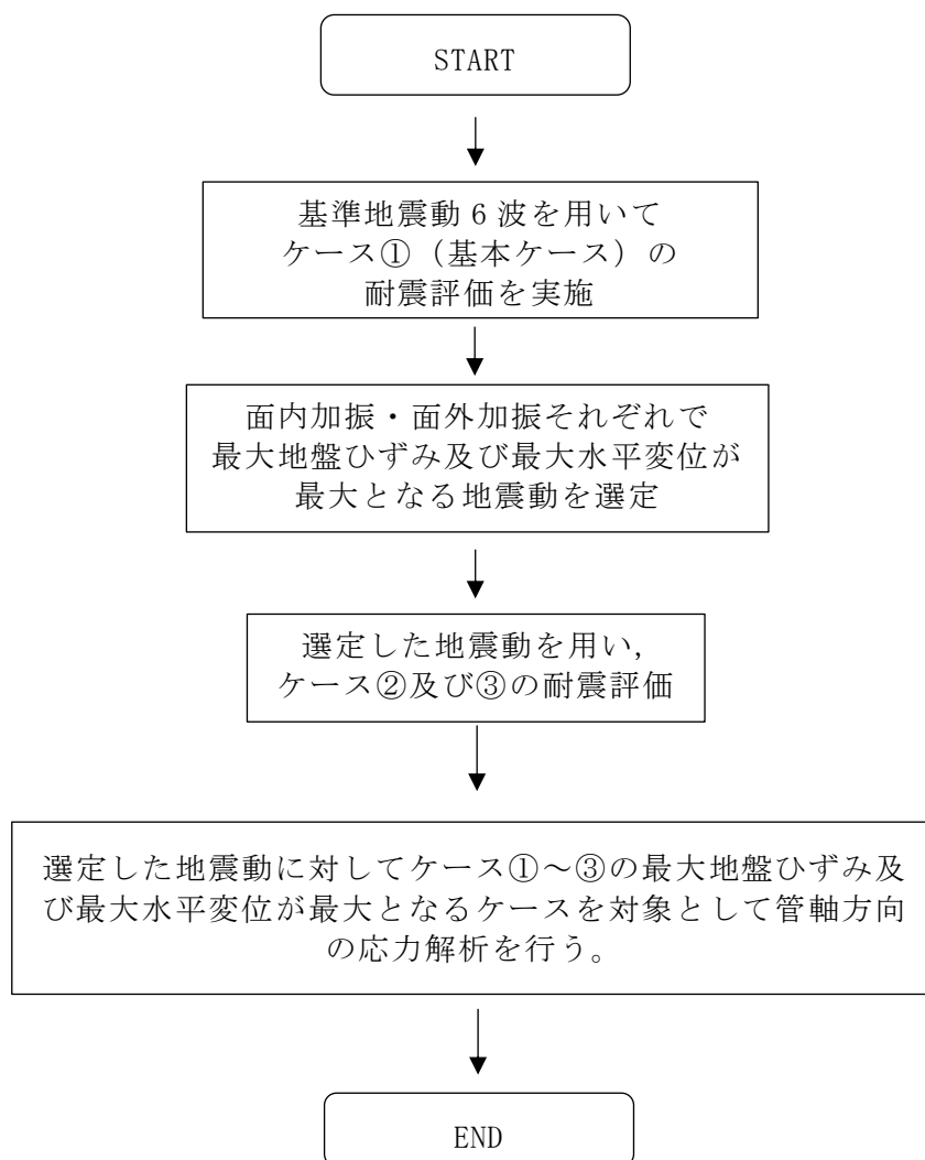
図 4-2 追加解析を実施する地震動の選定フロー
