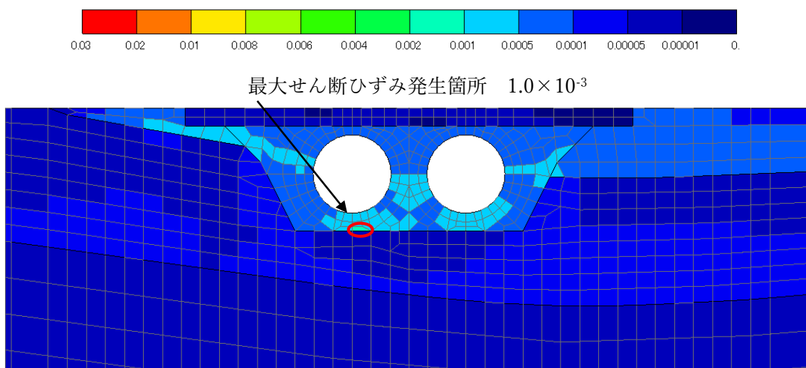
図 3-48 基礎地盤の最大せん断ひずみ分布図 (8/12) (解析ケース①, S_s - N 1 (- +) )
