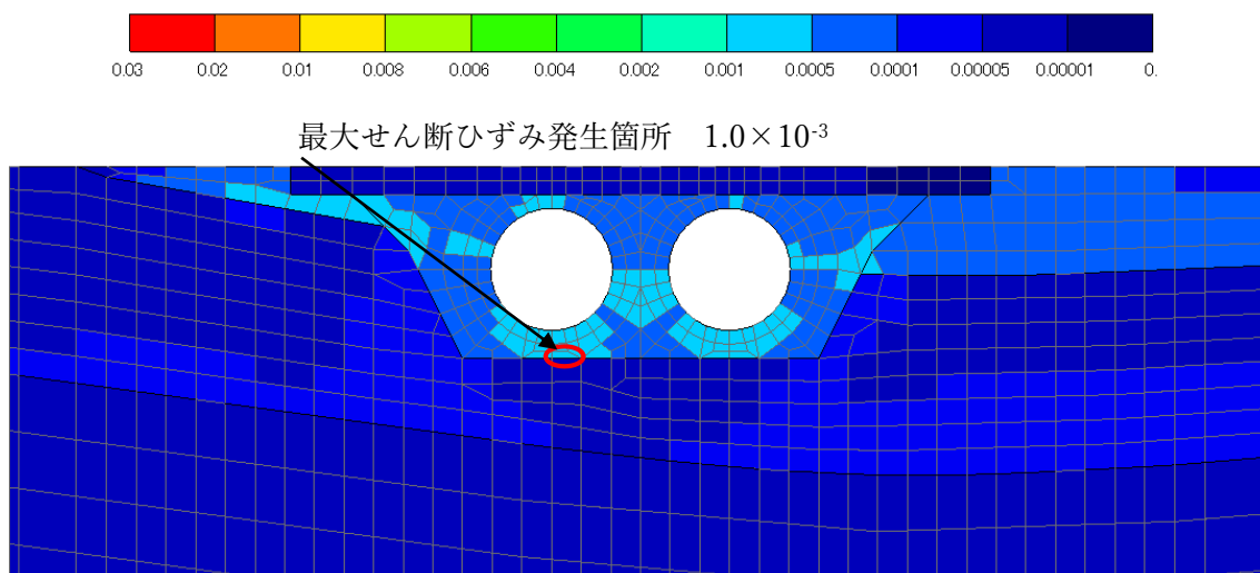
図 3-50 基礎地盤の最大せん断ひずみ分布図 (10/12) (解析ケース①, S_s - N_2 (NS) (- +) )
