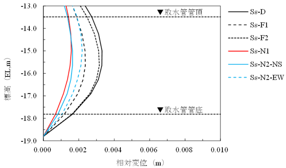
図 4-5 砕石の最大応答変位分布図（面内加振）（解析ケース①）
