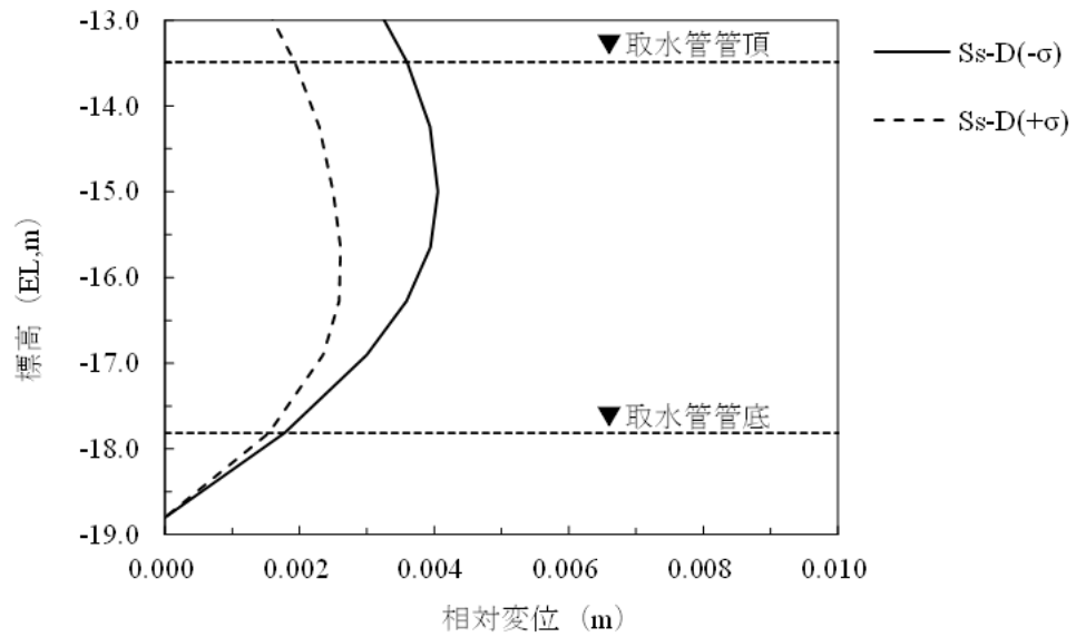
図 4-7 砕石の最大応答変位分布図（面内加振）（解析ケース②，③）
