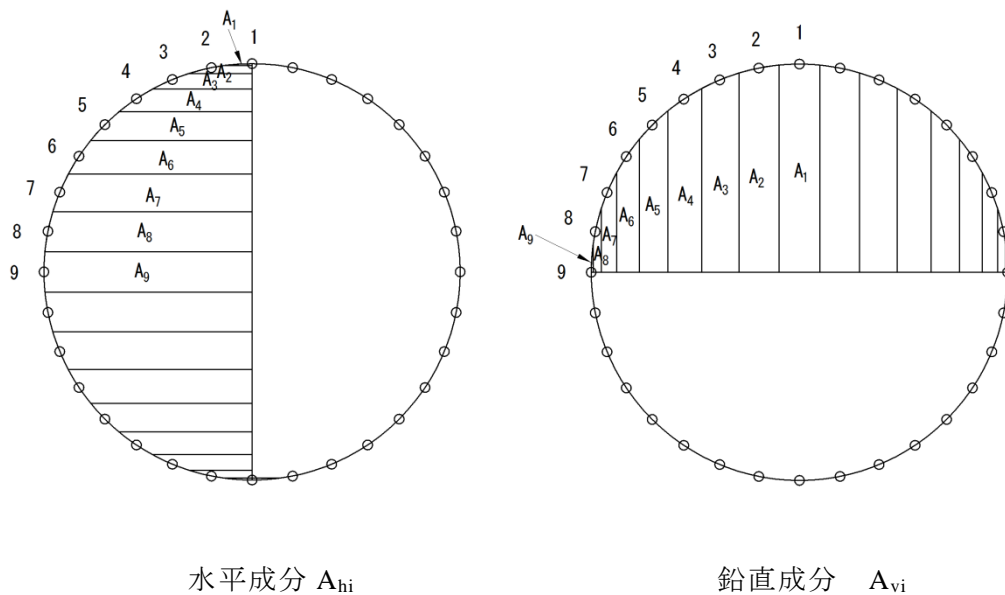
図3-14 動水圧の概念図
