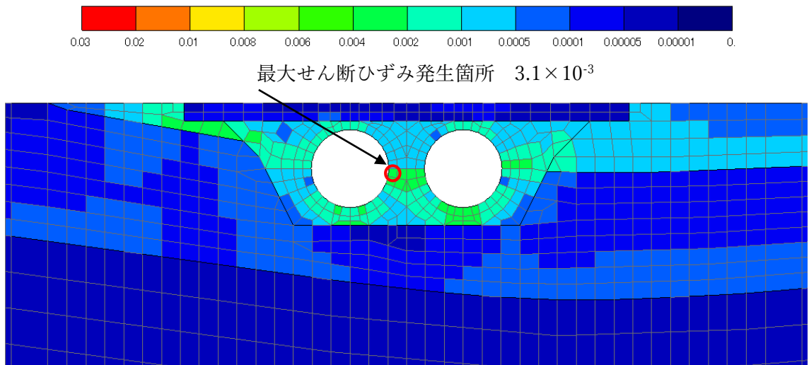
図 3-56 基礎地盤の最大せん断ひずみ分布図 (2/2) (解析ケース③, S_s - F_2 (++) )
