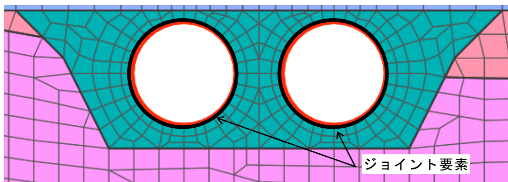
図 3-9 ジョイント要素設置箇所断面図
