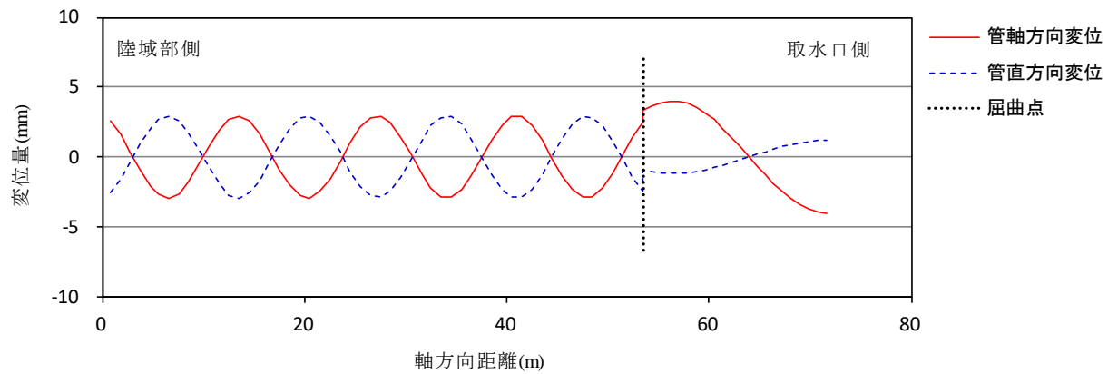
図 5-6 入力地盤変位（入射角 45°）
