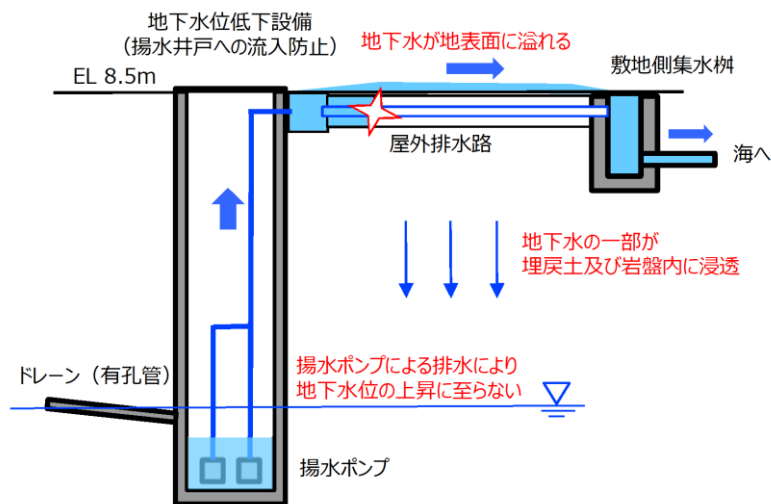
図3-1 地下に浸透した地下水の流れのイメージ
