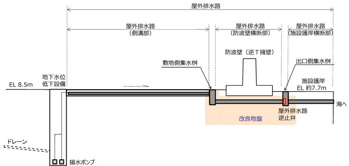
図 2-2 屋外排水路の縦断イメージ
