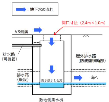
図 2-1 敷地側集水樹（開口寸法）
