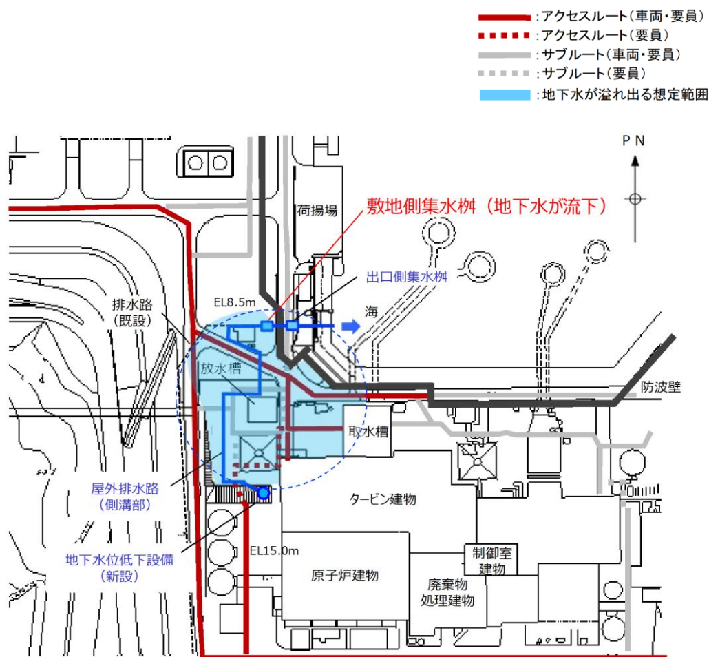
図 2-4 屋外排水路（側溝部）周辺のアクセスルート平面図
