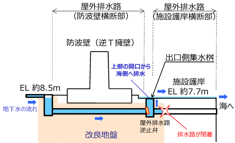
図 3-4 地震時における出口側集水桝の排水イメージ
