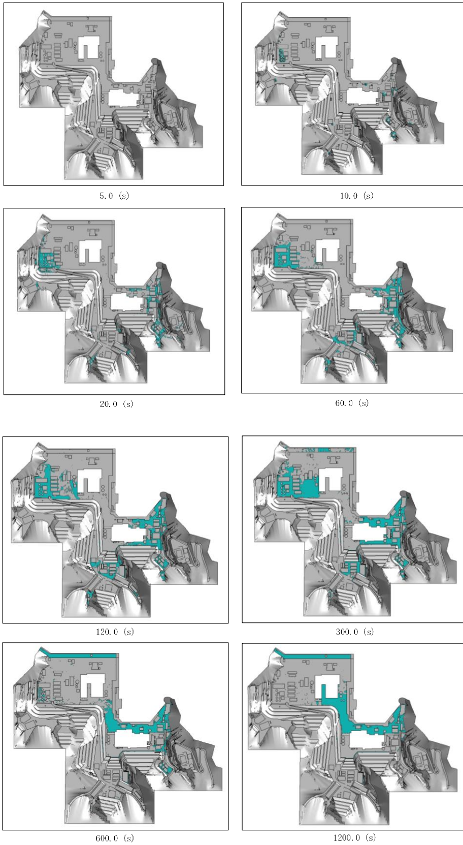
図 2-3 屋外タンク等の溢水伝播挙動
