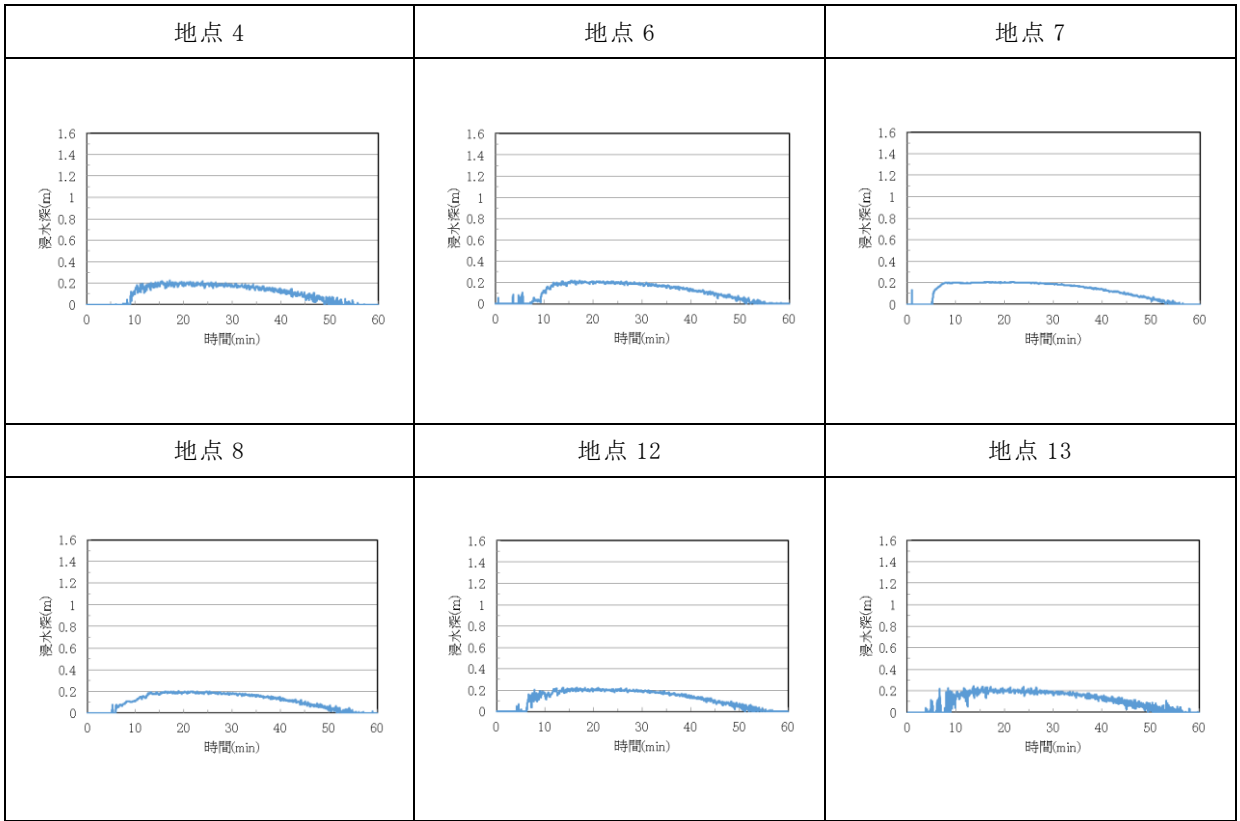
図 2-2 屋外排水路（側溝部）周辺の浸水深時刻歴
