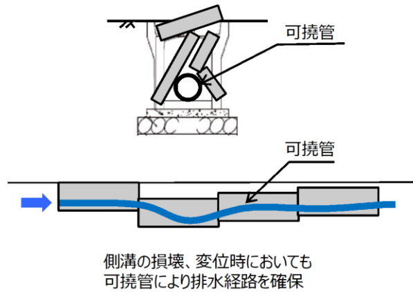
図 3-1 可撓管による排水イメージ
