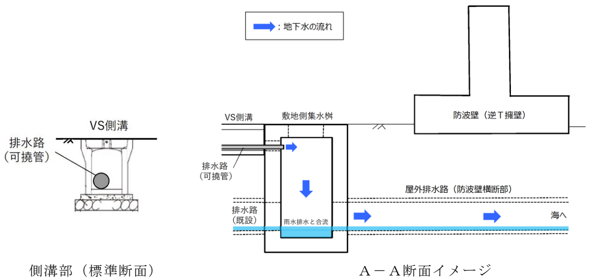
図 2-1 地下水の排水経路
