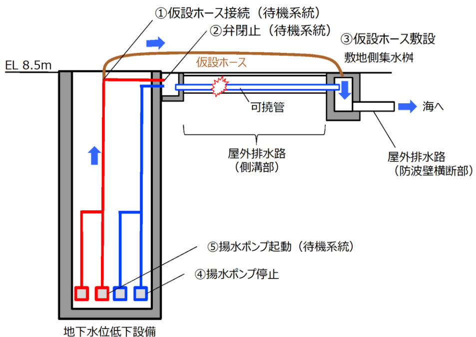
図 3-3 仮設ホース接続の概要
