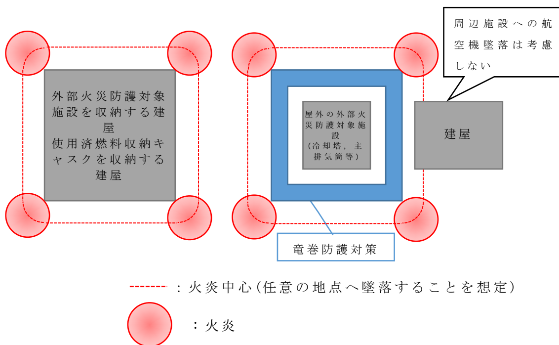
第 3.1-1 図 設計上想定する航空機の墜落地点のイメージ(平面図)
