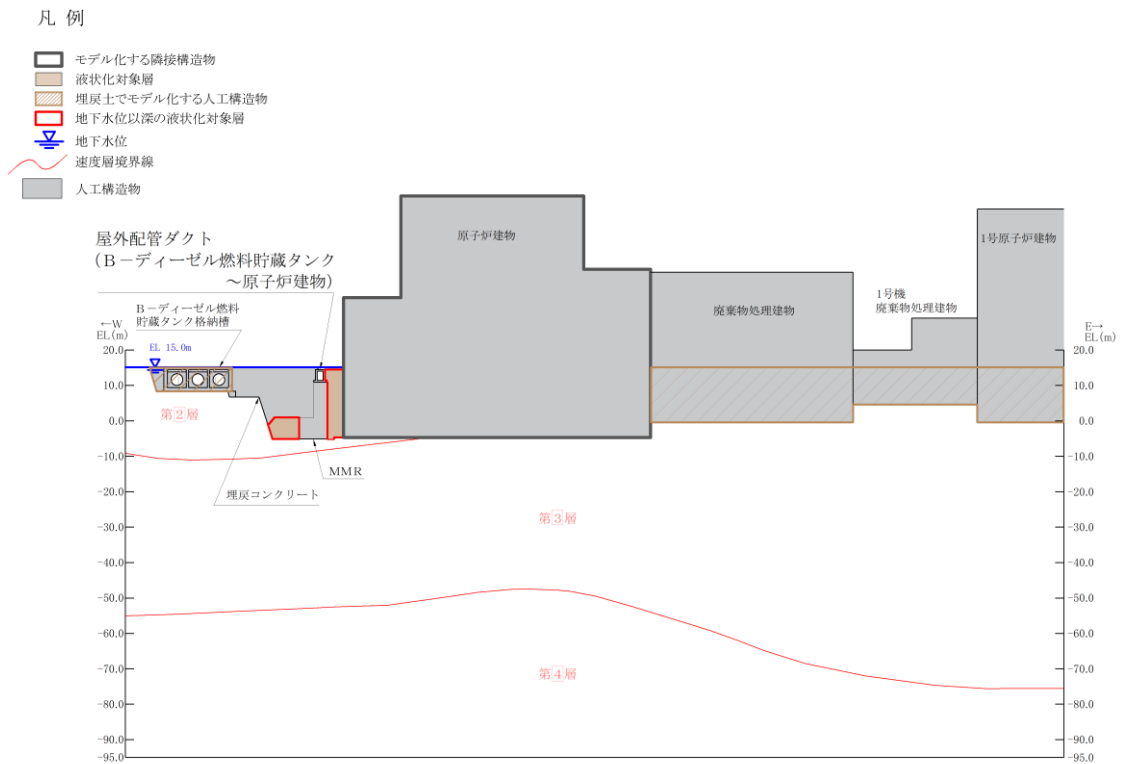
図 8.2-3(15) 埋戻土（非液状化）としてモデル化する場合の例
