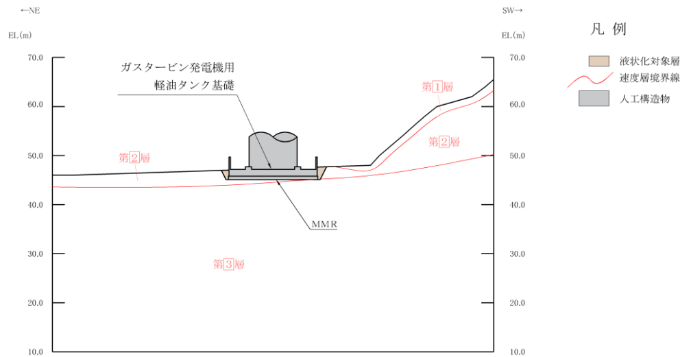
(速度層図)
