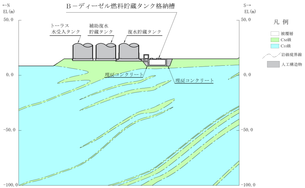
(岩級図)
