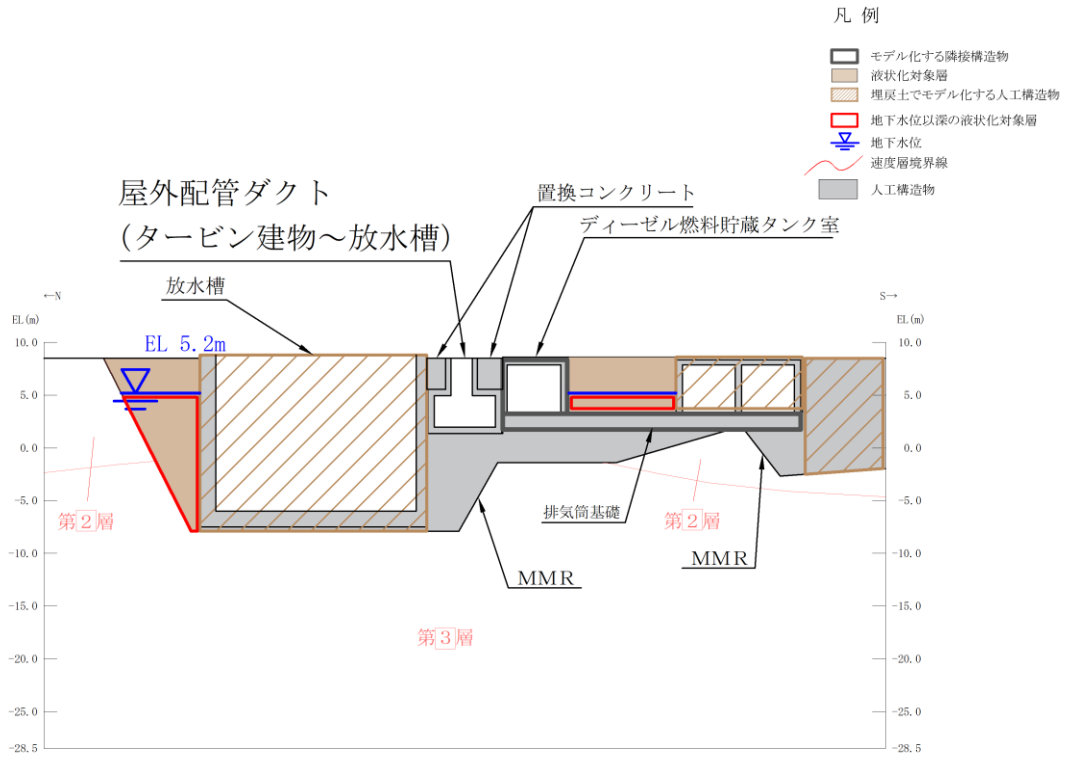
図 8.2-3(3) 隣接構造物としてモデル化する場合の例 (a) 排気筒基礎及びディーゼル燃料貯蔵タンク室：屋外配管ダクト (タービン建物～放水槽) 【B-B断面】
