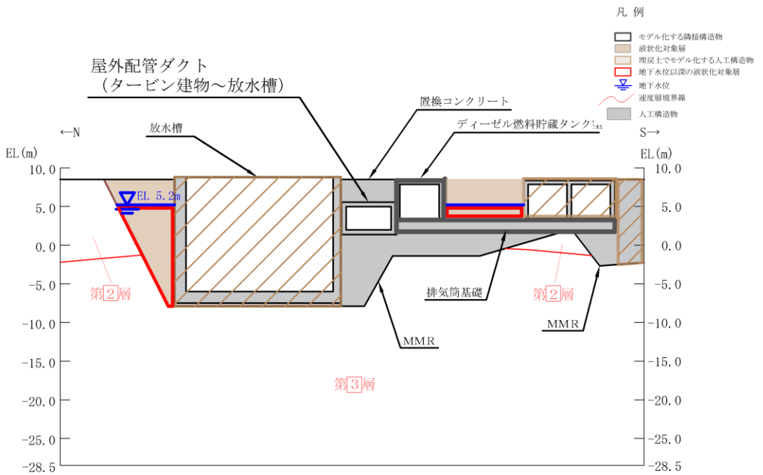
図 8.2-3(16) 耐震性を有さない構造物を埋戻土としてモデル化する場合の例 (e) 放水槽：屋外配管ダクト (タービン建物～放水槽) 【A-A 断面】
