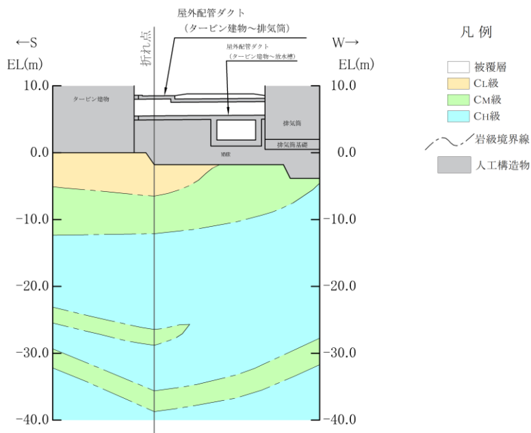
(岩級図)
