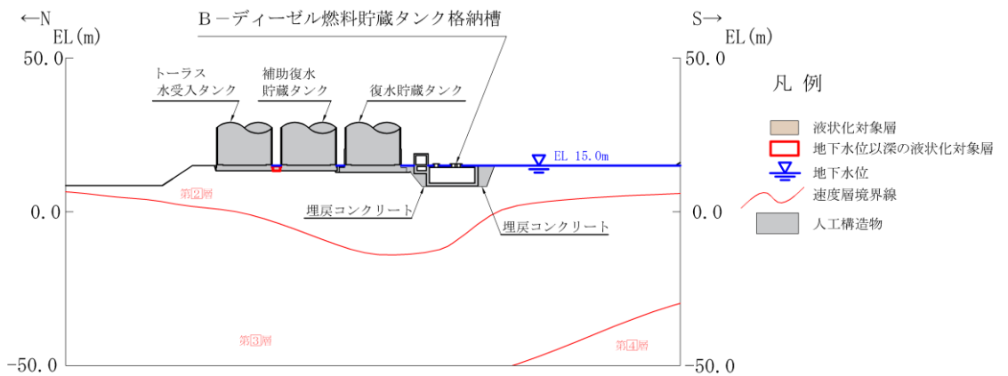
図 4.3-2(10) B-ディーゼル燃料貯蔵タンク格納槽【B-B断面】地質断面図 (②全応力解析)
