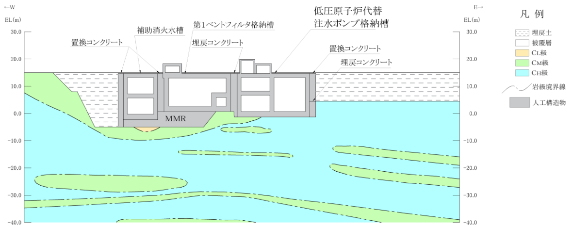
(岩級図)
