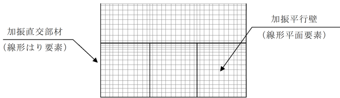
図 11.2-5 構造部材のモデル化 (B-B断面の例)
