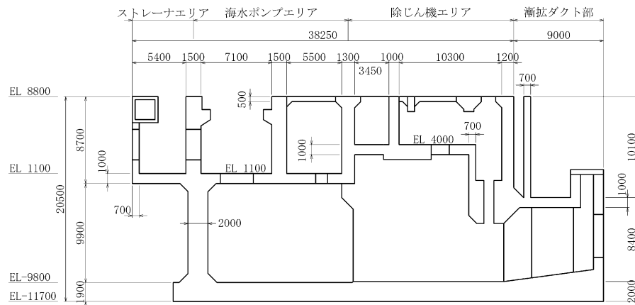
図 1-2 取水槽 縦断図
