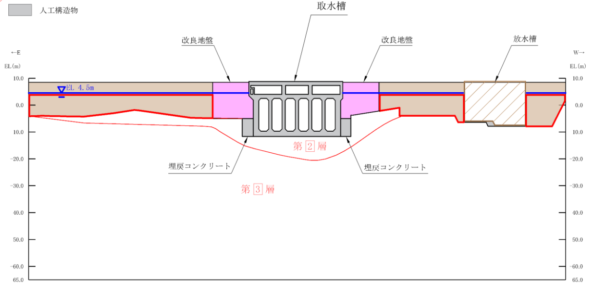
図 4.3-2(21) 取水槽【A-A断面】 地質断面図 (⑤有効応力解析)
