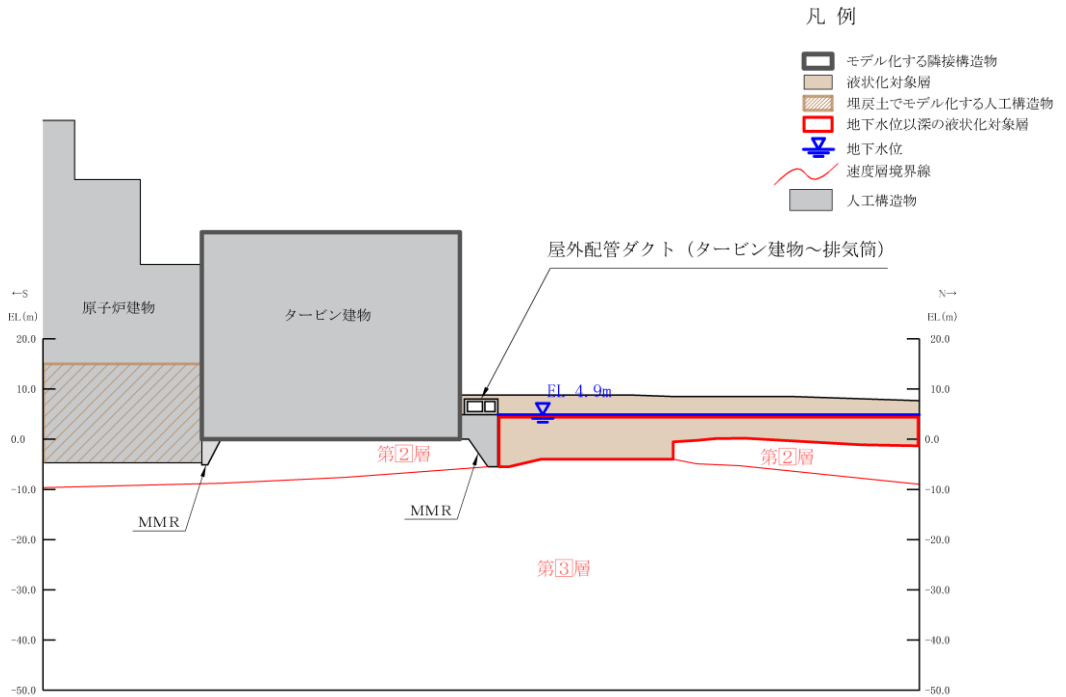
図 8.2-3(4) 隣接構造物としてモデル化する場合の例 (b) タービン建物：屋外配管ダクト (タービン建物～排気筒) 【A-A断面】
