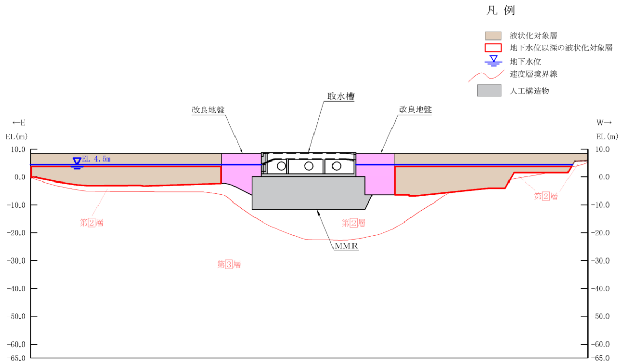
(速度層図)
