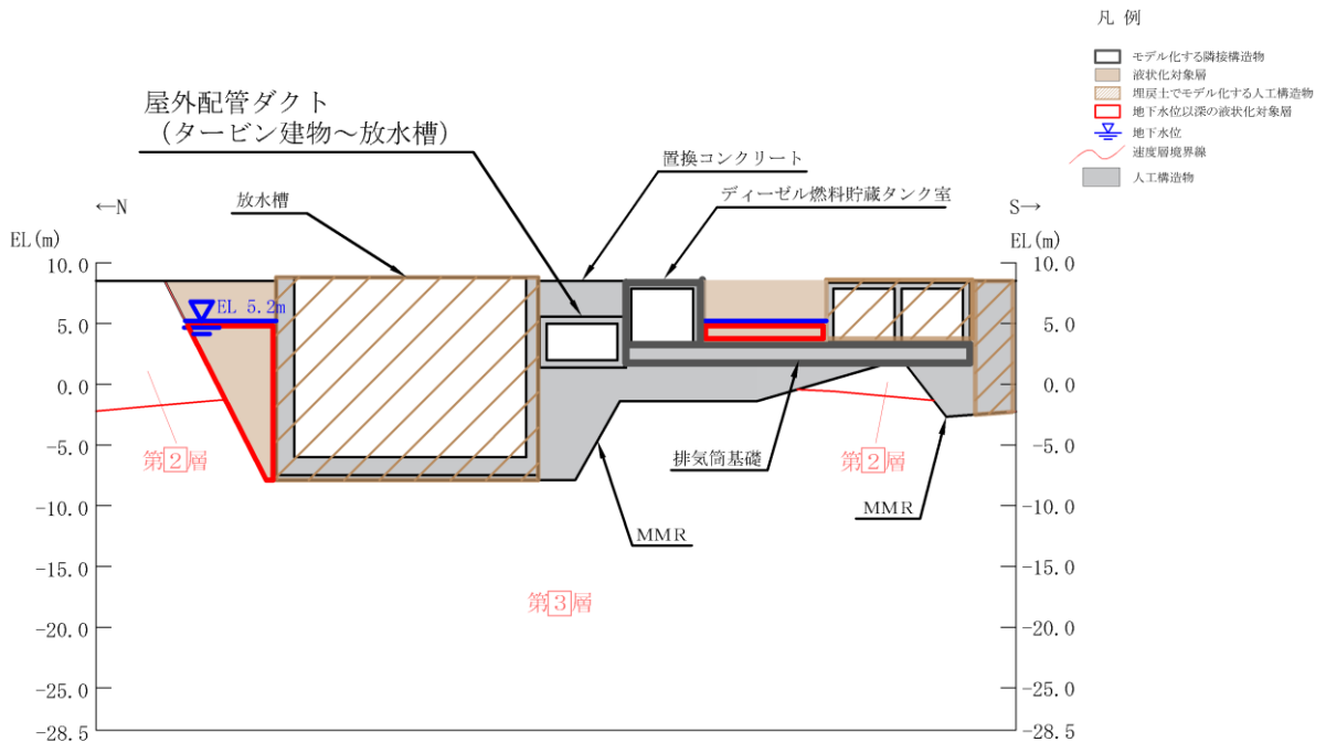
図 8.2-3(2) 隣接構造物としてモデル化する場合の例
