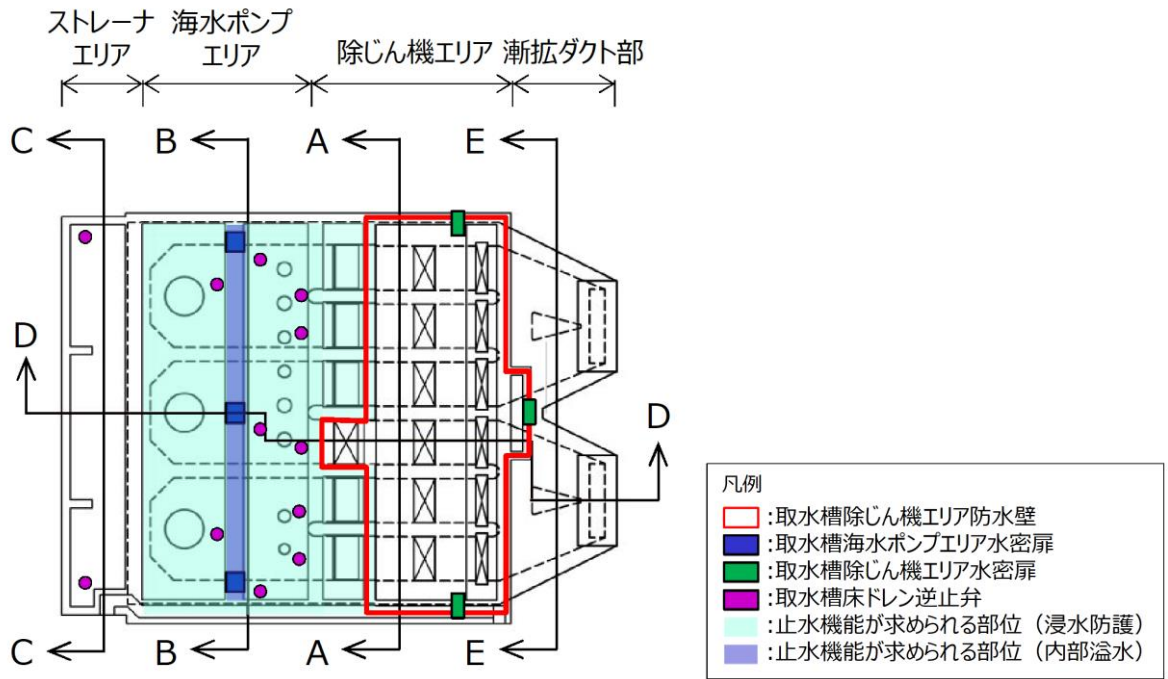
平面図
