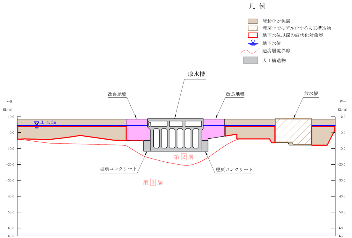
(速度層図)
