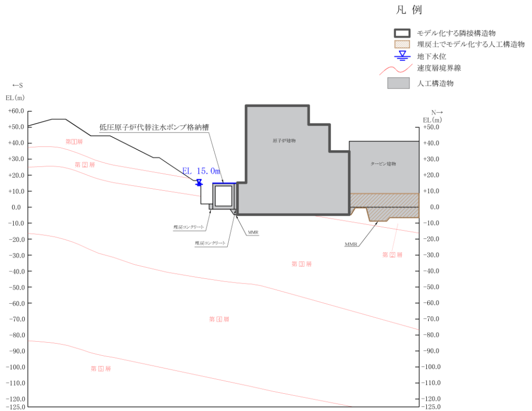
図 8.2-3(10) 隣接構造物としてモデル化する場合の例 (c) 原子炉建物：低圧原子炉代替注水ポンプ格納槽【B-B断面】
