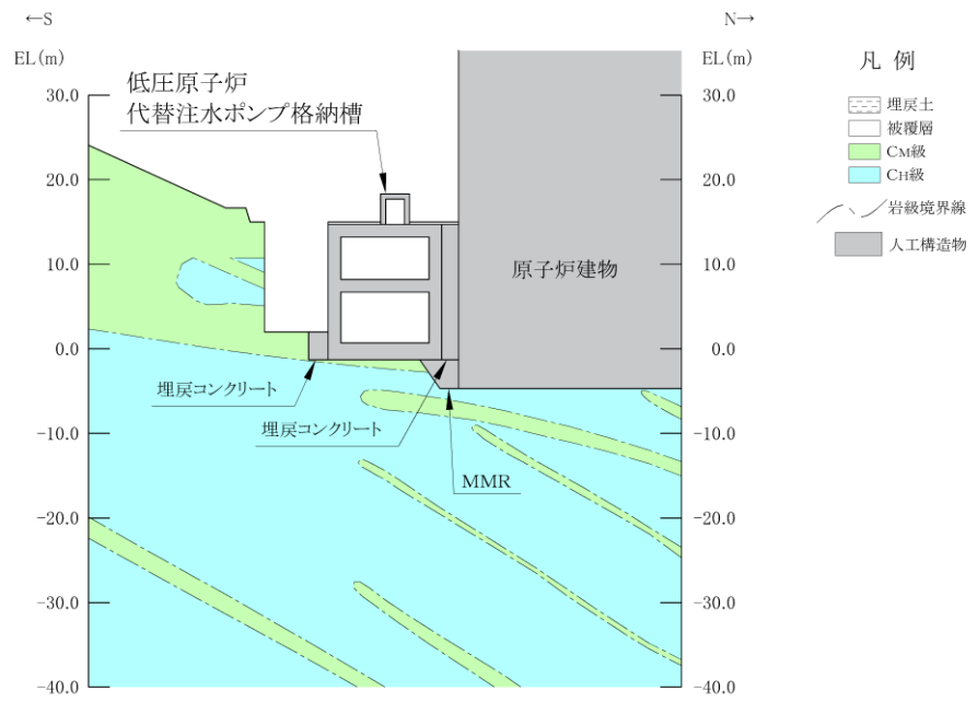
(岩級図)
