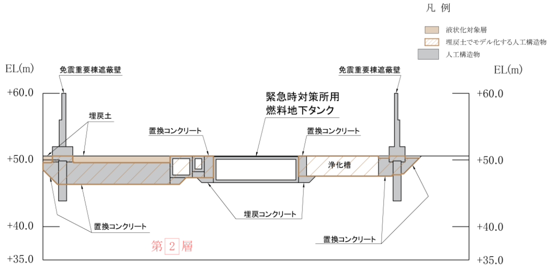
図 8.2-3(18) 耐震性を有さない構造物を埋戻土としてモデル化する場合の例
