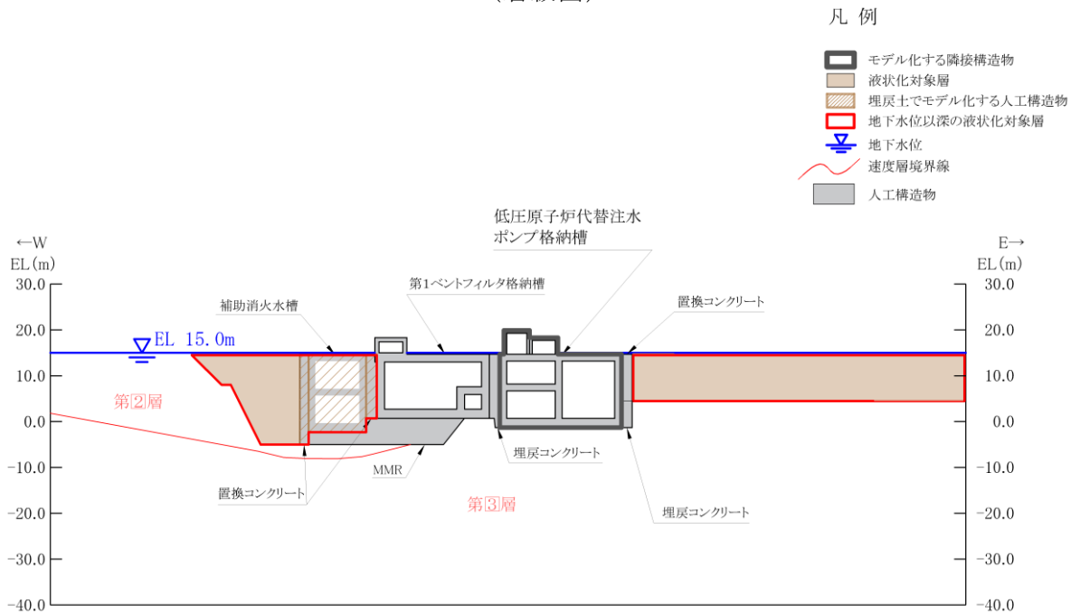
(速度層図)
