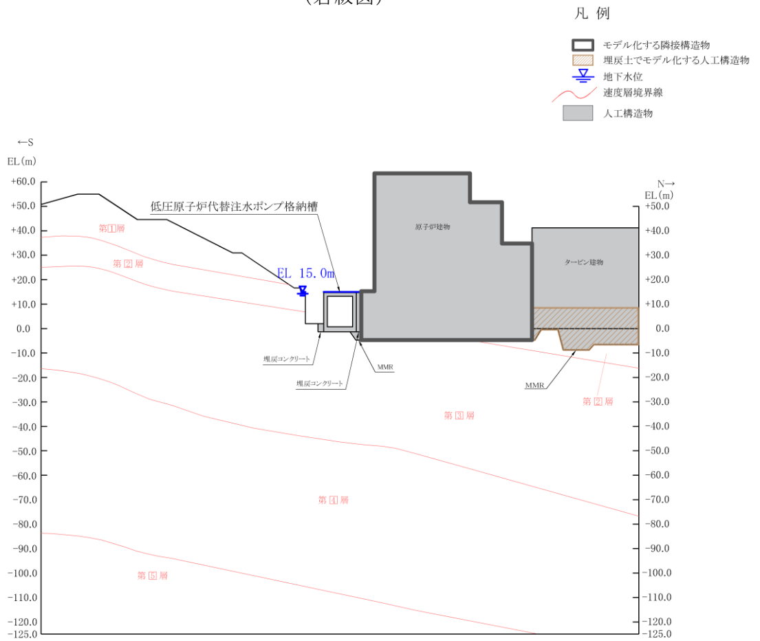
(速度層図)
