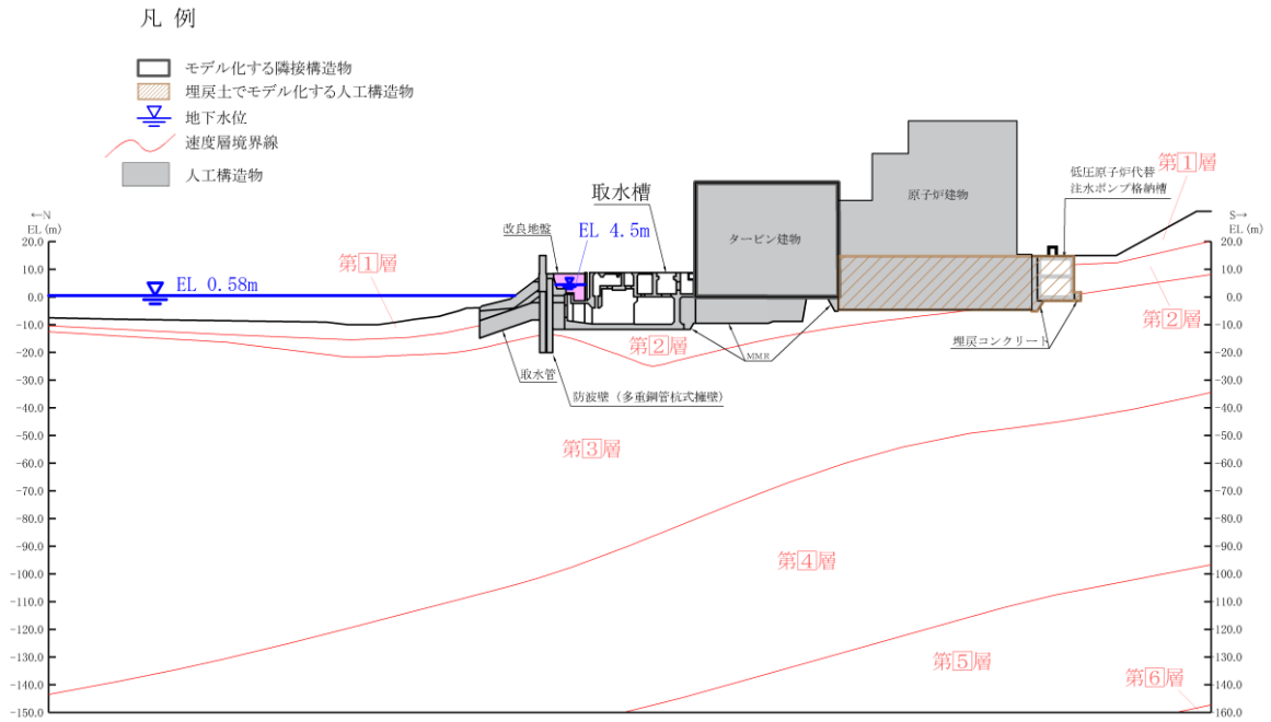
図 8.2-3(1) 隣接構造物としてモデル化する場合の例
