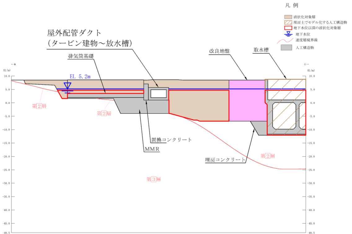
図 8.2-3(13) 埋戻土（非液状化）としてモデル化する場合の例
