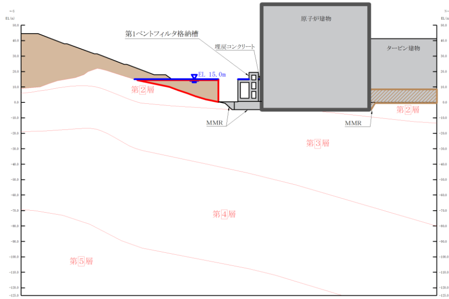
図 4.3-2(13) 第1ベントフィルタ格納槽 地質断面図 【A-A断面】 (②全応力解析)
