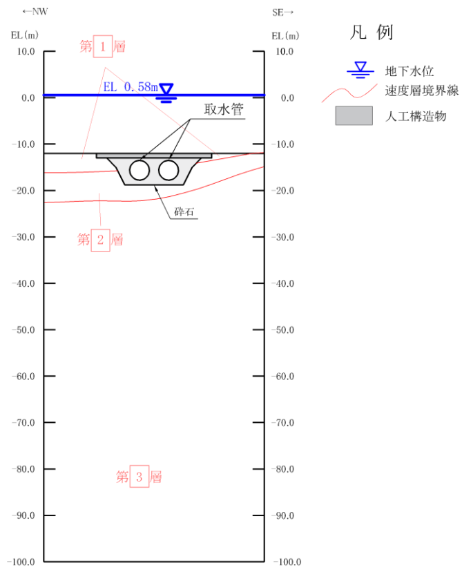
図 4.3-2(9) 取水管【C-C断面】地質断面図 (②全応力解析)
