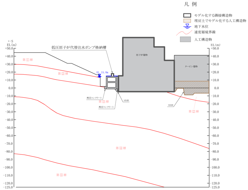
図 8.2-3(9) 隣接構造物としてモデル化する場合の例 (c) 原子炉建物：低圧原子炉代替注水ポンプ格納槽【A-A断面】
