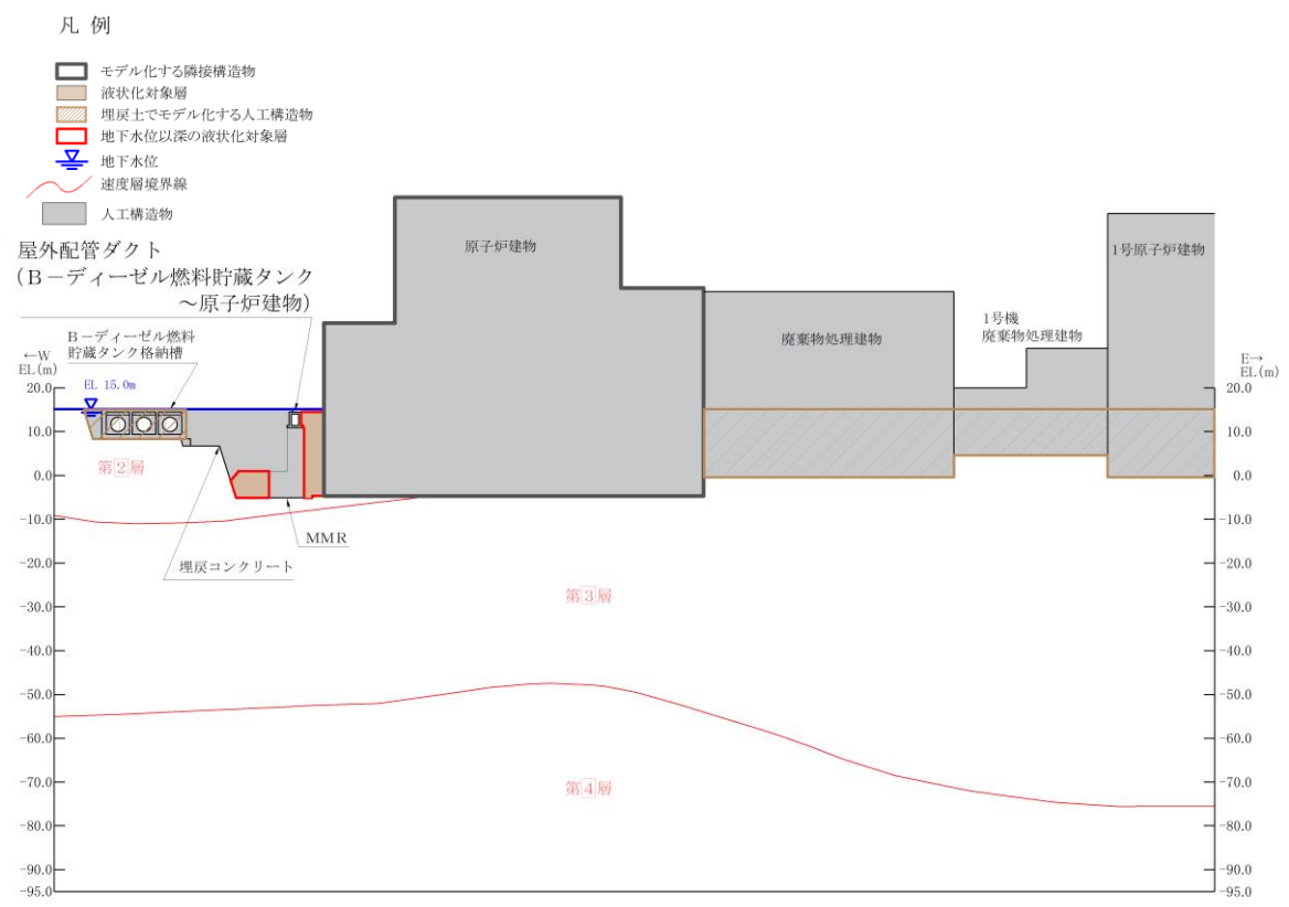
(速度層図)
