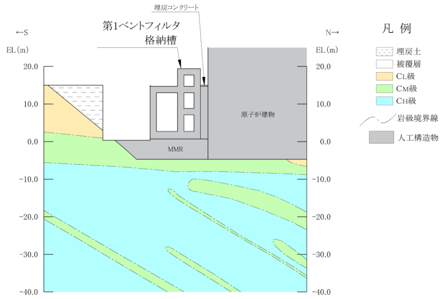
(岩級図)
