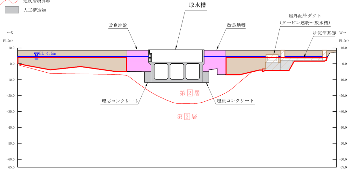
図 4.3-2(22) 取水槽【B-B断面】 地質断面図 (⑤有効応力解析)
