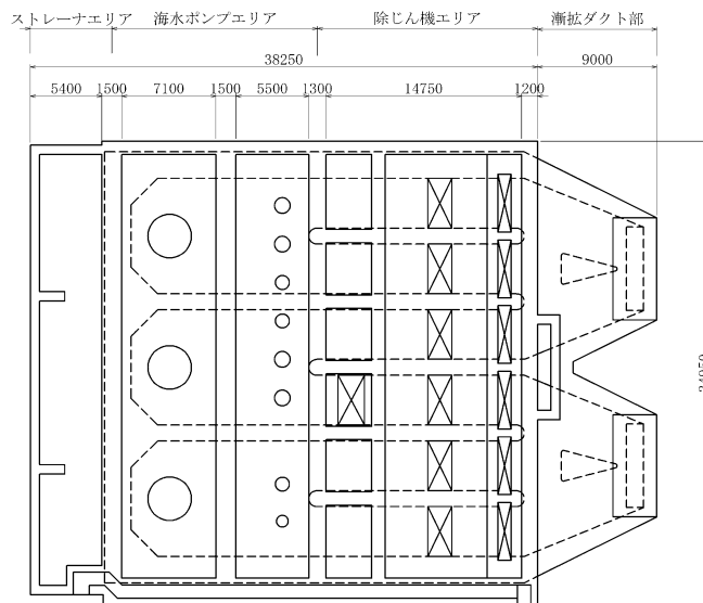
図 1-1 取水槽 平面図
