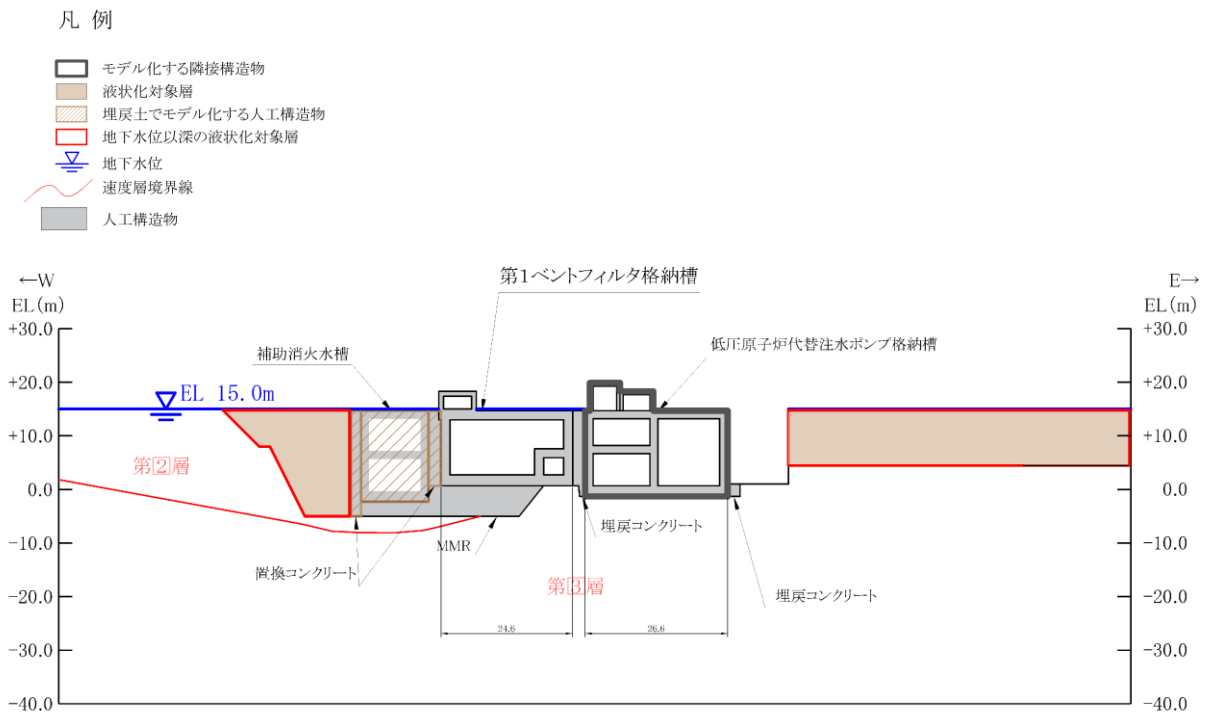
図 8.2-3(19) 耐震性を有さない構造物を埋戻土としてモデル化する場合の例
