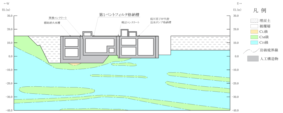
(岩級図)
