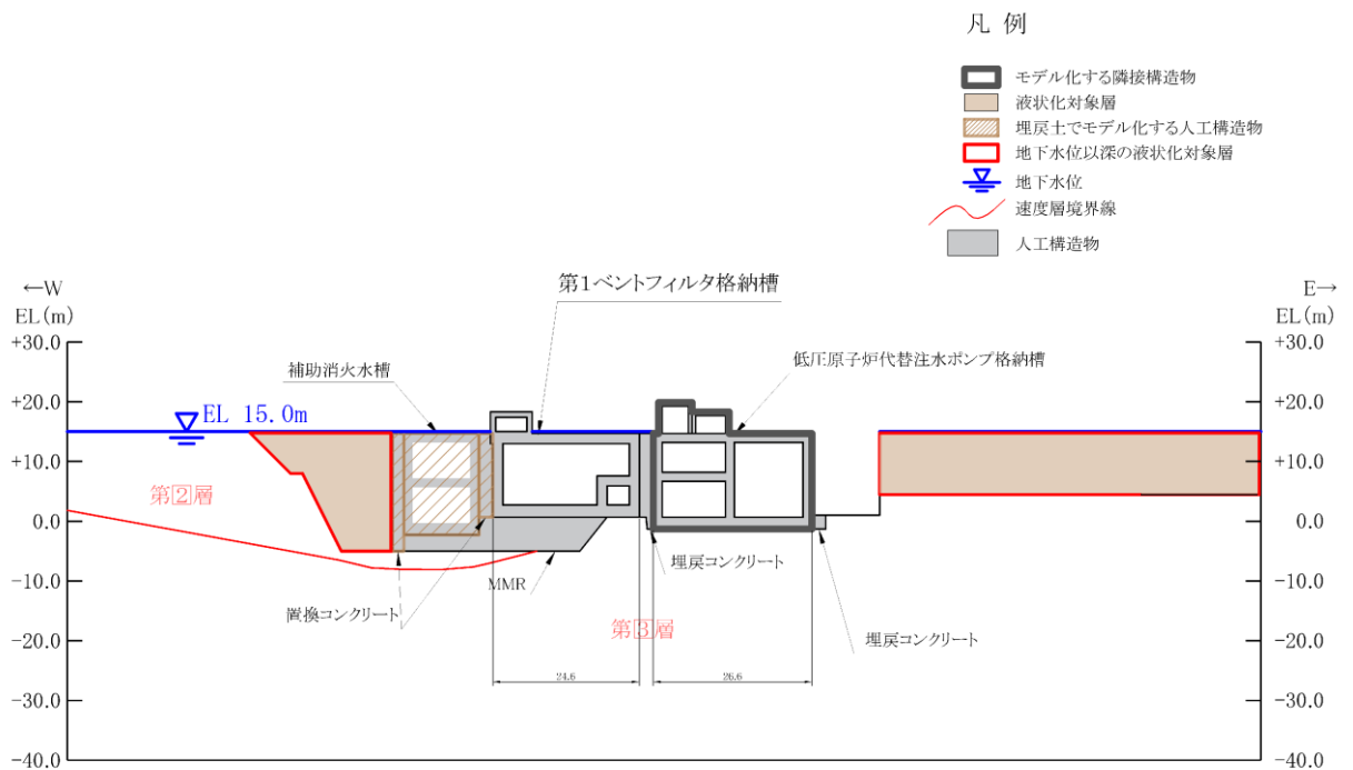
図 8.2-3(8) 隣接構造物としてモデル化する場合の例 (c) 低圧原子炉代替注水ポンプ格納槽：第1ベントフィルタ格納槽【C-C断面】
