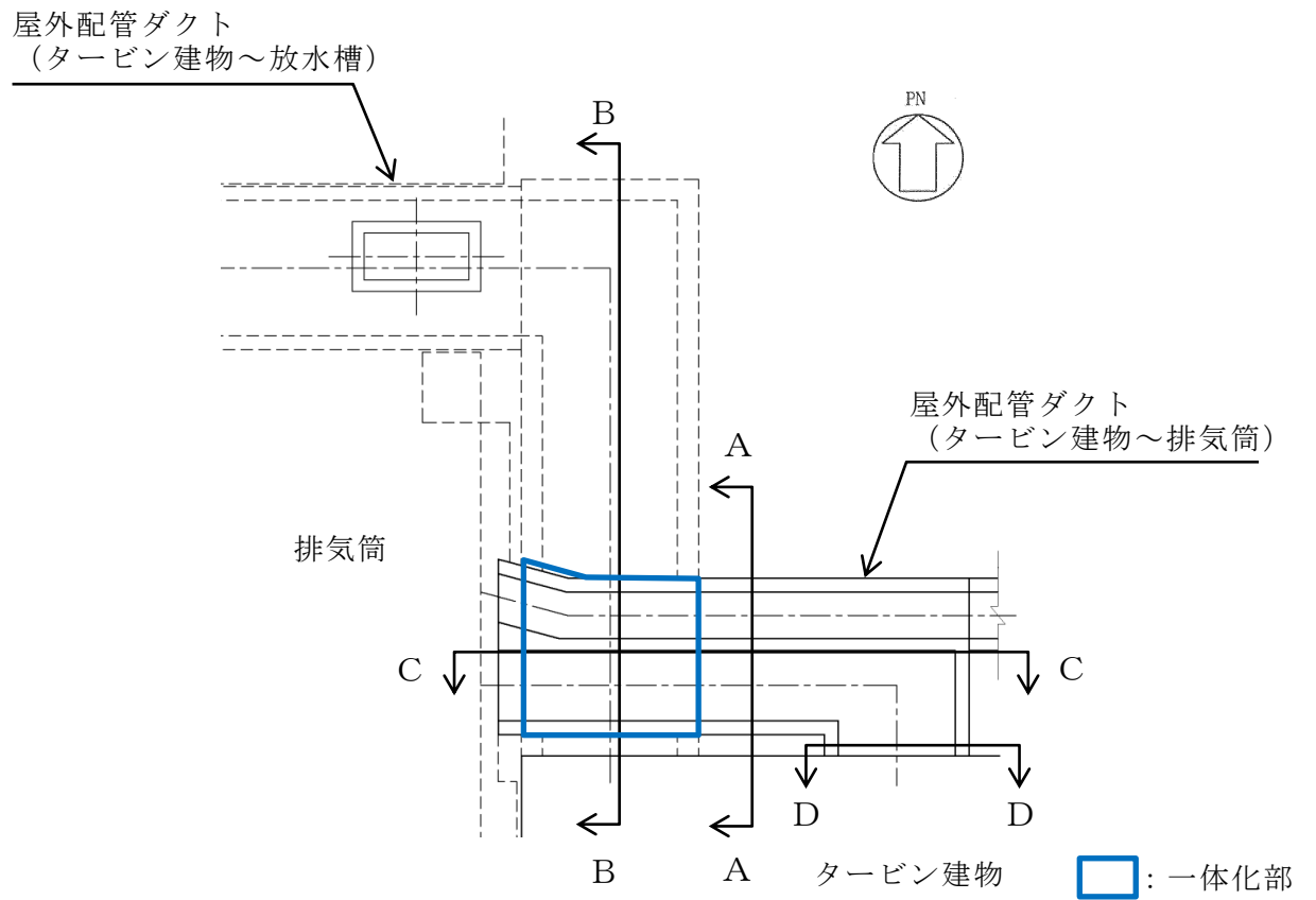
図 4.5-2 屋外配管ダクト (タービン建物～排気筒) 平面図
