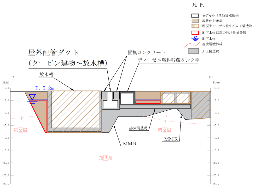
図 8.2-3(17) 耐震性を有さない構造物を埋戻土としてモデル化する場合の例 (e) 放水槽：屋外配管ダクト (タービン建物～放水槽) 【B-B 断面】
