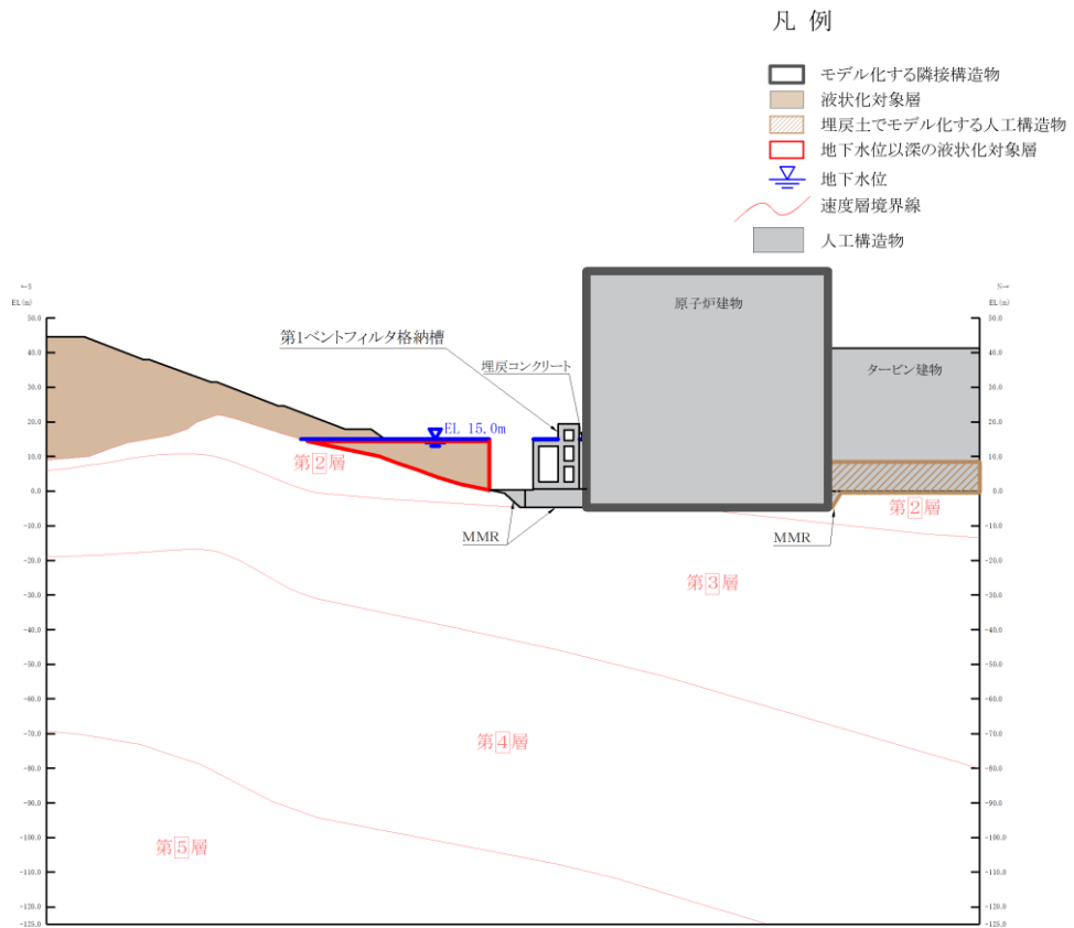
図 8.2-3(6) 隣接構造物としてモデル化する場合の例
