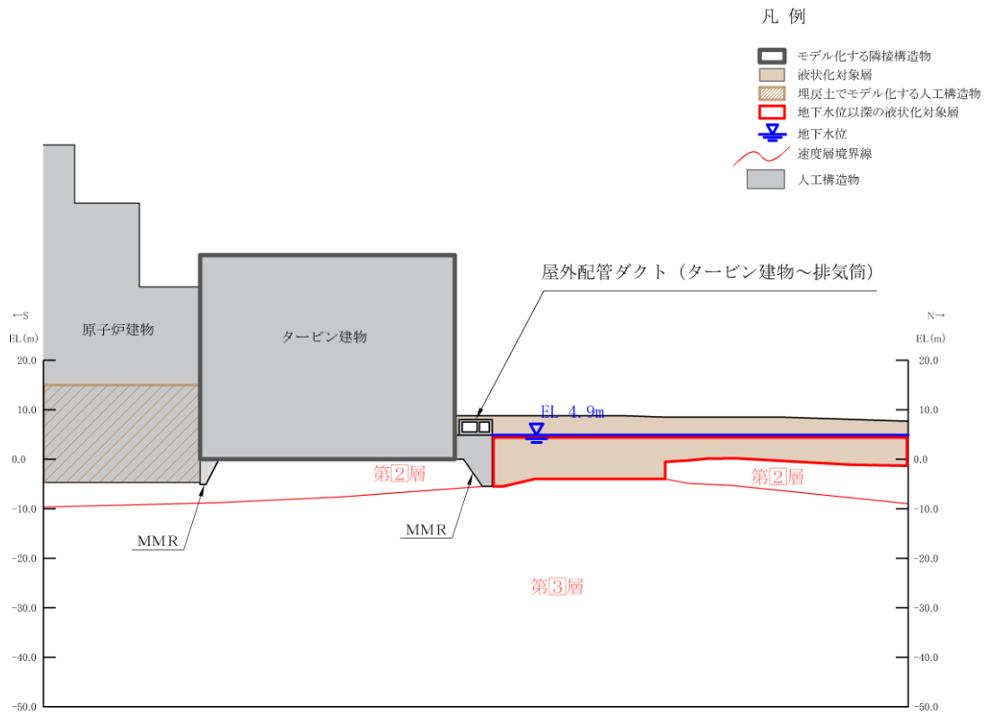
図 4.3-2(5) 屋外配管ダクト (タービン建物～排気筒) 【A-A断面】 地質断面図 (①全応力解析)
