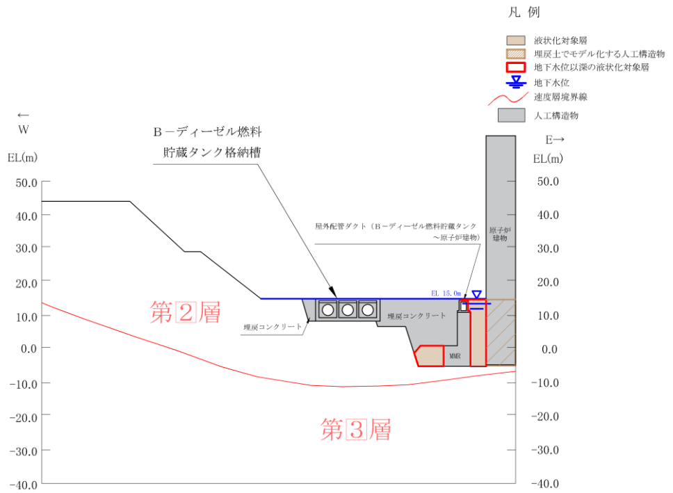
図 8.2-3(14) 埋戻土（非液状化）としてモデル化する場合の例
