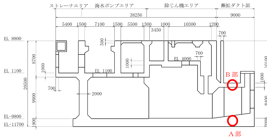
(i) 継手部付近の縦断図
