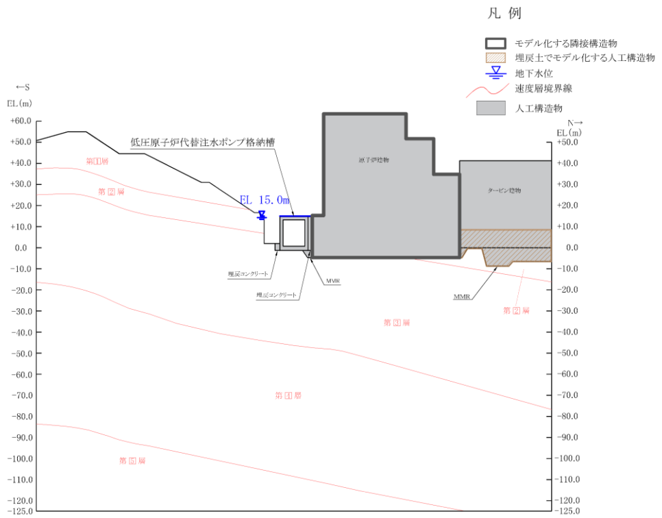
図 4.3-2(16) 低圧原子炉代替注水ポンプ格納槽【B-B断面】 地質断面図 (②全応力解析)
