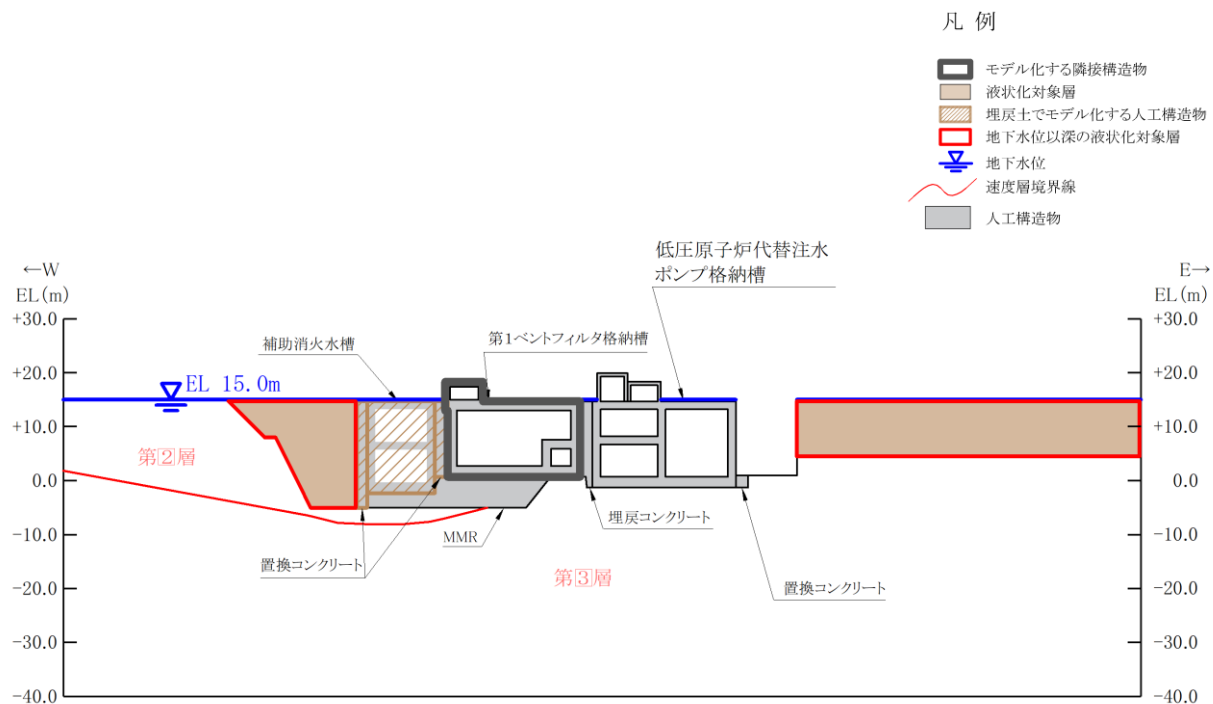
図 8.2-3(11) 隣接構造物としてモデル化する場合の例
