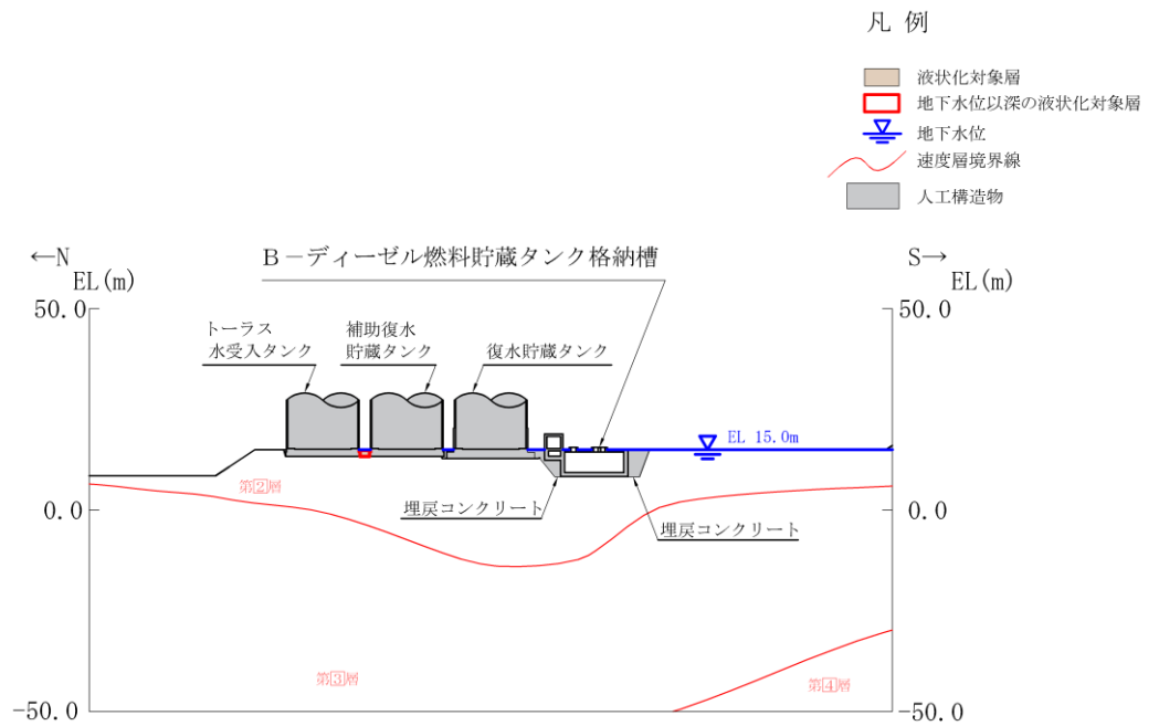
(速度層図)
