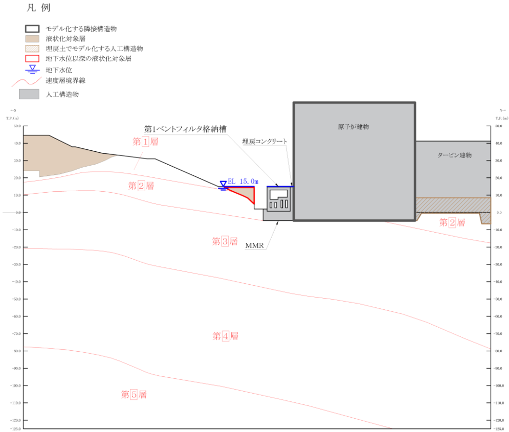
図 8.2-3(7) 隣接構造物としてモデル化する場合の例 (c) 原子炉建物：第1ベントフィルタ格納槽【B-B断面】
