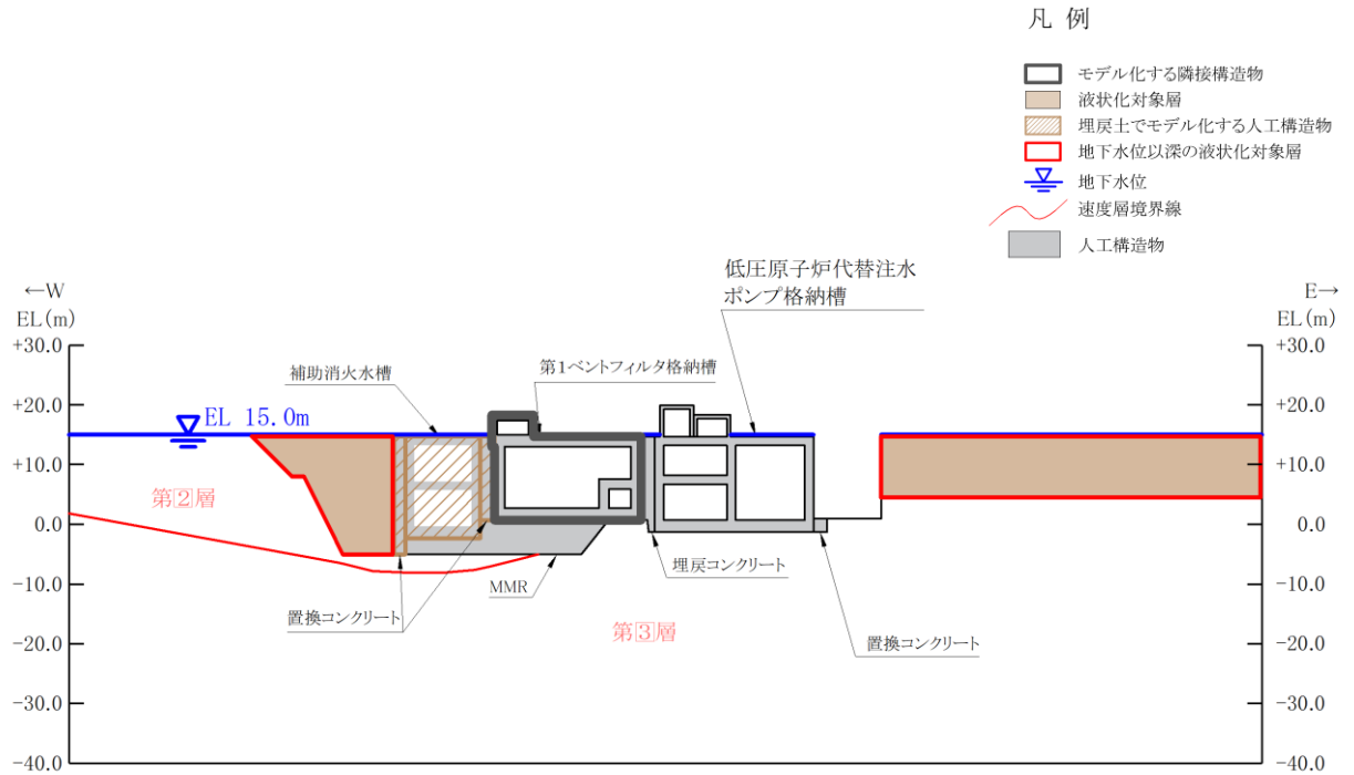
図 4.3-2(17) 低圧原子炉代替注水ポンプ格納槽【C-C断面】
