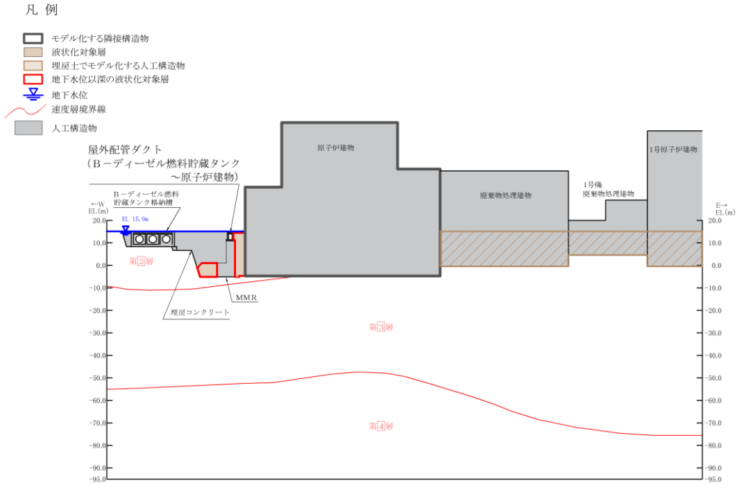
図 8.2-3(5) 隣接構造物としてモデル化する場合の例
