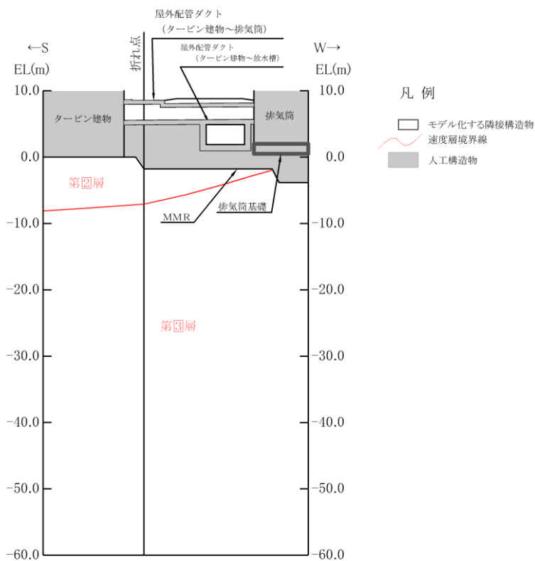
(速度層図)
