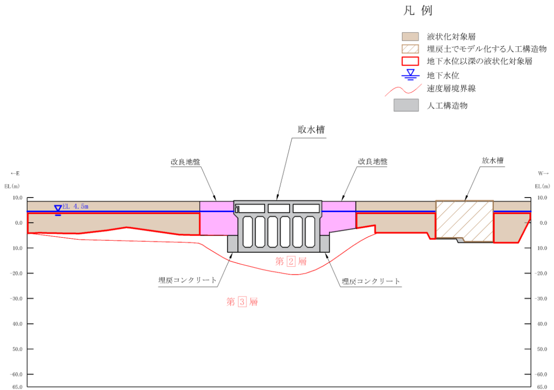
図 8.2-3(12) 埋戻土（非液状化）としてモデル化する場合の例
