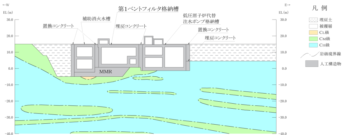
(岩級図)
