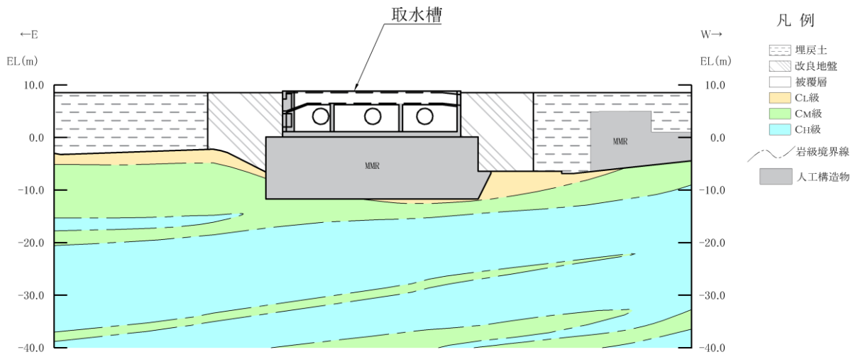
(岩級図)
