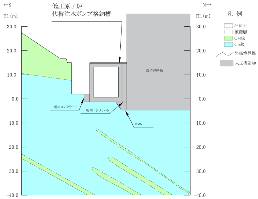
(岩級図)
