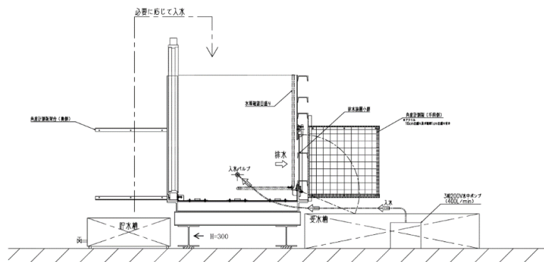
図 4-28 通水試験概要図
