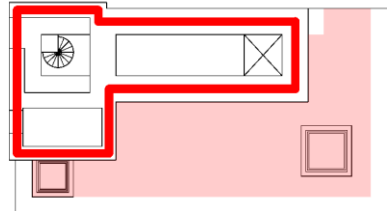
第1ベントフィルタ格納槽 EL 14700
