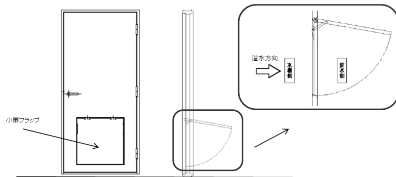
図4-25 通水扉の概要図
