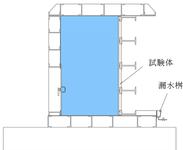
図4-7 溢水用防水壁の漏えい試験概要図
