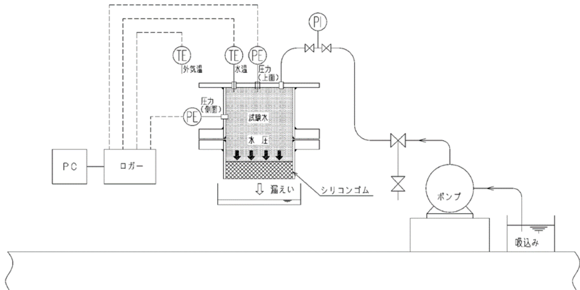
図4-11 漏えい試験概要図（シール材）
