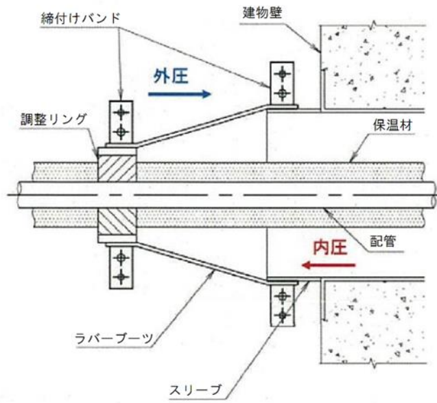
図 4-12 漏えい試験概要図 (ブーツ)
