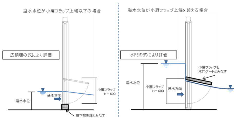
図 4-27 排水量評価式の適用状況
