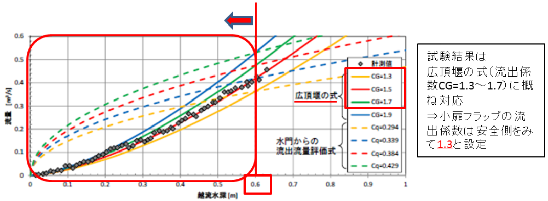
図 4-30 流出係数の設定 (広頂堰の式)
