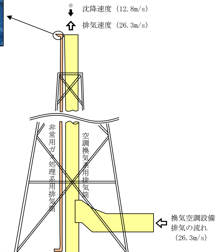
図1 排気筒（空調換気系用，非常用ガス処理系用）概要図
