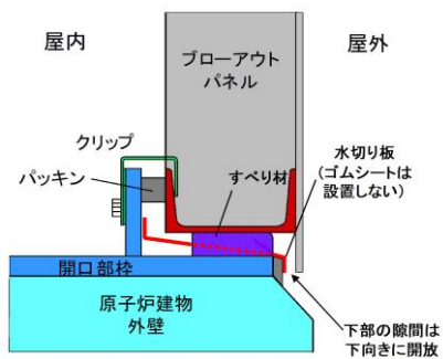
C-C 断面図 (通常時)
