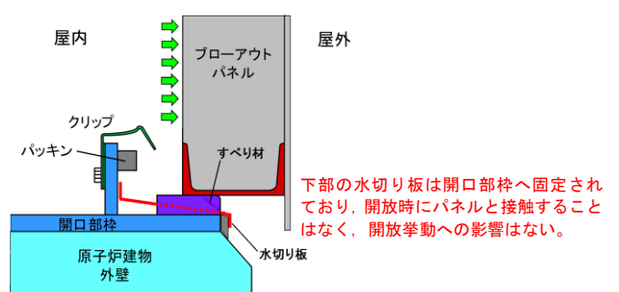
C-C 断面図 (開放動作時)
