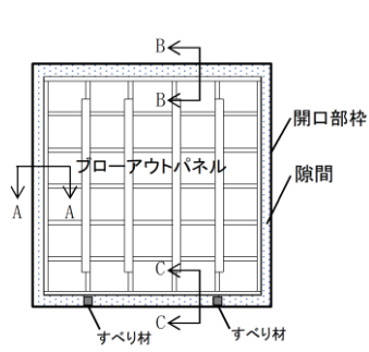
パネル見附図
