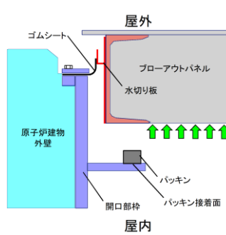
A-A 断面図 (開放動作時)
