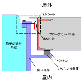
A-A 断面図 (通常時)
