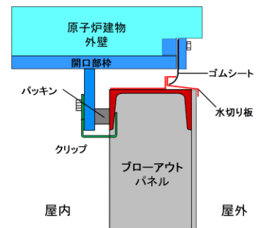
B-B 断面図 (通常時)
