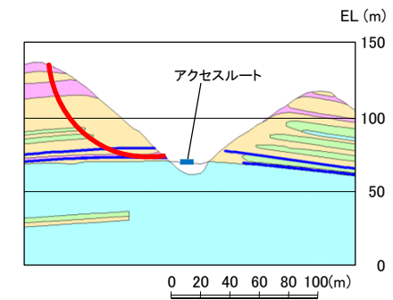
⑭-⑭' 断面
