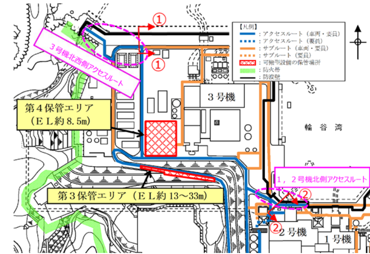
全体平面図
