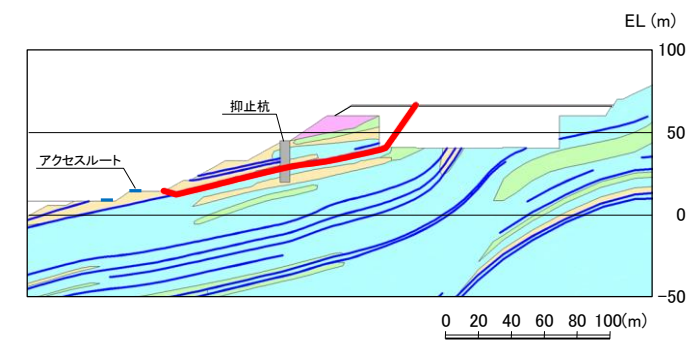
①-①' 断面
