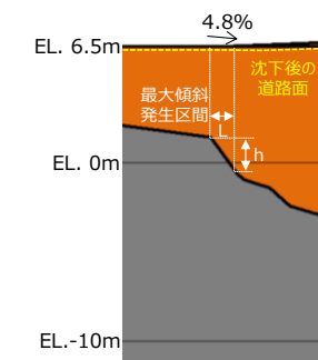
③-③断面
