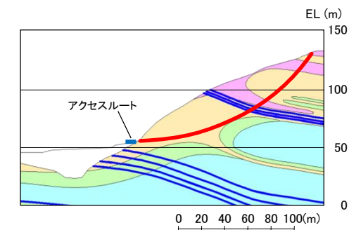
⑬-⑬' 断面
