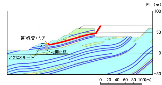
①-①' 断面
