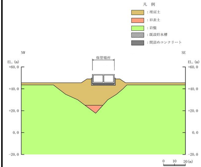
図 2-9 保管場所 (第 2 保管エリア) の地中埋没構造物 (輪谷貯水槽(西 1/西 2))
