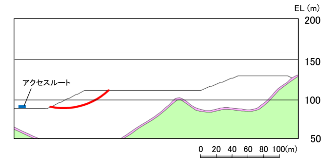
⑰-⑰' 断面
