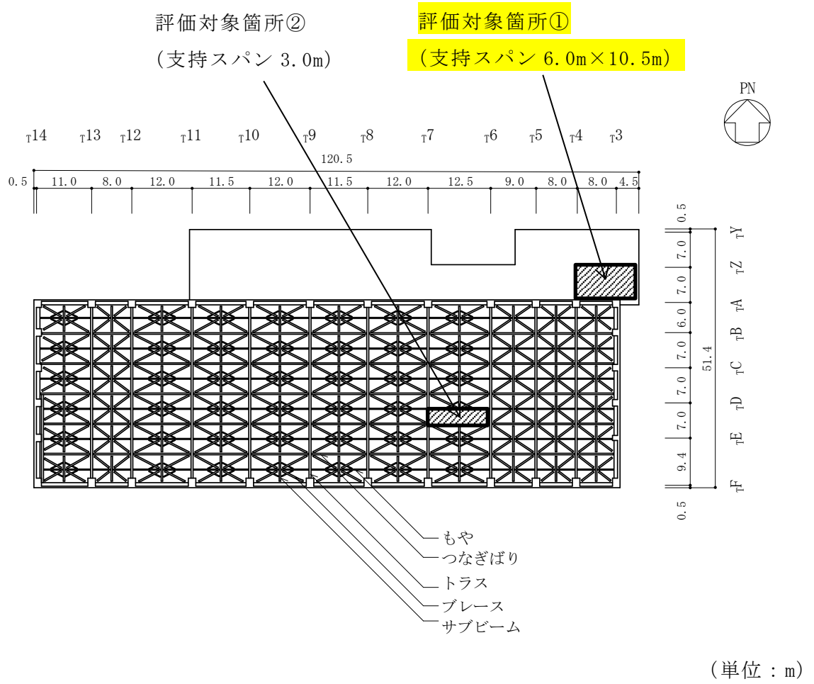
図 4-3 評価対象箇所 (屋根スラブ, EL 41.6m)
