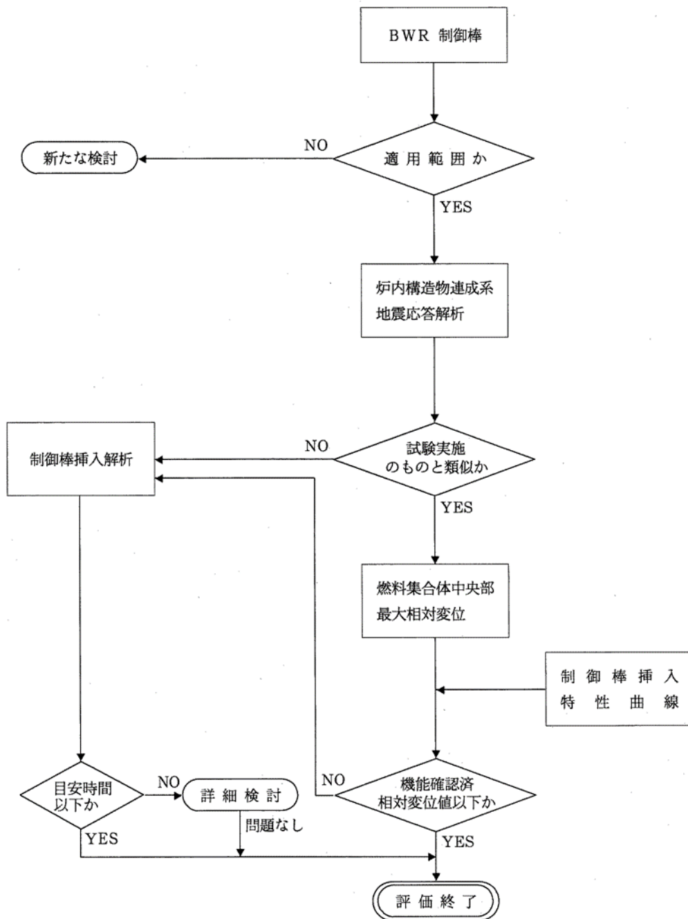
図 2-1 制御棒挿入性の評価手順 (BWR) (J E A G 4 6 0 1-1991 追補版)
