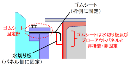
部分詳細図
