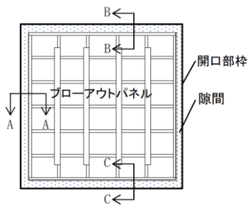
パネル見附図
