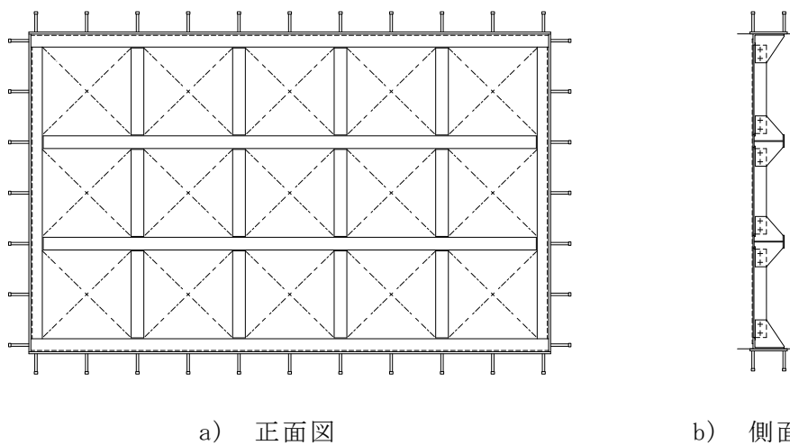
図 2-1 (1) 原子炉建物内側ブローアウトパネルの構造 (No. 4, No. 5 立面図)
