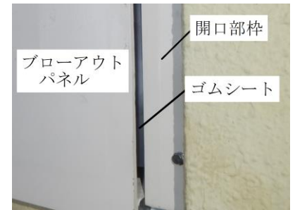
パネル据付状況 (水切り板部)
