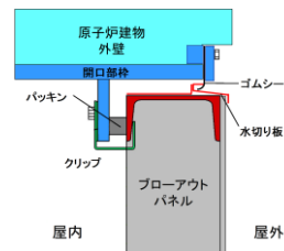
B-B 断面図
