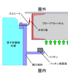
A-A 断面図 (開放時)
