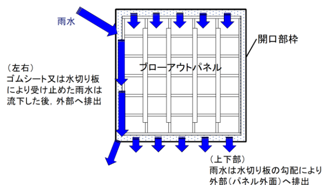
雨水排水概要 (雨水の流れ)
