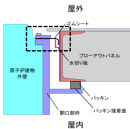
A-A 断面図
