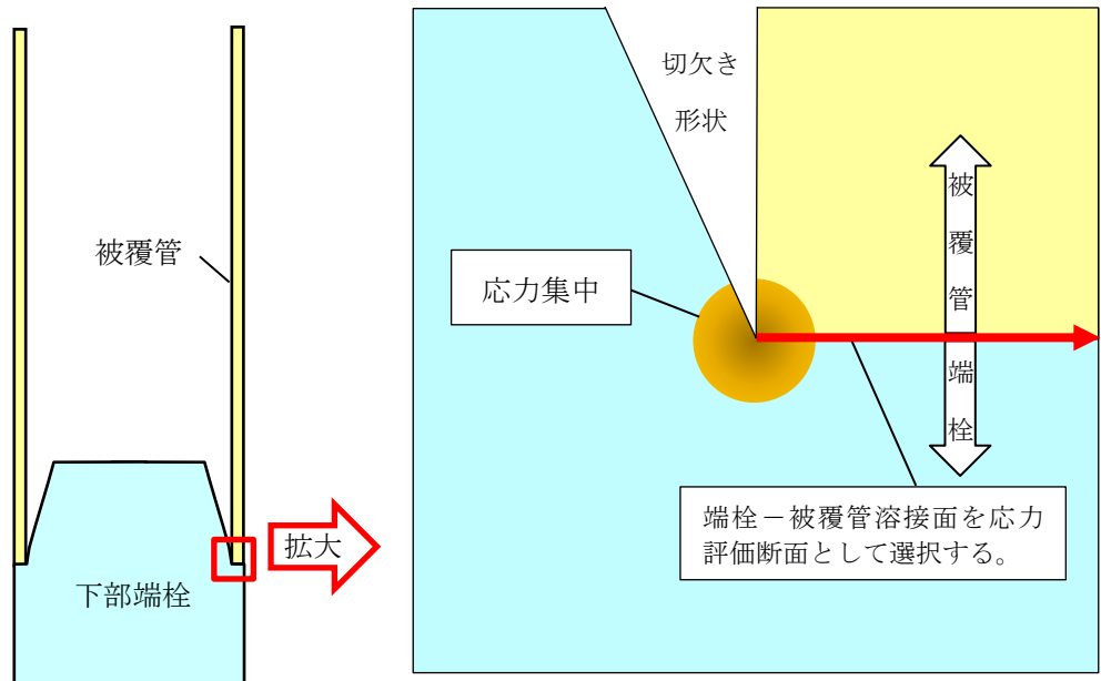
付図-1 下部端栓部の有限要素法による応力解析体系の模式図
