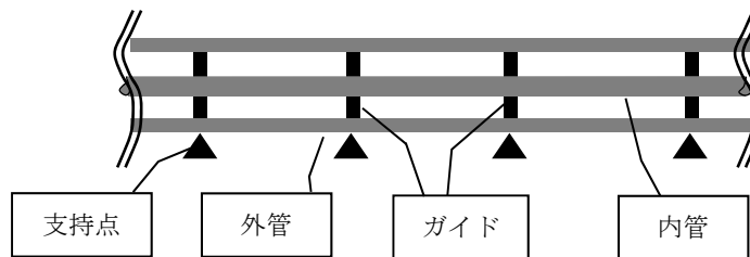
第 2-1 図 二重管の構造概要図
