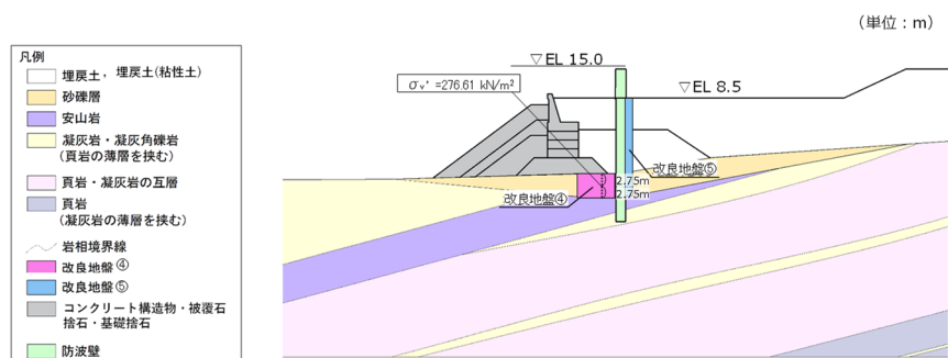
図 4.2.2-1 改良地盤④における G_{ma} 算定に用いる \sigma_v'
