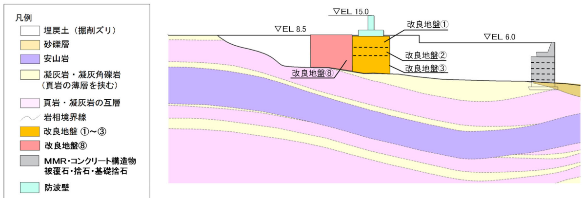
図 3-12 流動化处理土の配置図 (防波壁 (逆T擁壁)，K-K断面)
