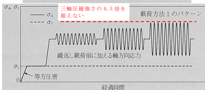
図 4.5.3-4 JGS 2563 载荷方法の模式図等(赤字で加筆)
