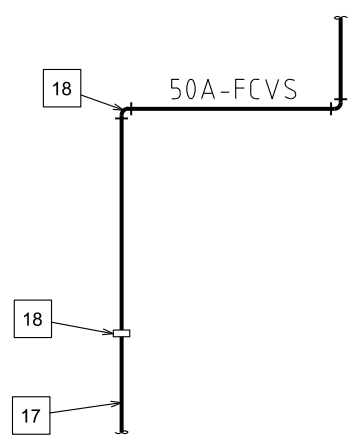
F~F矢視図
