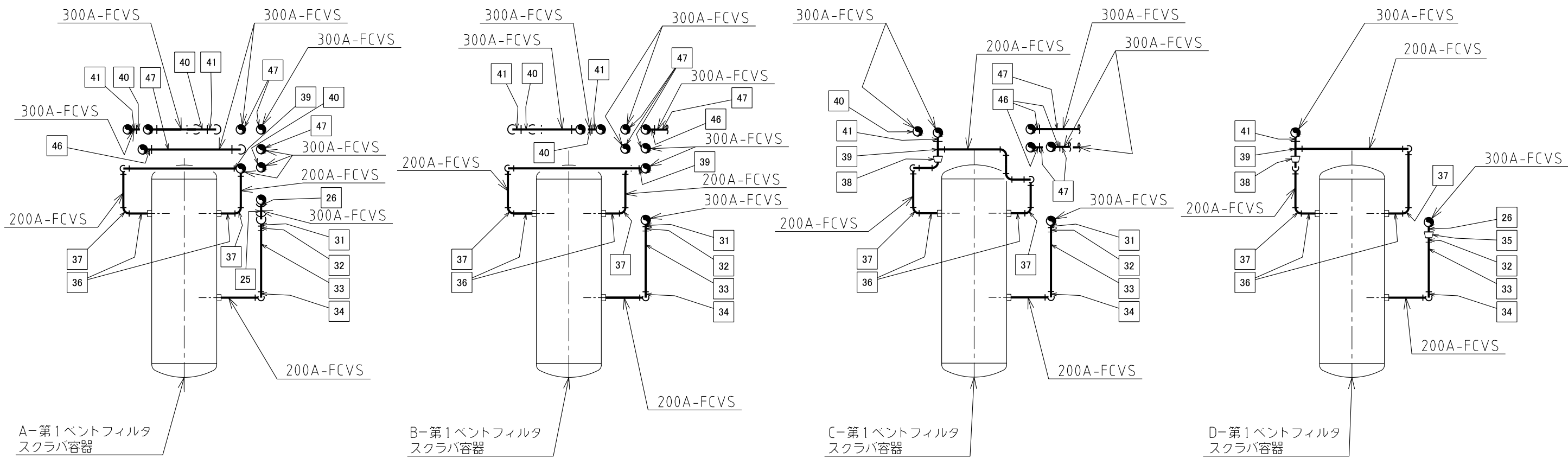
C~C矢視図
