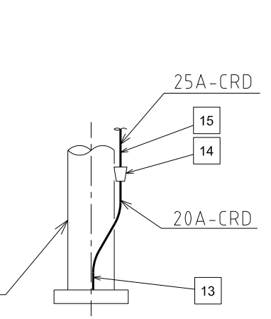
G~G矢視図 (T.Y.P.)
