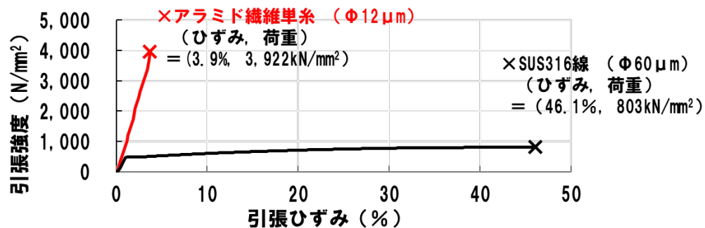
第 1 図 引張強度の比較（アラミド繊維、SUS316）
