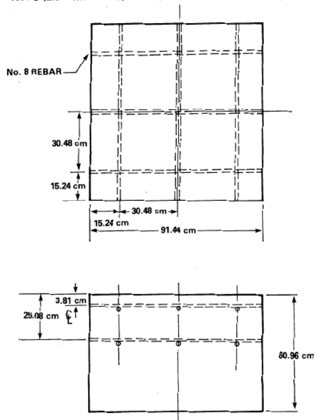
第 24 図 コンクリート試験体の概要 (LSC-1)
