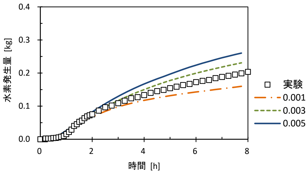
第 22 図 CONTAIN-LMRによるナトリウム-コンクリート反応実験(III-1M)の水素発生量との比較 (FRACV=0.001, 0.003, 0.005 の感度解析)
