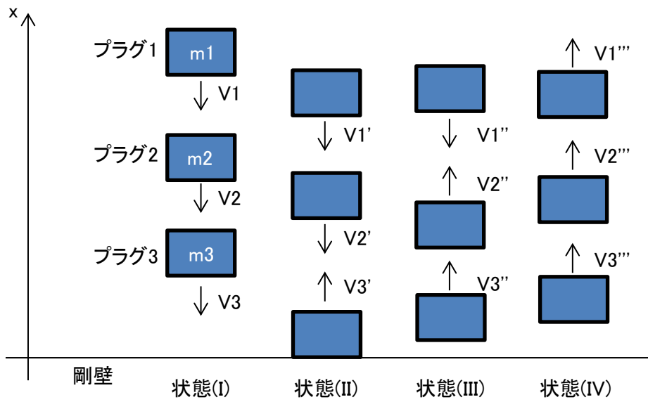
第 4. 1. 1 図 互いに独立したプラグの衝突解析のイメージ (Case-6)
