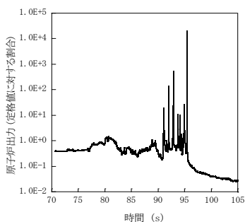
原子炉出力の推移
