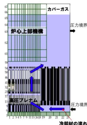
SIMMER-III r-z 2次元計算体系図
