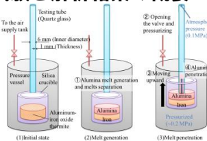
THEFIS 試験の概要
