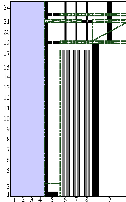
内部ダクトと燃料ピン束を2次元軸対象で表現した、炉内試験の解析体系（図外側の数字はr、z方向のセル番号、灰色は燃料ペレット、黒はステンレススティール、水色はナトリウム）
