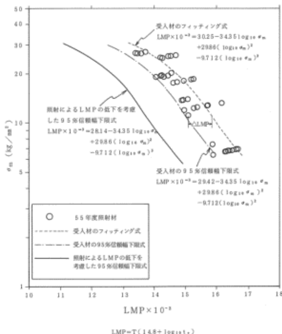
図30 昭和55年度材照射済燃料被覆管(急速加熱試験)のLMPとσ m の関係
