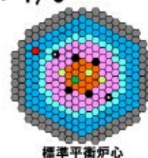
標準平衡炉心
