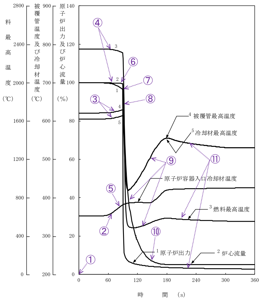
第 4. 4. 9 図 主冷却器空気流量の減少
