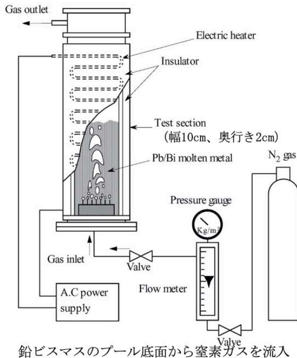
鉛ビスマスのプール底面から窒素ガスを流入 第 4.16 図 鉛ビスマス二相流動試験装置の概略図
