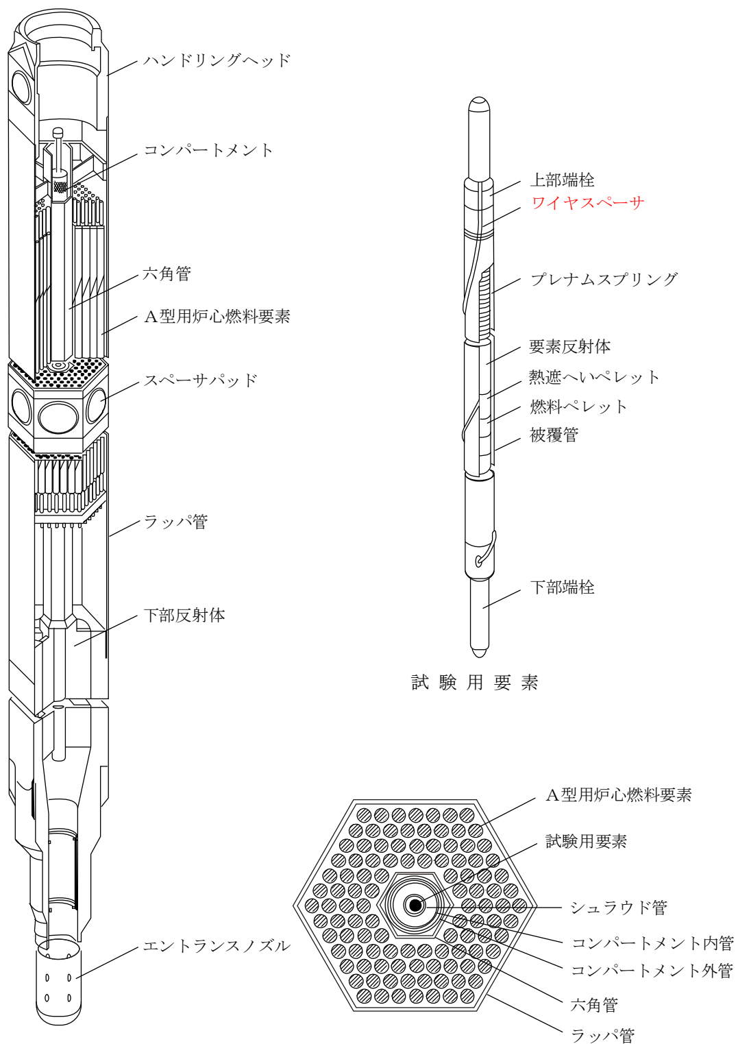
第 4.1.2 図 A型照射燃料集合体—限界照射試験用 (参考用)
