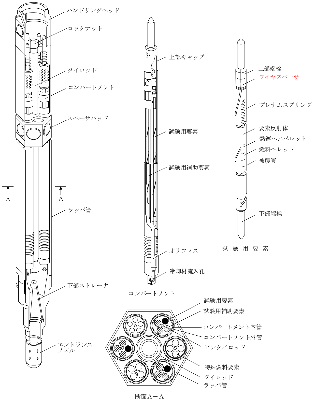
第 4.1.3 図 B型照射燃料集合体—限界照射試験用 (参考用)
