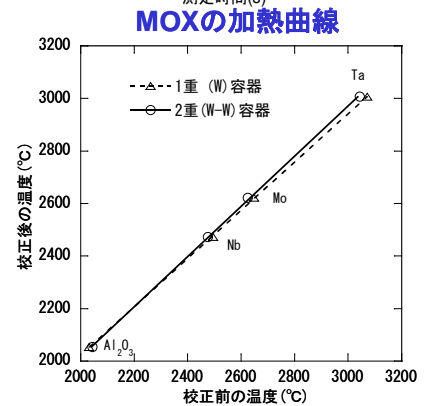
標準試料による温度校正
