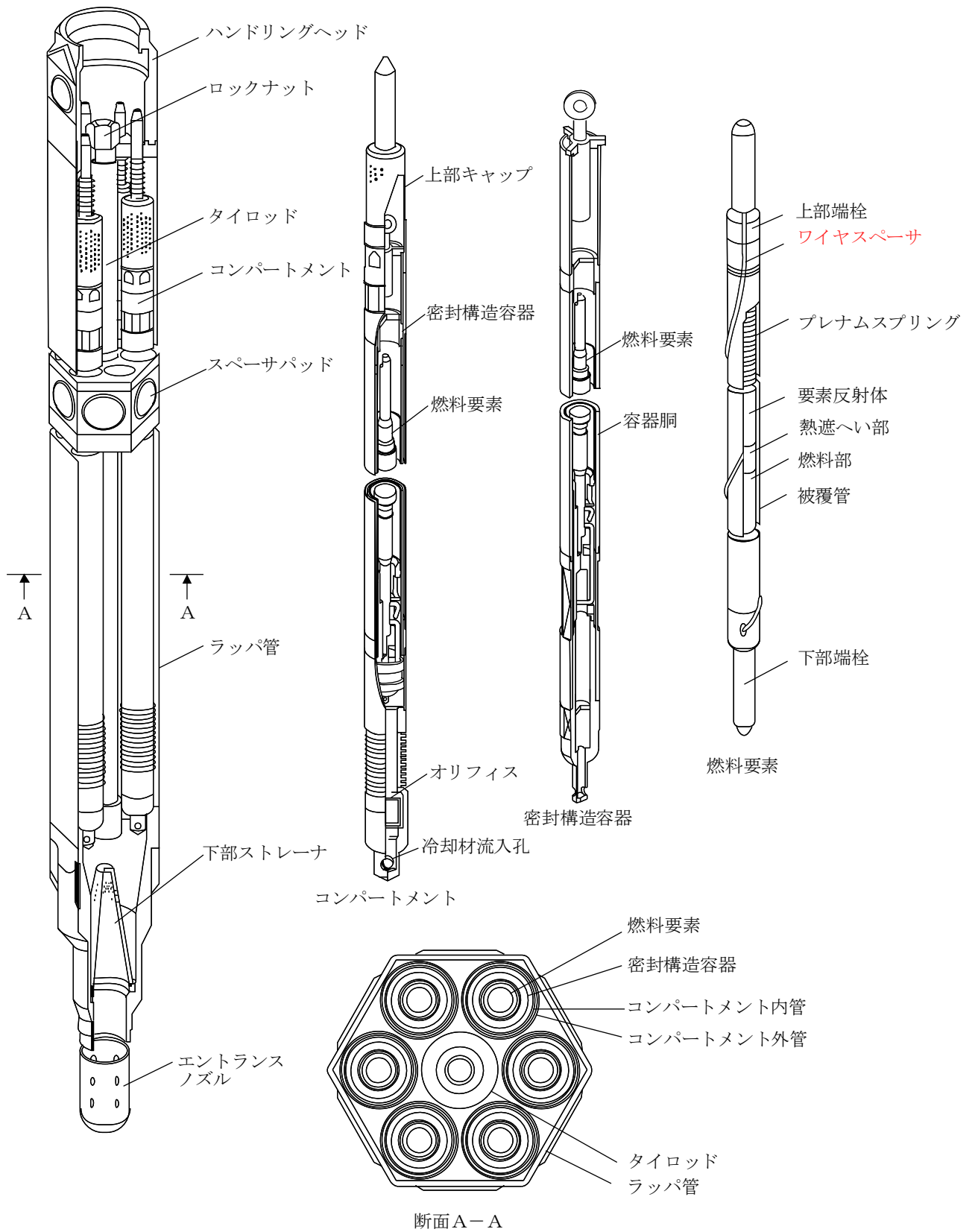
第 4.1.5 図 B型照射燃料集合体—基礎試験用 (参考用)
