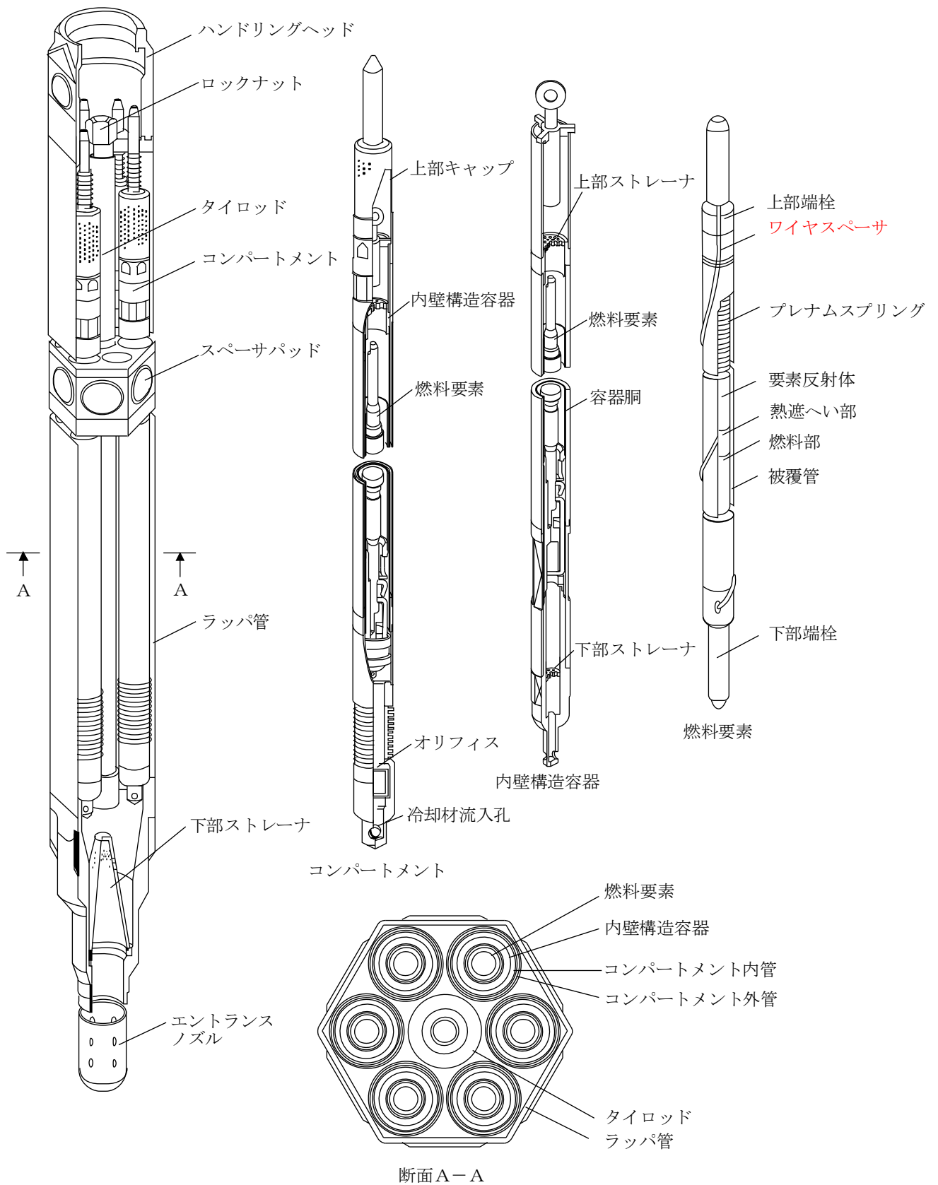
第 4. 1. 4 図 B 型照射燃料集合体—先行試験用 (参考用)
