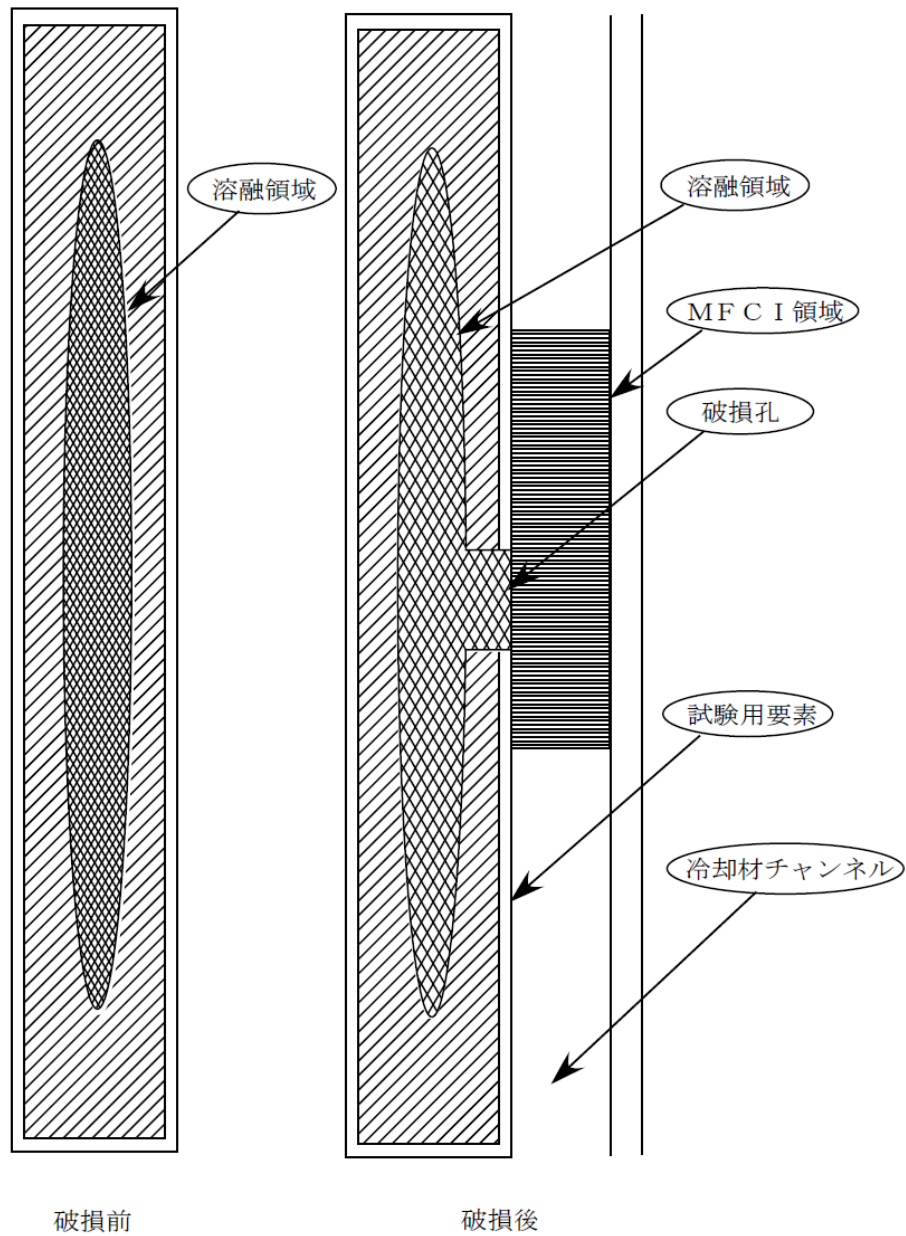
第1図 熔融燃料放出によるMFC Iの発生
