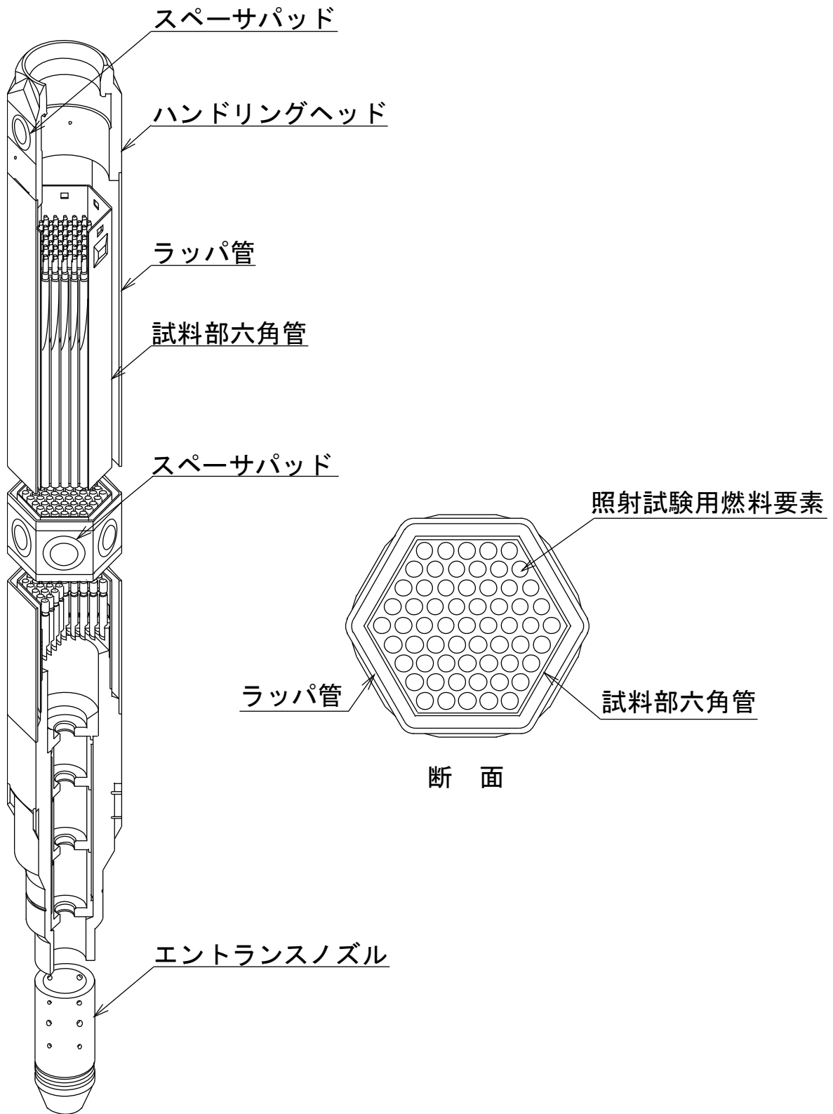
第 4.1.6 図 C型照射燃料集合体 (参考用)
