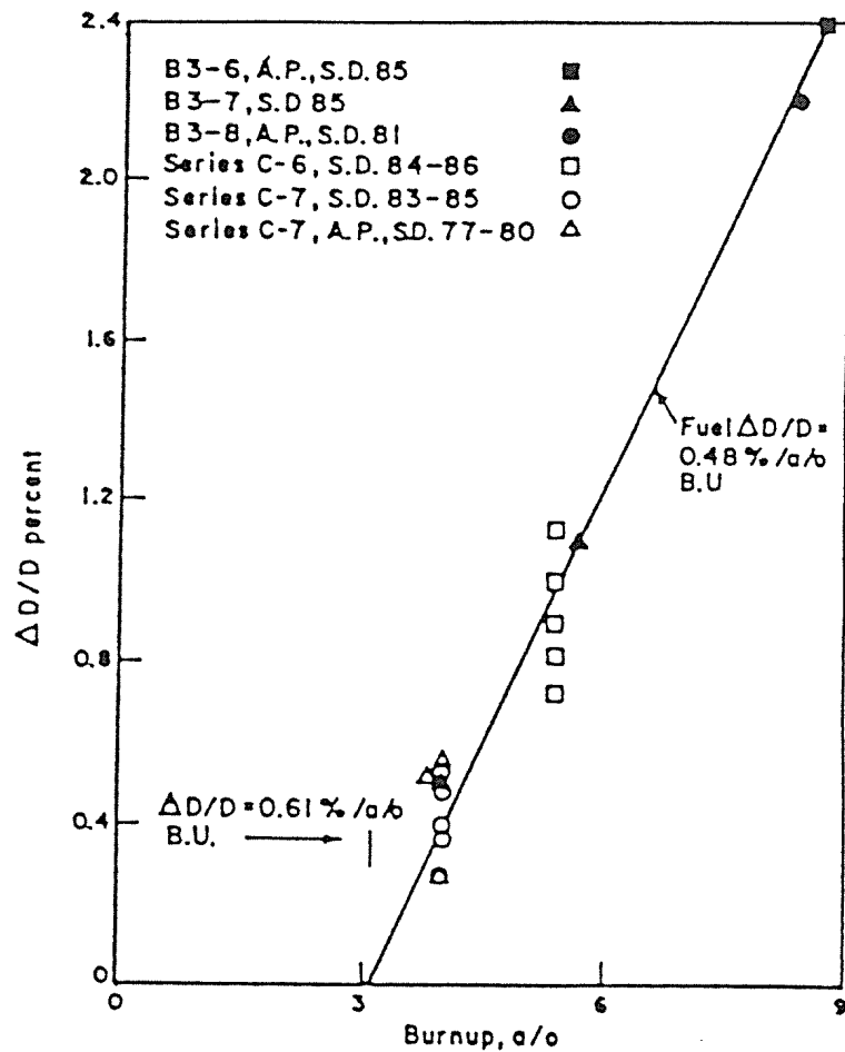
第 2.5.1 図 窒化物燃料の被覆管歪
