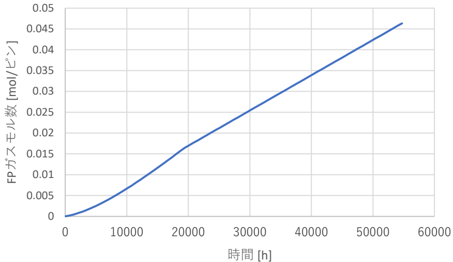
第 3.1 図 FP ガス発生量の計算結果
