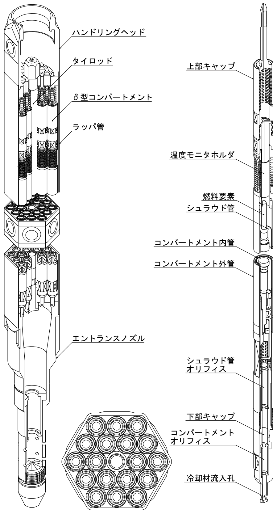
第 4.1.8 図 D型照射燃料集合体－ \delta 型コンパートメント最大装填型 (参考用)
