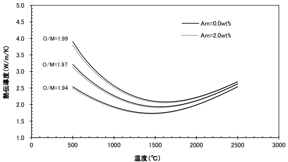
第1図 MOX燃料熱伝導度の温度依存性 (ペレット密度94%TD)
