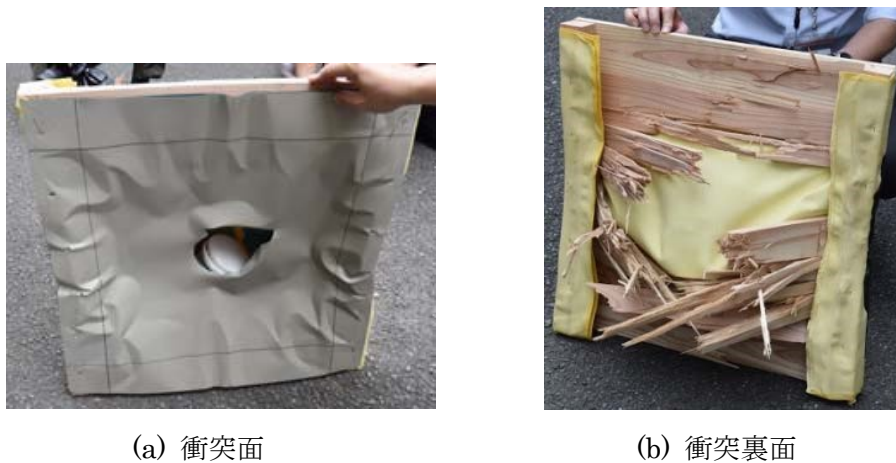
第3図 試験後の退避壕補強屋根 (写真)
