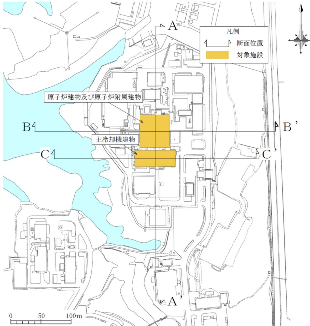
評価対象断面
