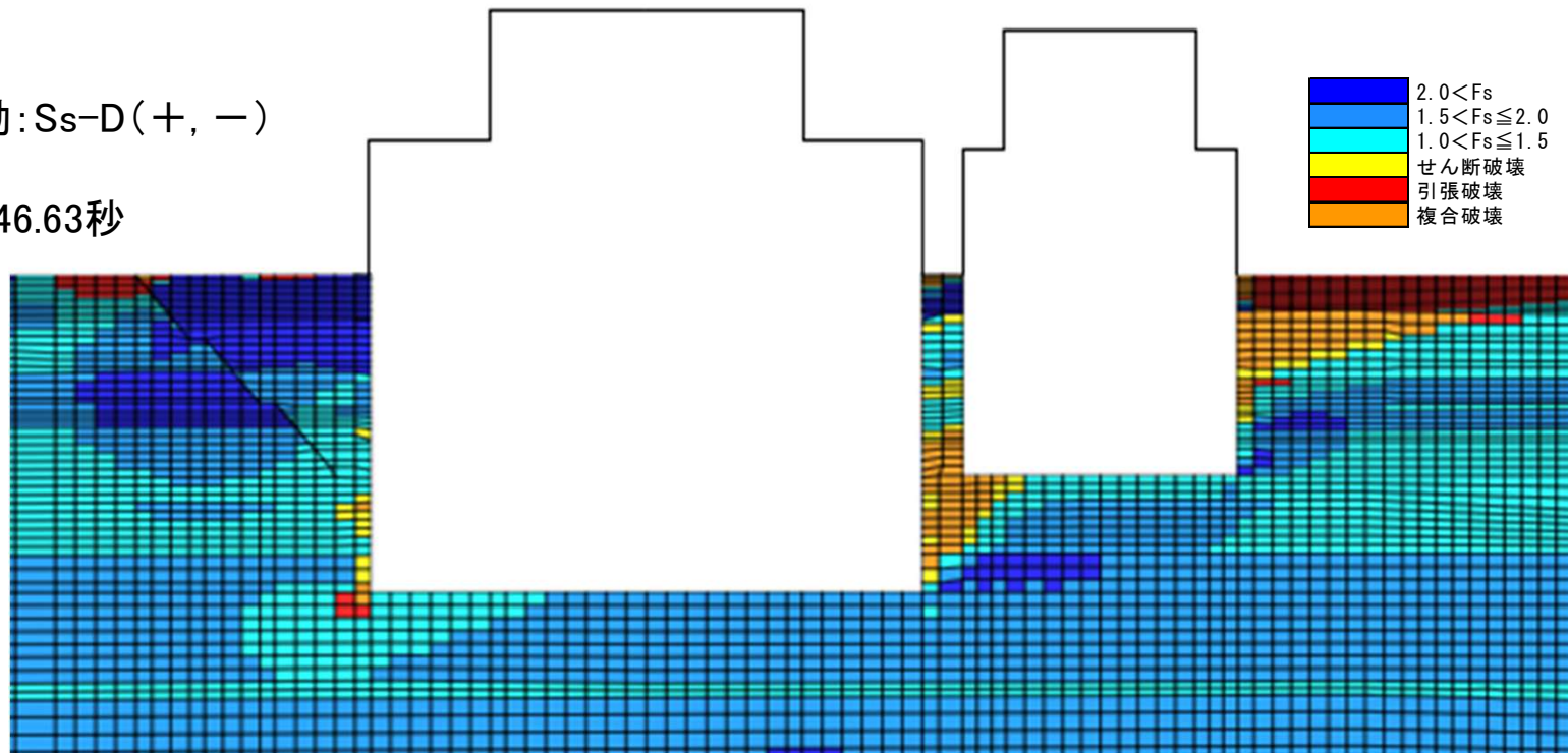
局所安全率
