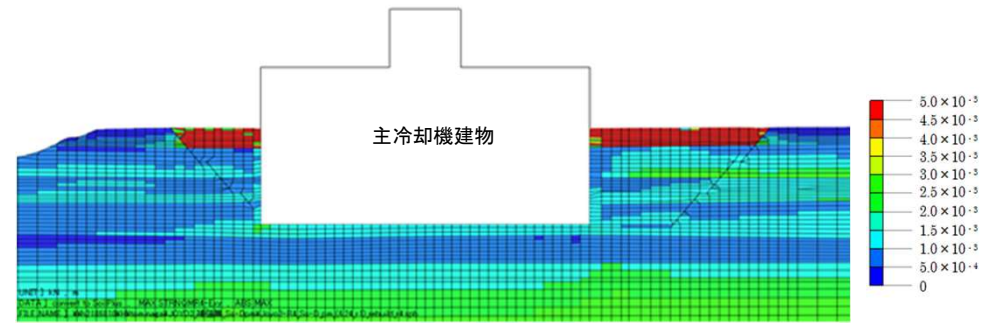
最大せん断ひずみ(-)
