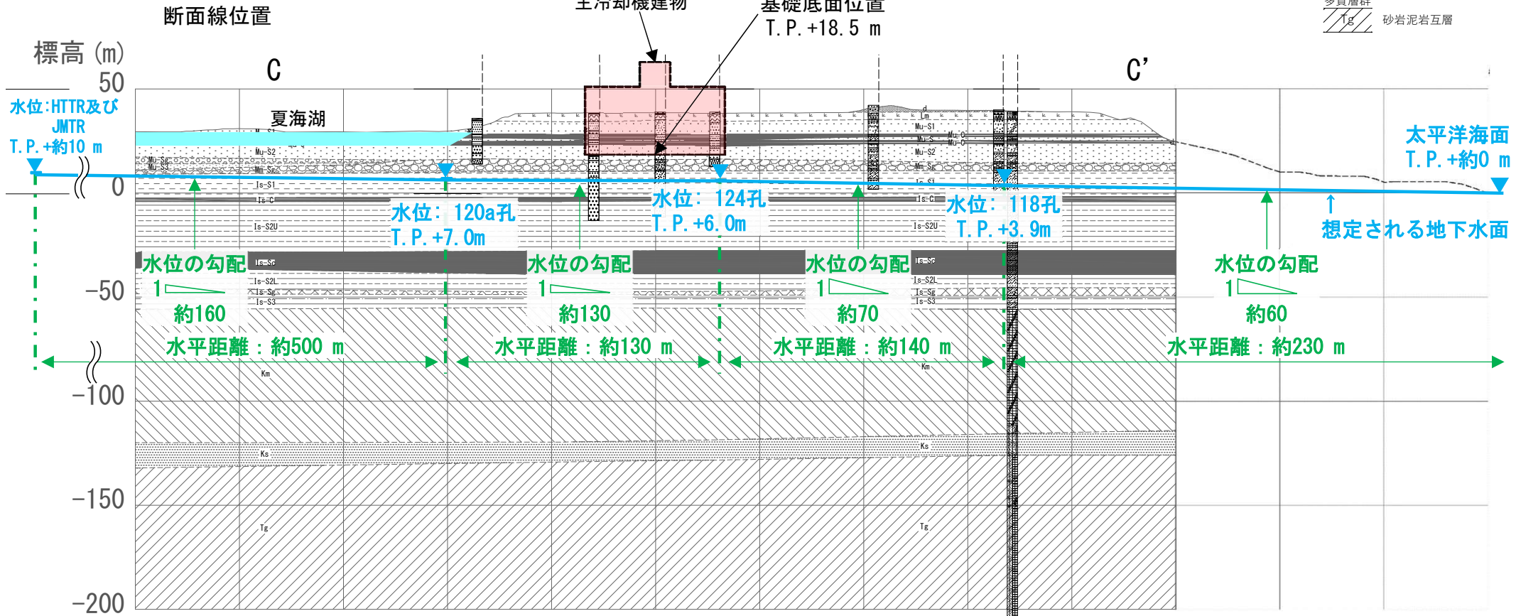
C-C' 断面(東西方向)
