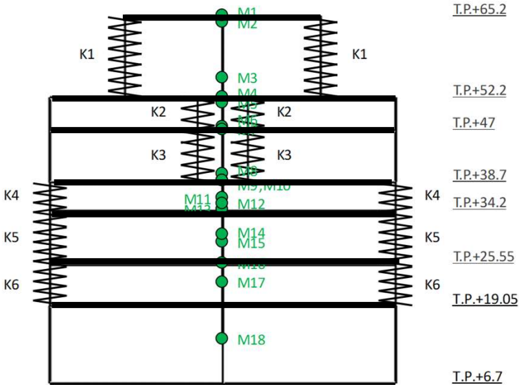
有限要素モデル
