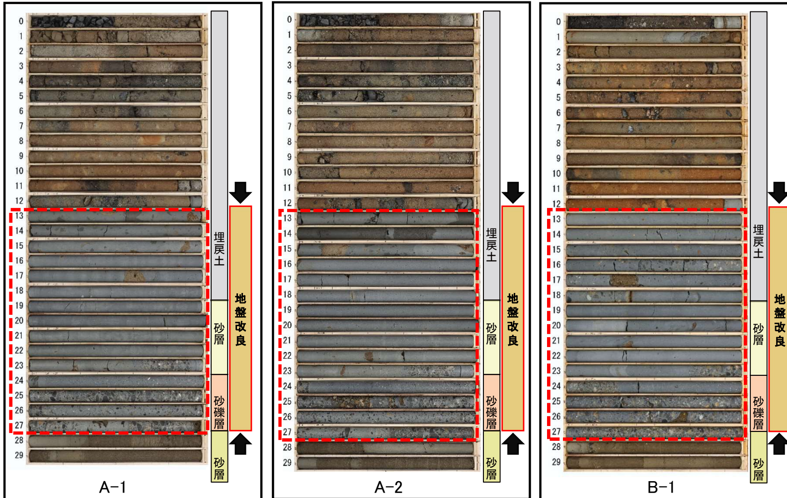
地盤改良範囲
