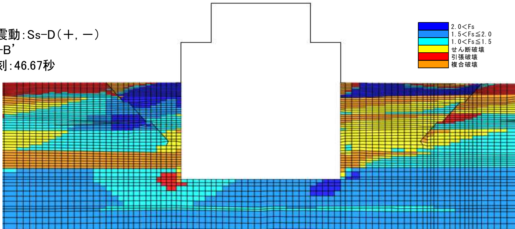
局所安全率
