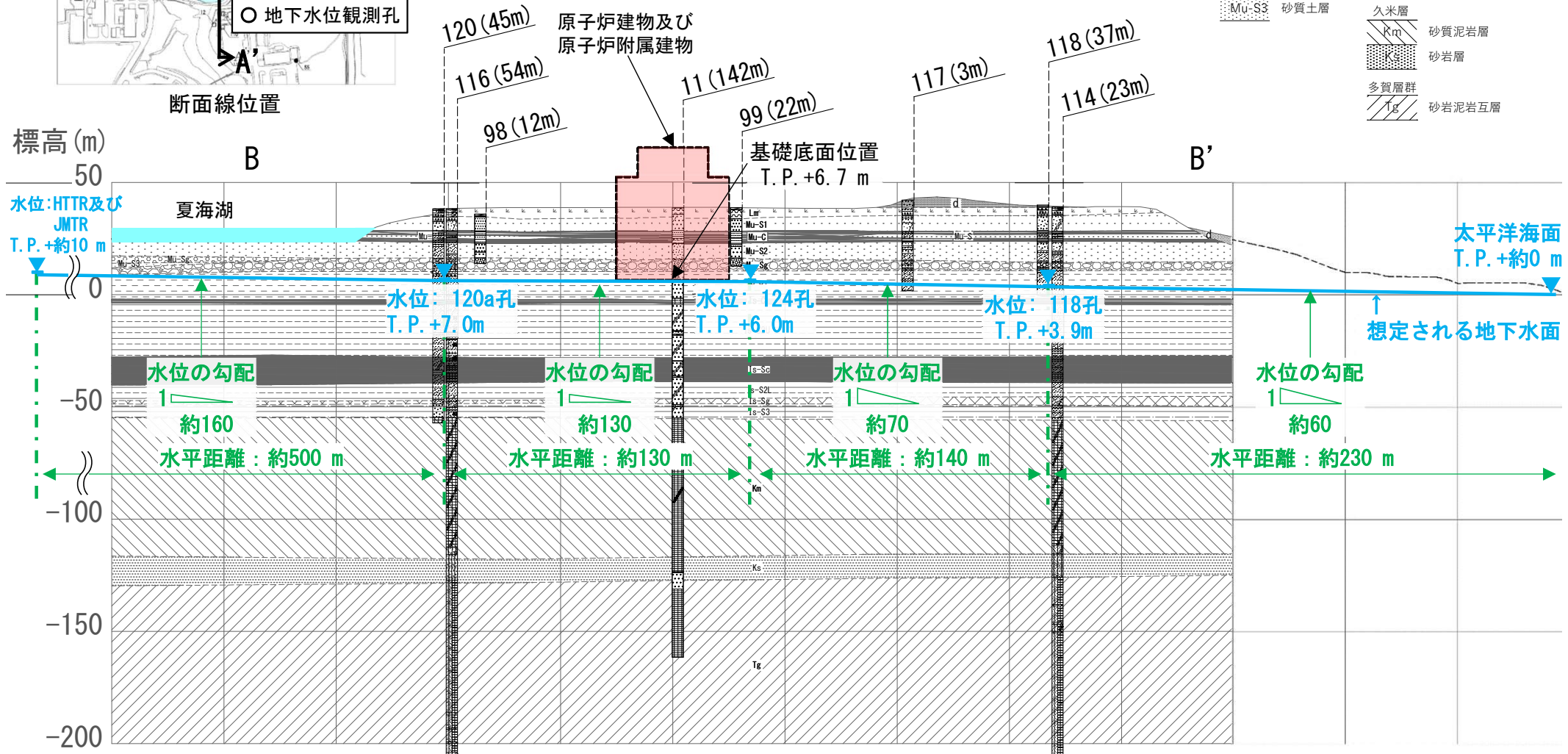
B-B' 断面(東西方向)
