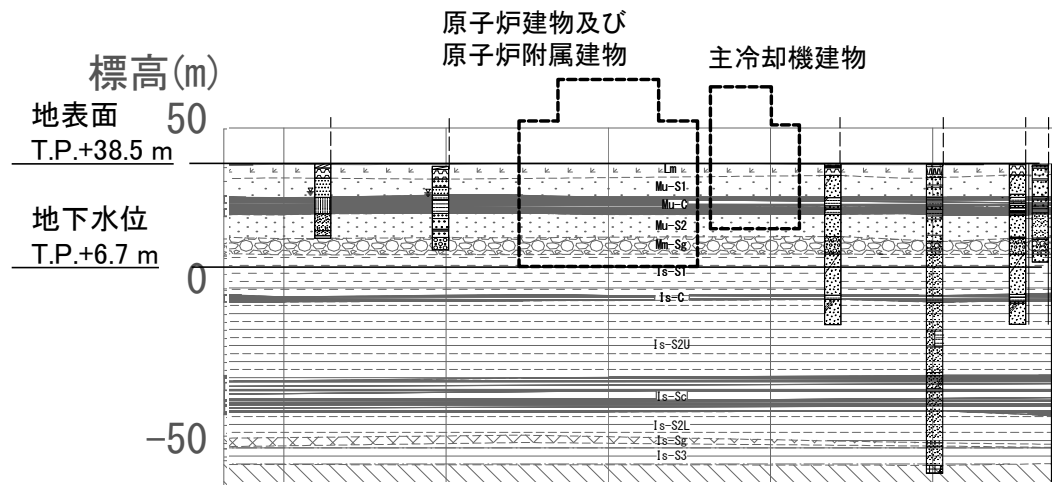
評価対象施設の周辺断面(A-A' 断面)
