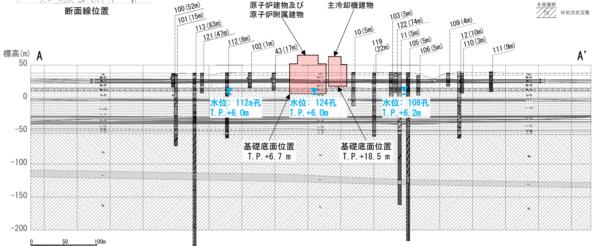
A-A' 断面(南北方向)
