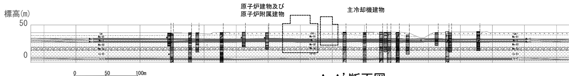
A-A' 断面図
