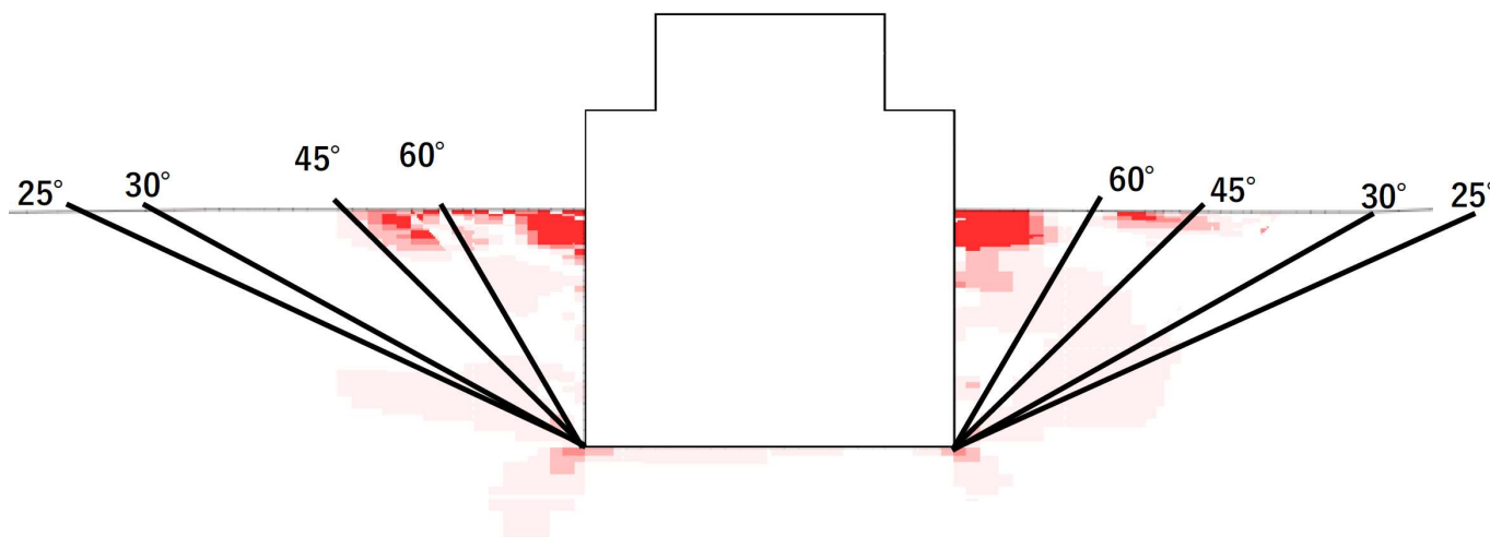
せん断応力比分布
