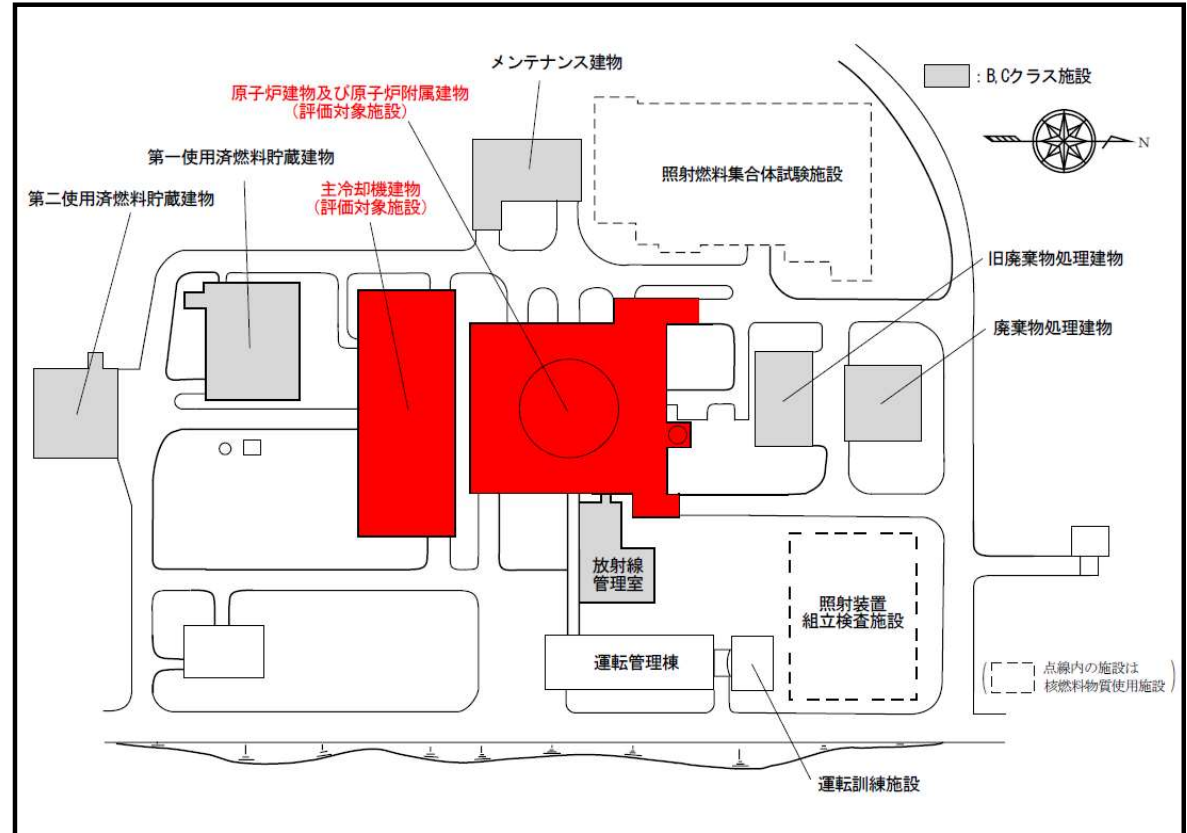
評価対象施設配置図
