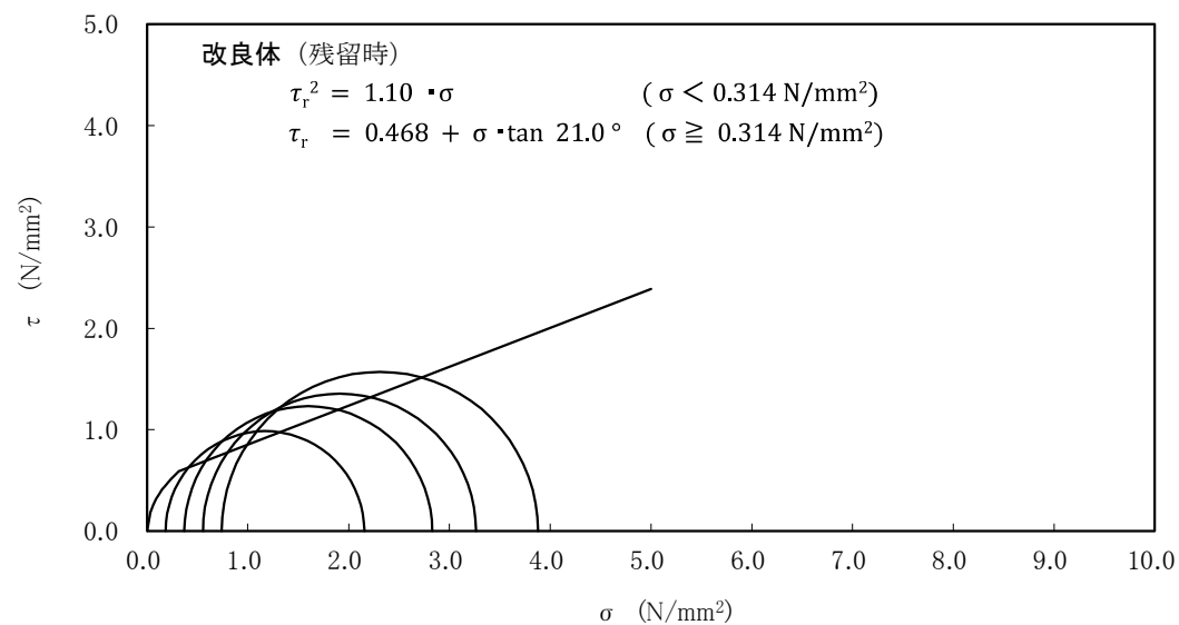
強度特性(改良地盤)
