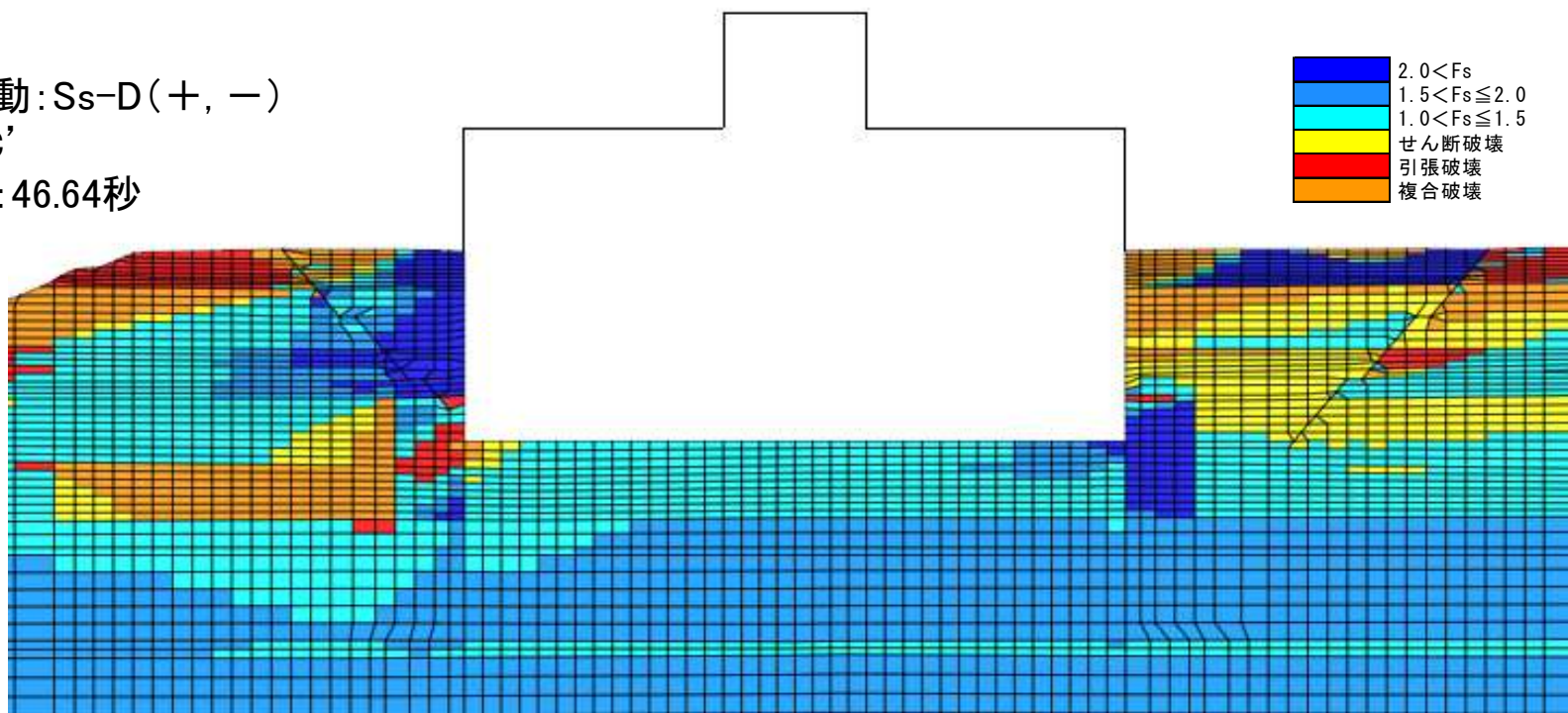
局所安全率
