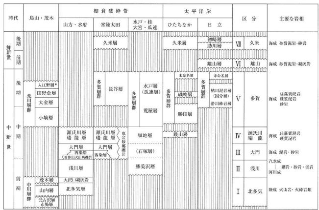
*入江野層は、本図幅地域内に分布しない。 第2図 水戸図幅地域内の新第三系の対比
