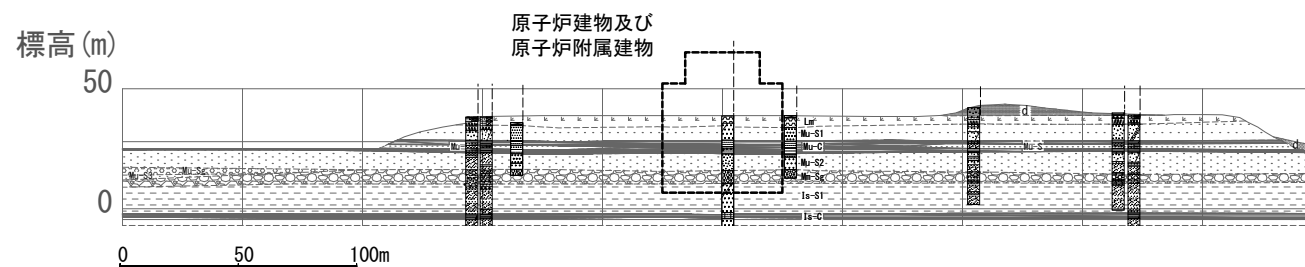
B-B' 断面図
