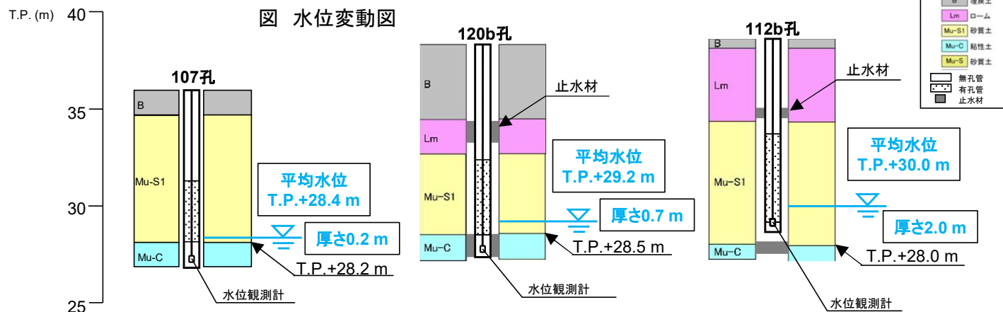
図 宙水観測孔構造図
