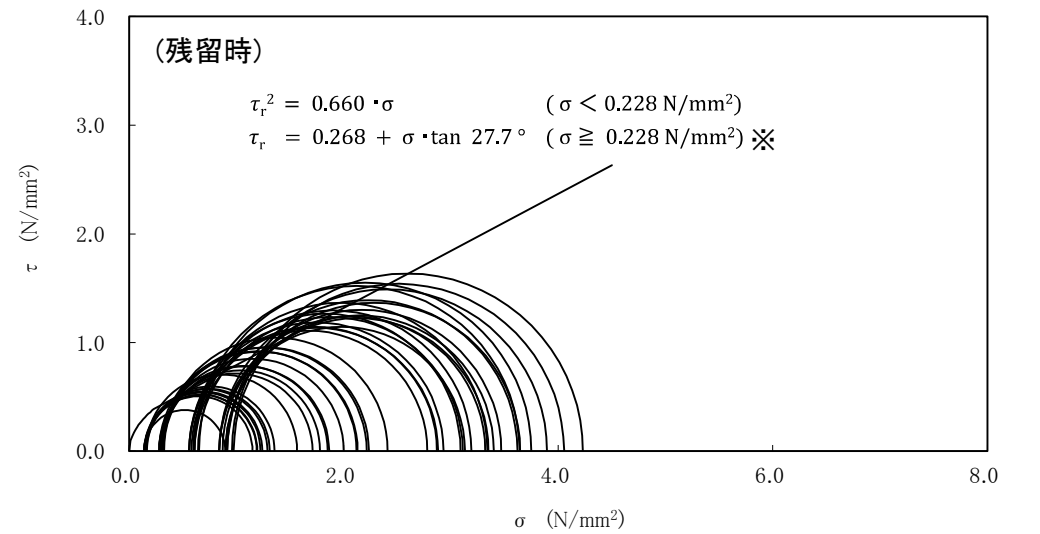
強度特性(Is-S 1 )
