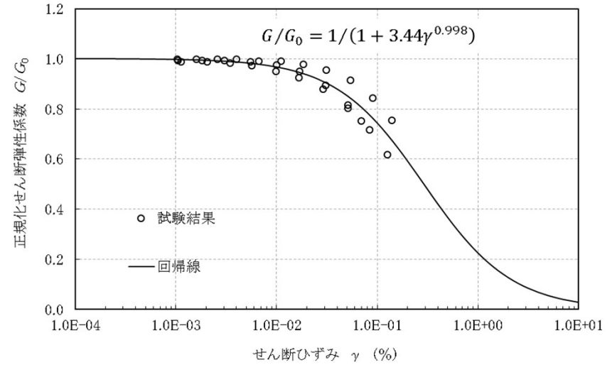
(a) 正規化せん断弾性係数 G/G_0
