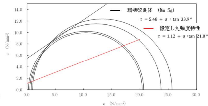
現地改良体 Mm-Sg (砂礫層)
