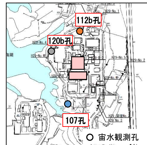
図 宙水観測孔位置
