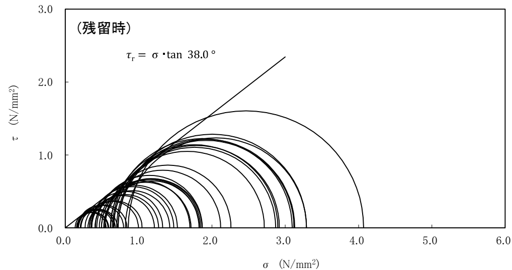
強度特性(Mu-S 2 )
